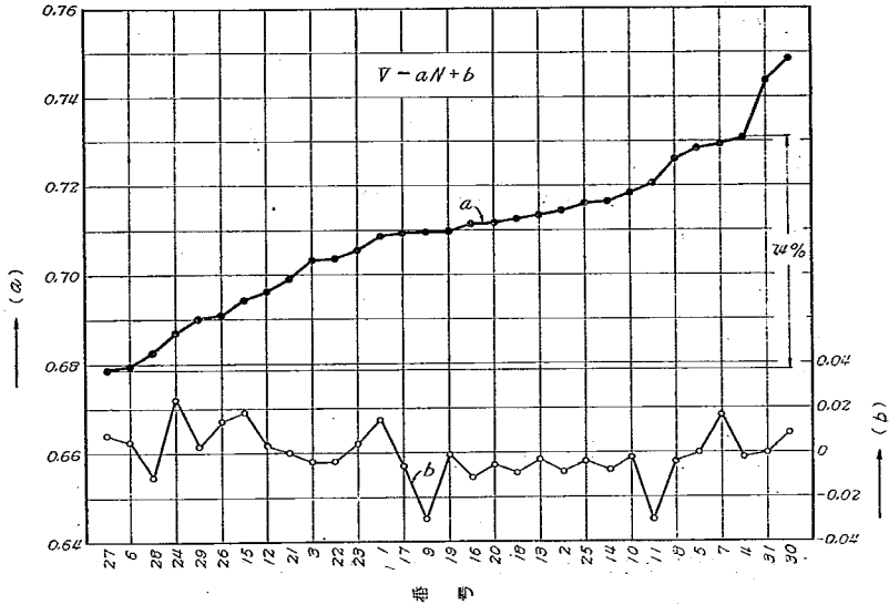
図二 外国製ブライス式流速計係数表, ←は普通ガーレー製の流速計に附した係數表より算定した a 及 b の値, (表-2 参照)
