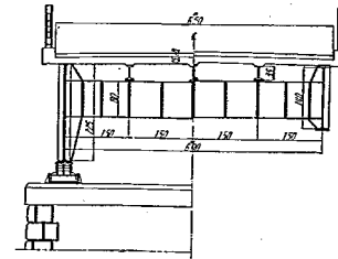
鶴川橋 一般圖 縮尺由
