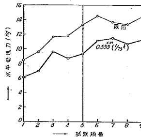
圖-5 試験順序と水平抵抗力との関係
