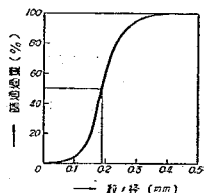
図-2 砂篩分試験の結果
