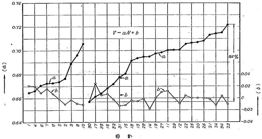
図二 外国製ブライス式流速計係数表, ←は普通ガーレー製の流速計に附した係數表より算定した a 及 b の値, (表-2 参照)
