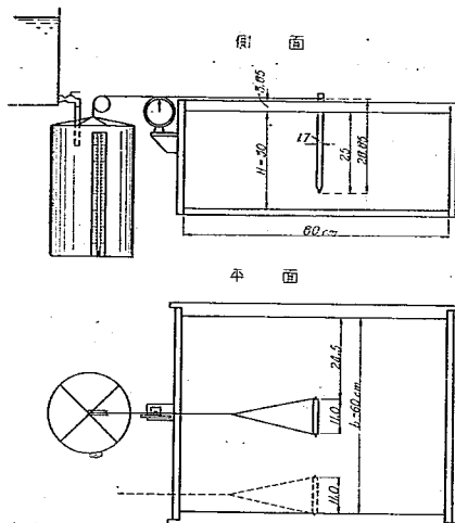
図-1 小型試験装置
