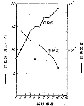
圖-7 試験順序と打止り迄の打撃回数
