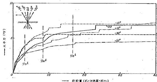
図-3 力(kg)と杭の地表面に於ける移動量(mm)との関係
