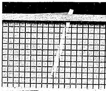
写真—3 \theta = +15^\circ 試験前
