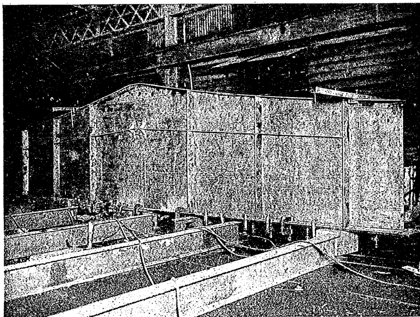
圖-30 上突縁板の假着を終り、厚板を多数の緊付具を用ひ緊結し、本焊接に着手せんとする状況。
