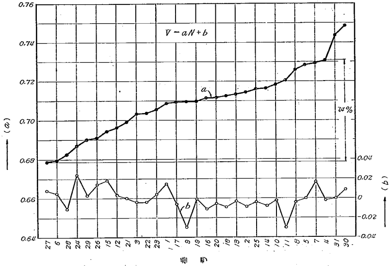
図二 外国製ブライス式流速計係数表, ←は普通ガーレー製の流速計に附した 係数表より算定した a 及 b の値, (表-2 参照)
