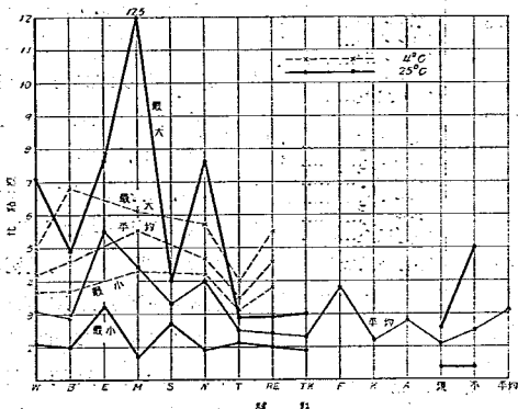
圖 — 7. 4°/25°C 比粘度の比
