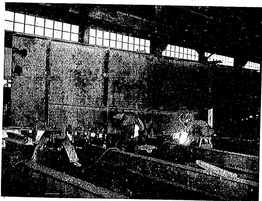
圖-28 緊結具に依る下突縁板の取付
