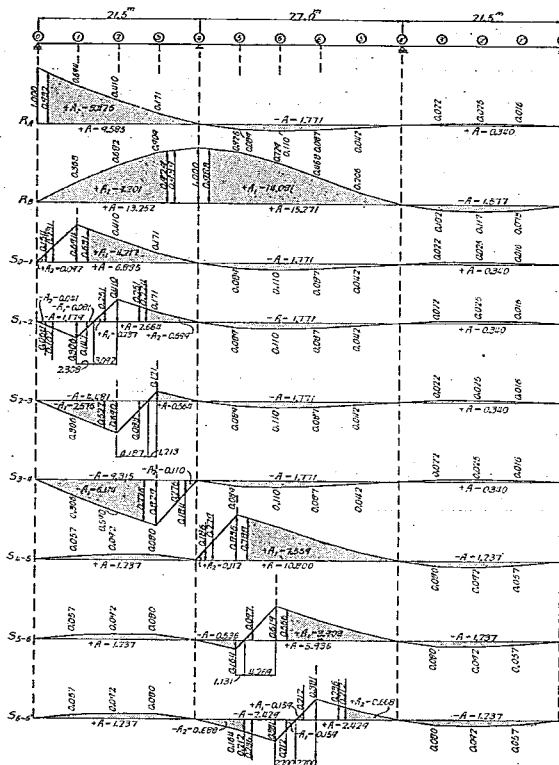
圖-10 反力及び剪斷力影響線
