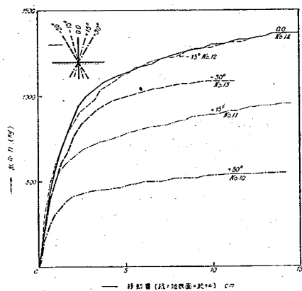
図-10 力と移動量との関係 (米松杭の場合)
