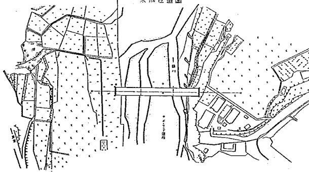
築橋位置圖
