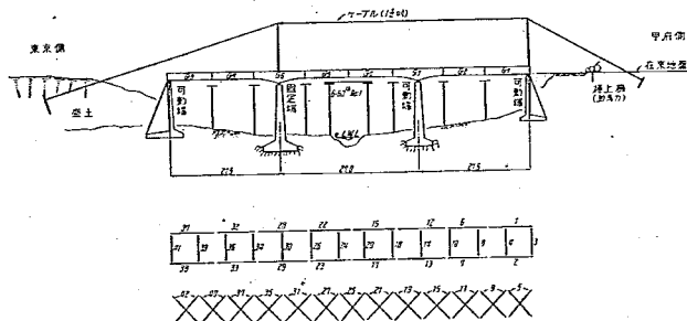
圖—38 下突縁取付
