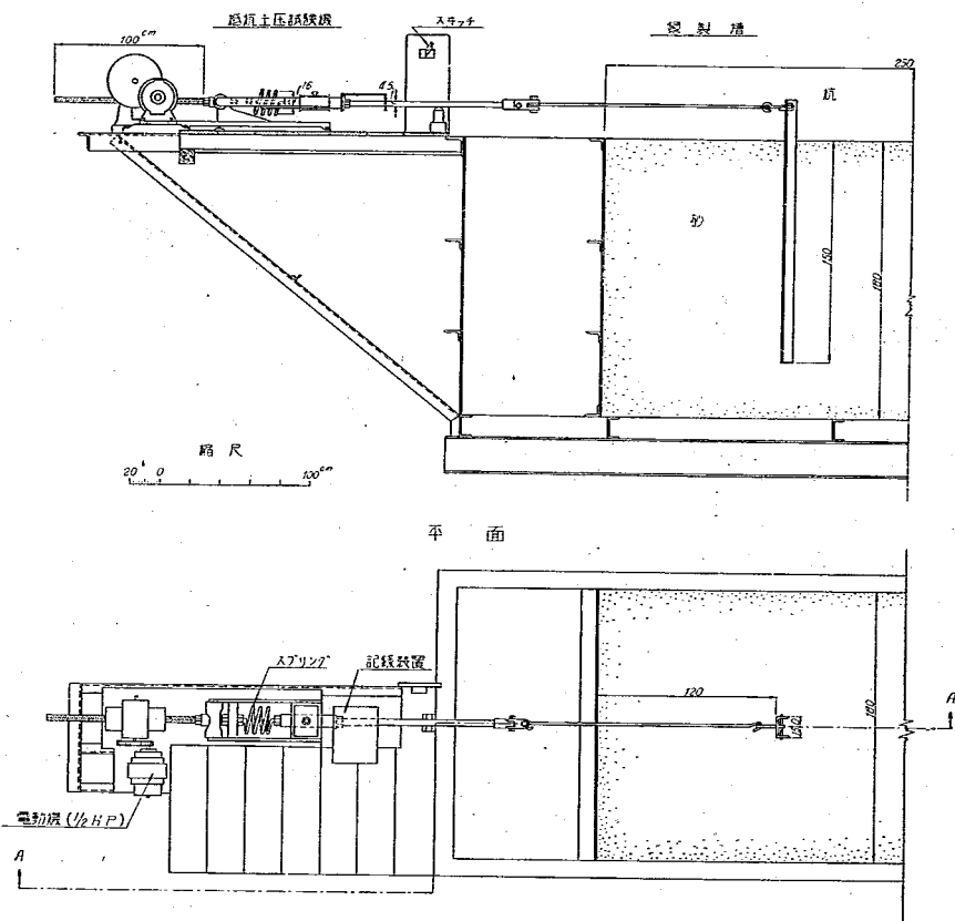
圖-8 大型試験装置
