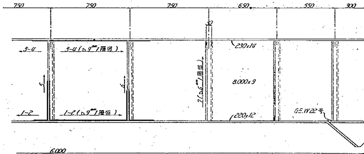
圖-25 歪の状態
