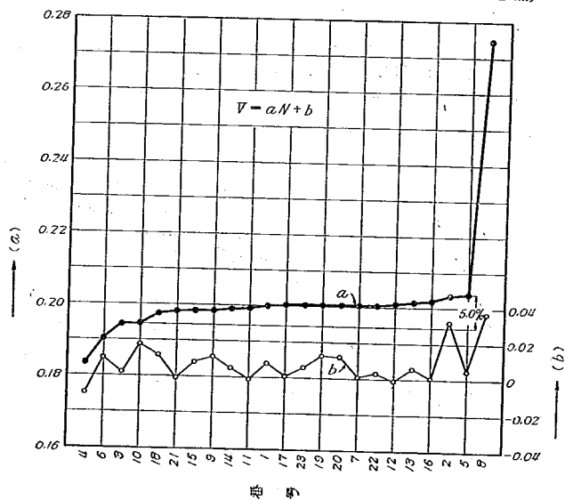
圖一4 森式流速計係數表，すべて桿にて支へて検定したもの。(表-5 参照)
