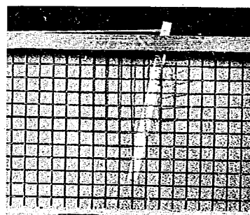
写真—4 同左 試験後 d = 1.1 cm
