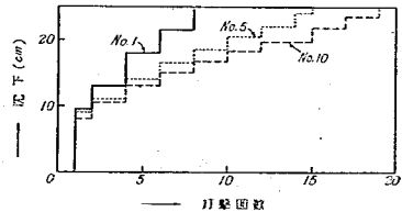
圖-7 試験順番と打止り迄の打撃回數
