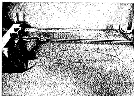
写真—11 大型試験 溝形鋼杭（杭の長さ1.8 m）に 依るもの \theta = +15^\circ 試験後の地表面の状 態、地表面の杭の動き d=11.85 cmの時
