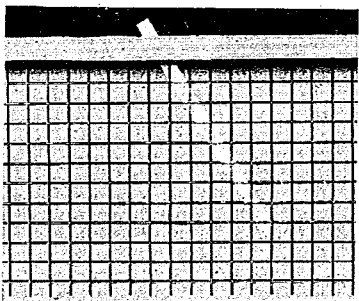
写真—9 \theta = -30^\circ 試 験 前
