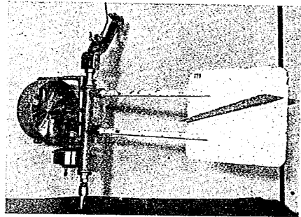
寫眞—4 森式流速計
