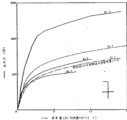
図-9 鉛直杭の水平抵抗力と移動量との関係
