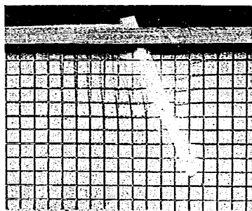
写真—8 同左 試験中 ( d=0 \sim 1.5 cmの間露出)
