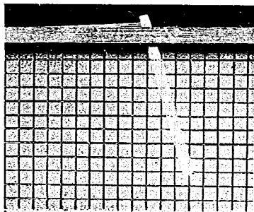
写真—7 \theta = -15^\circ 試 験 前
