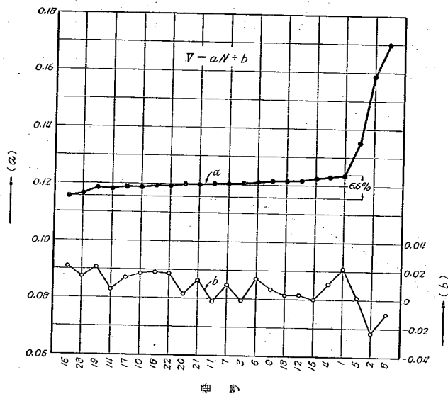
圖一4 森式流速計係數表，すべて桿にて支へて検定したもの。(表-5 参照)
