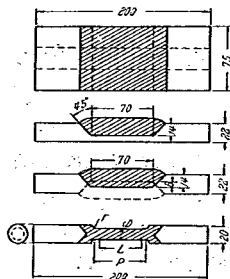
附錄圖—1 引 張 試 験 片 標點距離 L=50 \text{ mm} 平行部長 P=60 \text{ mm} 直径 D=14 \text{ mm} 圓弧の半径 V=5 \text{ mm}
