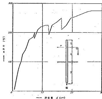
圖-13 自然地盤による結果—地中の深さを同一とし、水平力を加へる高さを變へた場合
