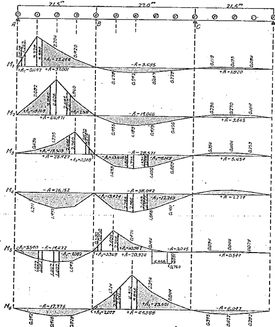
圖-9 曲 げ モー メ ン ト 影 響 線
