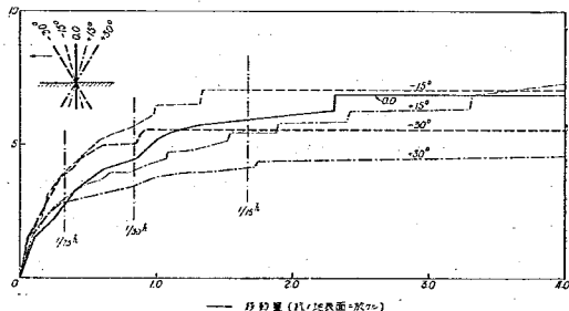
図-3 力(kg)と杭の地表面に於ける移動量(mm)との関係
