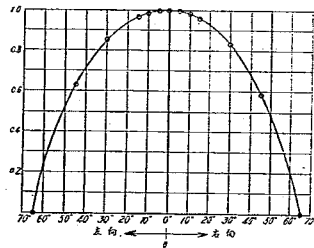
圖—6 森式流速計の軸の流向に對する偏角による係數 a の變化
