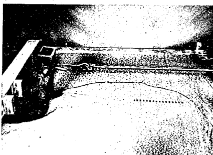
写真—12 大型試験, \theta = 0^\circ , d=13.95 cmの時
