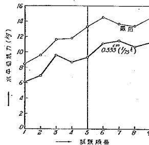
圖-5 試験順番と水平抵抗力との関係
