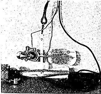
寫眞—3 廣井式流速計
