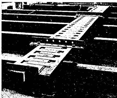
圖—35 高欄
