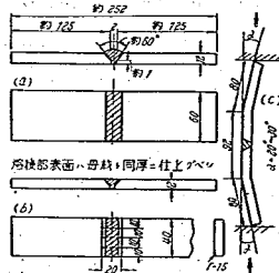
附錄圖—2 曲 げ 試 験 片
