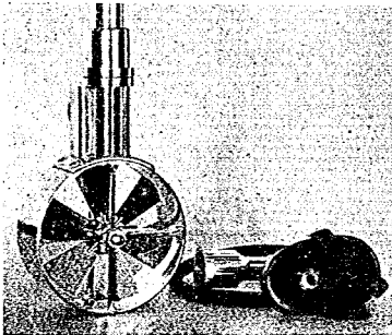
寫眞—3 廣井式流速計
