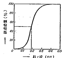
図-2 砂篩分試験の結果
