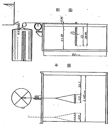
図-1 小型試験装置
