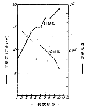
圖-7 試験順番と打止り迄の打撃回數
