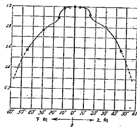
圖—6 森式流速計の軸の流向に對する偏角による係數 a の變化
