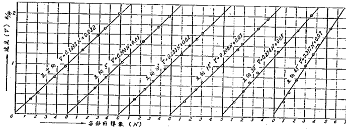
圖—5 森式流速計の軸が流向に對し傾いた場合の同轉數の變化 ——左方向の實驗値
