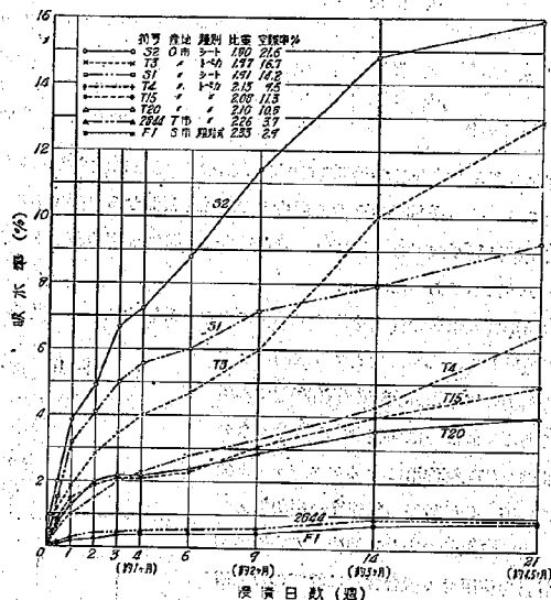
圖-15 各種舗装切取試驗材の吸水試験
