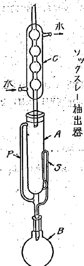
圖-15 ソックスレー抽出器
