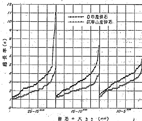
圖—1 碎石粒子の細長率
