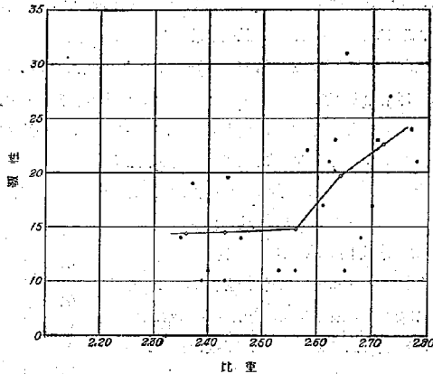
圖-3 礫石安山岩の靱性と比重との關係
