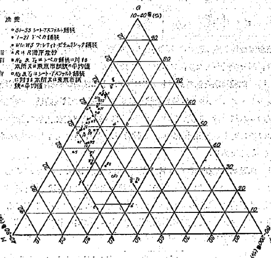
圖-6 シートアスファルト、トベカ及びワレレー イト・ビチュリシク舗装の細骨材部分の粒度三角圖
