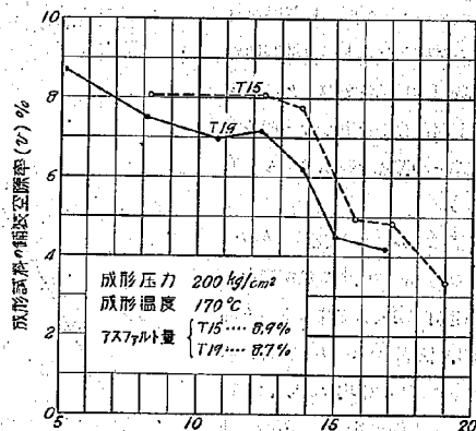
圖一11 トベカ舗装混合物の舗装空隙率と填充材部分含有量との關係
