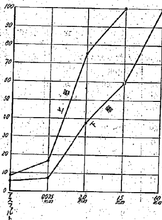
圖-13 表層及び基層の配合平均値
