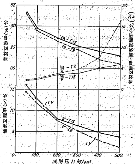
圖-8 トベカ舗装混合物成形壓力と舗装空隙率及び骨材空隙率との關係
