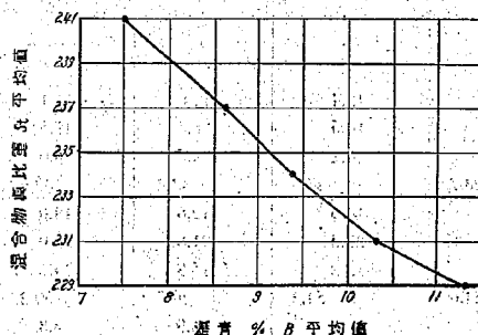
圖-1 真比重と瀝青量との關係
