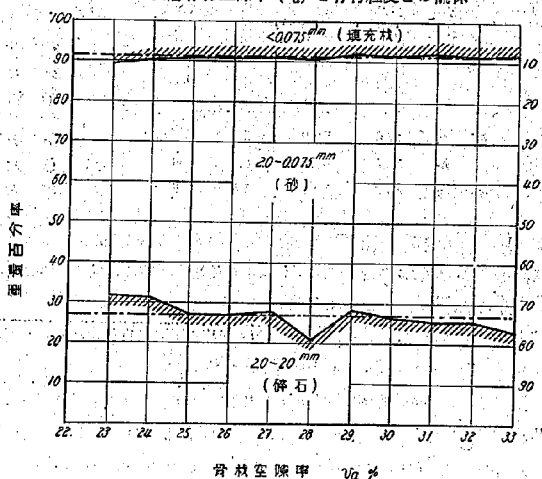
圖—5 表層骨材空隙率( v_a )と骨材粒度との關係
