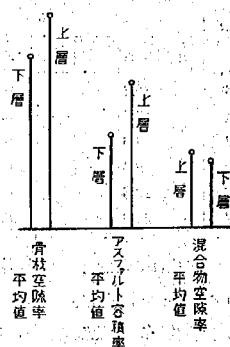
圖-10 アスファルト容積率, 骨材空隙率, 混合物空隙率等に就て表層と基層との比較
