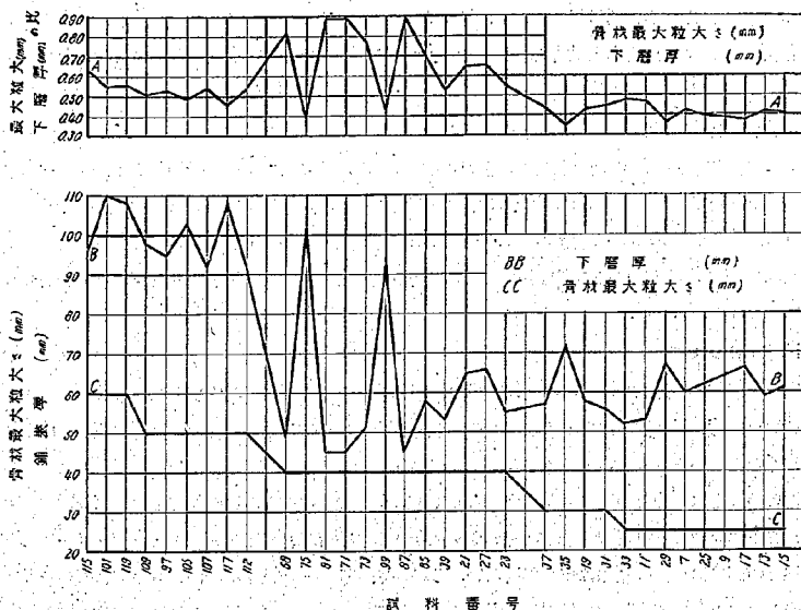
圖—12 基層骨材最大粒の大きさと鋪裝厚との關係
