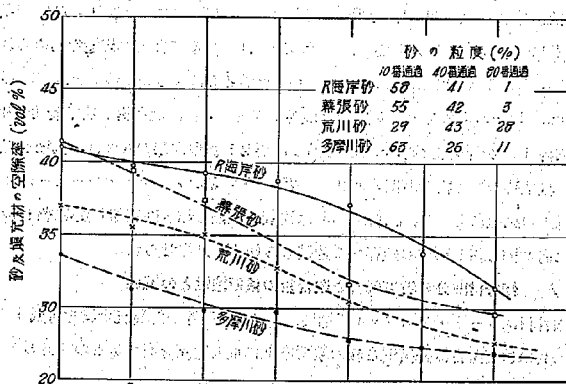
圖一10 砂の性質(粒度)と空隙率の關係 (ケロシン法)
