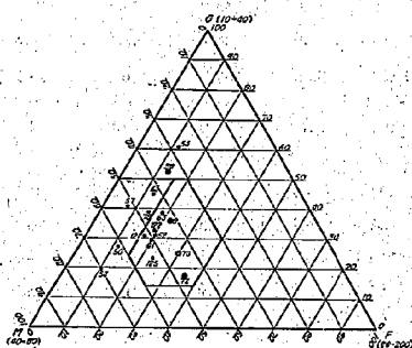
圖-6 (4) 骨材空隙率平均 v_a = 25.6\% の表層の砂の粒度
