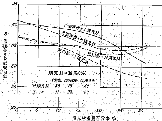
圖-12 填充材の性質と砂-填充材混合物の空隙率との關係(ケロシン法)
