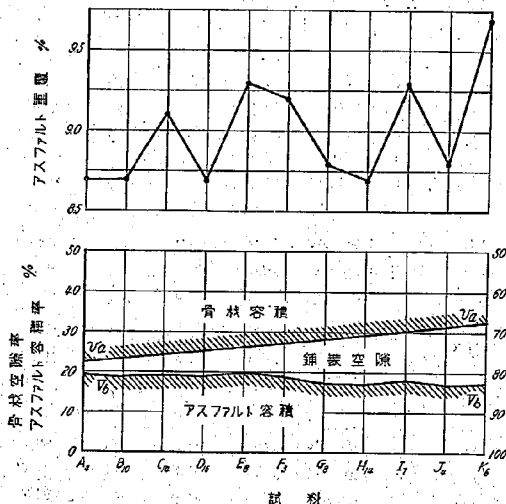
圖—4 表層骨材空隙率( v_a ) 鋪裝空隙率( v ) 骨材容積率( v_s ) 及びアスファルト容積率( V_b )の關係
