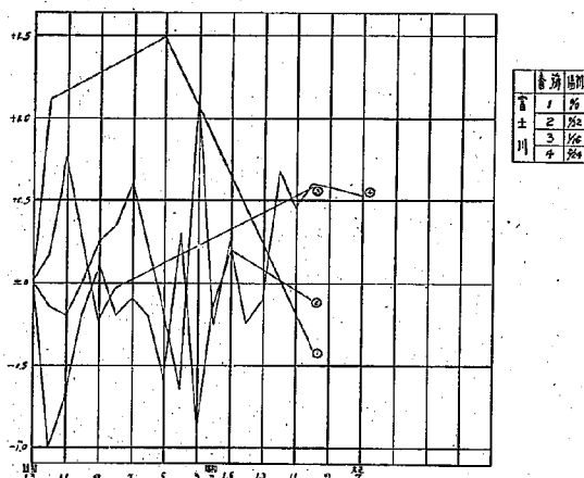
圖 — 11 富士川河床変遷圖
