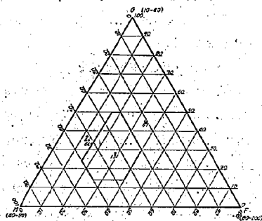
圖-6 (1) 骨材空隙率平均 v_a = 22.4\% の表層の砂の粒度
