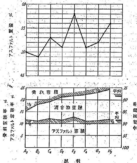
圖-9 基層骨材空隙率 ( v_a ), 混合物空隙率 ( v ) 骨材容積率 ( V_a ) 及びアスファルト容積率 ( V_b ) の關係
