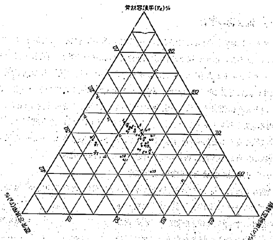
圖-7 アスファルト舗装の骨材容積率、瀝青容積率及び舗装空隙率の相互關係を示す三角圖
