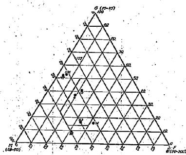
圖一6 (9) 骨材空隙率平均
