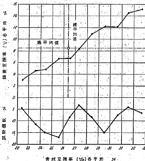
圖—3 表層の骨材空隙率 ( v_a ) 各平均値と鋪装空隙率 ( v ) 各平均値との關係
