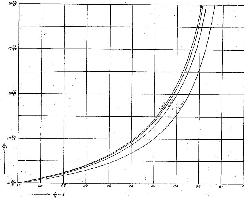
図-7 k - \frac{I_e}{I_0} と \alpha' - \frac{EI_e}{L^3} の関係. \alpha' = \frac{\alpha}{k} .
