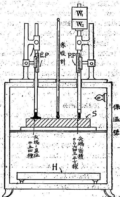
圖-16 軟 化 點 試 験 器
