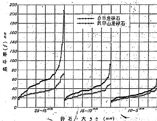
圖—2 碎石粒子の扁平率
