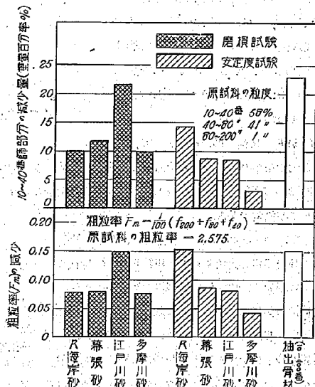
圖-4 各種砂の磨損試験及び安定度試験
