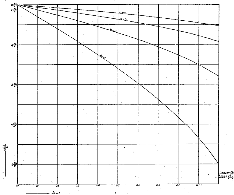
圖-6 k = \frac{I_a}{I_c} と L = \frac{EI_c}{L^2} の關係
