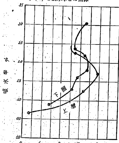
圖-8 表層及び基層の混合物空隙率 ( V ) と吸水率との関係
