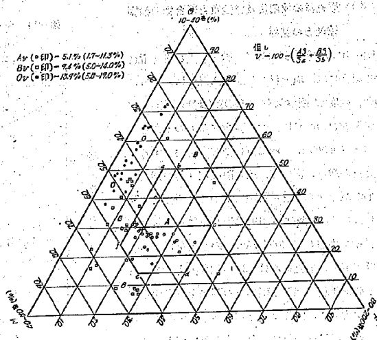
圖-9 トベカ舗装の細骨材部分(10~200番)の粒度と鋪装空隙率との關係
