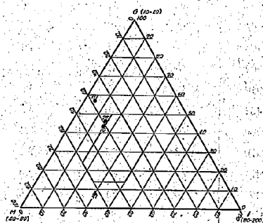
圖一6 (11) 骨材空隙率平均
