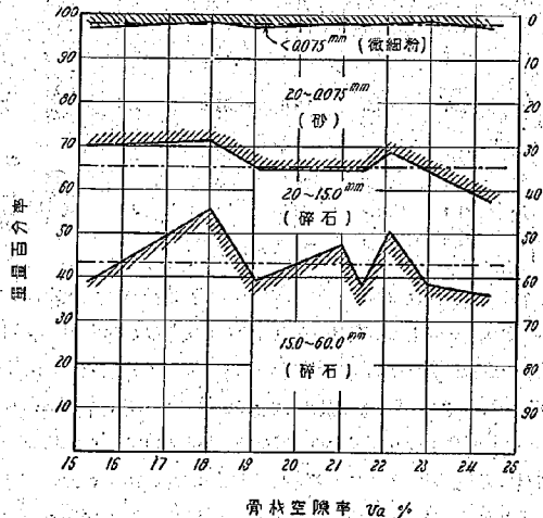
圖-11 基層骨材空隙率 ( v_a ) と骨材粒度との關係
