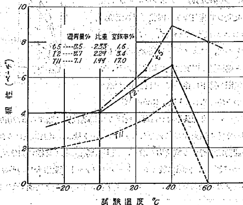
圖-16 トベカ舗装の靱性と試験温度との關係
