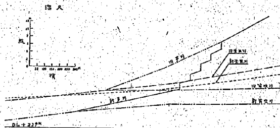
圖—10 釜無川、笛吹川合流點附近縦斷圖
