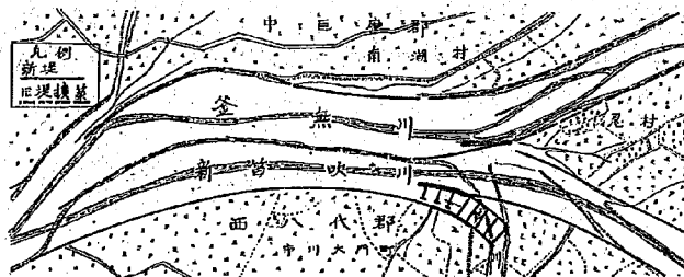
圖一七 釜無川、笛吹川、蘆川 3 川合流點附近平面圖 (1)
