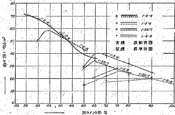
圖-9 水セメント比と曲げ強さとの關係(細粗骨材比 1:2)
