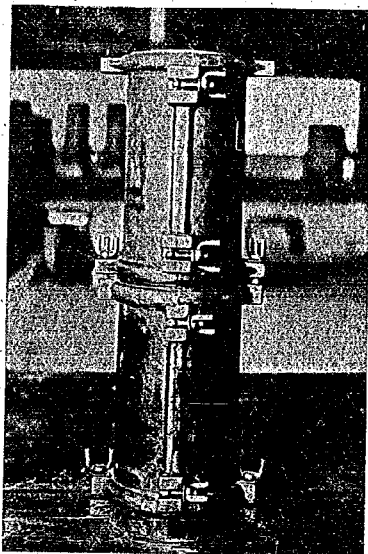
圖一3 振動突固曲げ試験體作成狀況(其の1)
