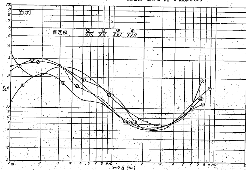
図-7 XIX, XX, XXI, XXII 測定線に於ける \rho_a \sim a 関係を示す
