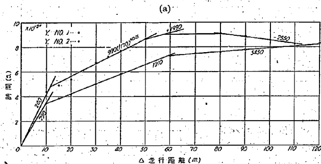
圖—22. 各測定線に於ける走時曲線 (A~D) を示す
