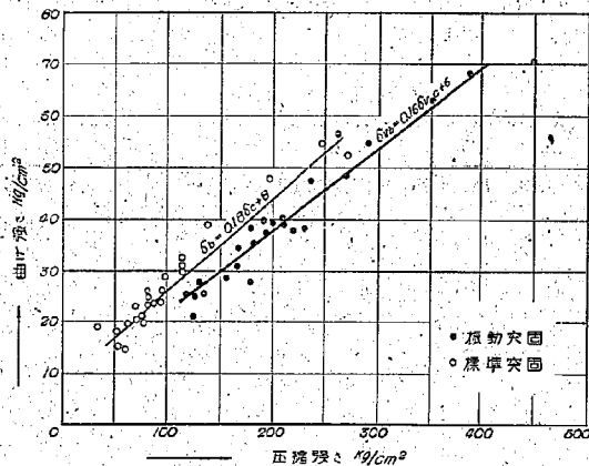
図—12 圧縮強さと曲げ強さとの関係
