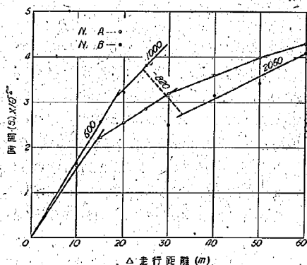
圖-13. 彈性波式實驗の走時曲線(4~2 曲線)
