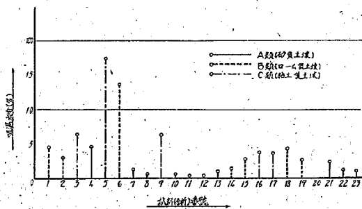
圖-2 機械分析結果
