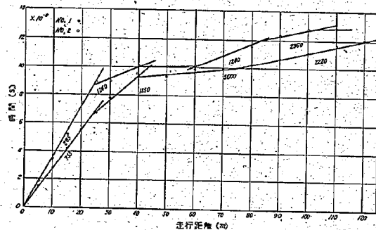
圖-4 I 地域盆地に於ける弾性波式實驗の走時曲線 ( d-v 曲線)
