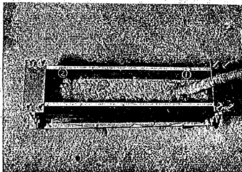
圖一3 振動突固曲げ試験體作成狀況(其の1)
