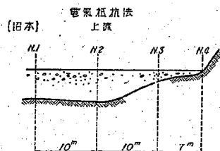
(b) N-1 , N-2 , N-3 による岩盤位置を示す
