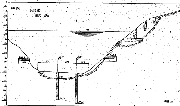
圖-21. 與瀬堤堰豫定地域試錐による岩盤位置
