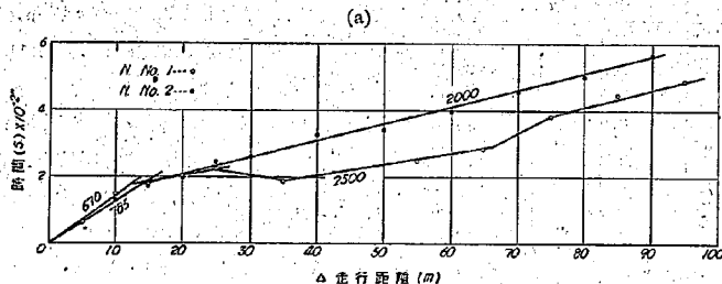
圖-16. 各測定線に於ける走時曲線 ( d-t 曲線)
