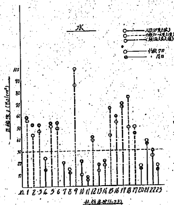
圖-4 壓縮強さと材齢との關係
