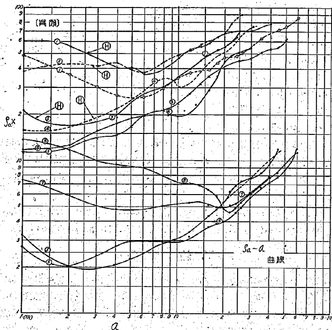
図-24. 各測定線に於ける \rho_a \sim a 曲線を示す
