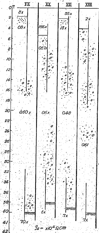
圖-8 \rho_a \sim と地表よりの深さとの關係を示す
