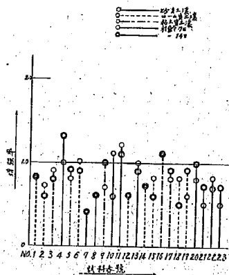
圖-5(4) ボルトランド普通セメント(2%)
