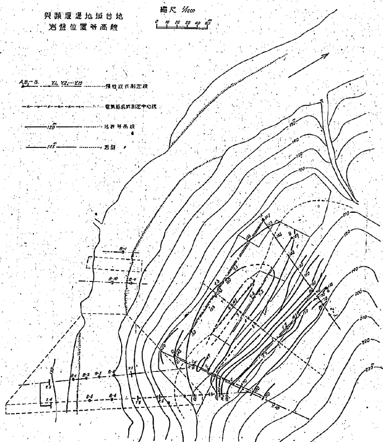
圖-20. 第 III 地域平面圖
