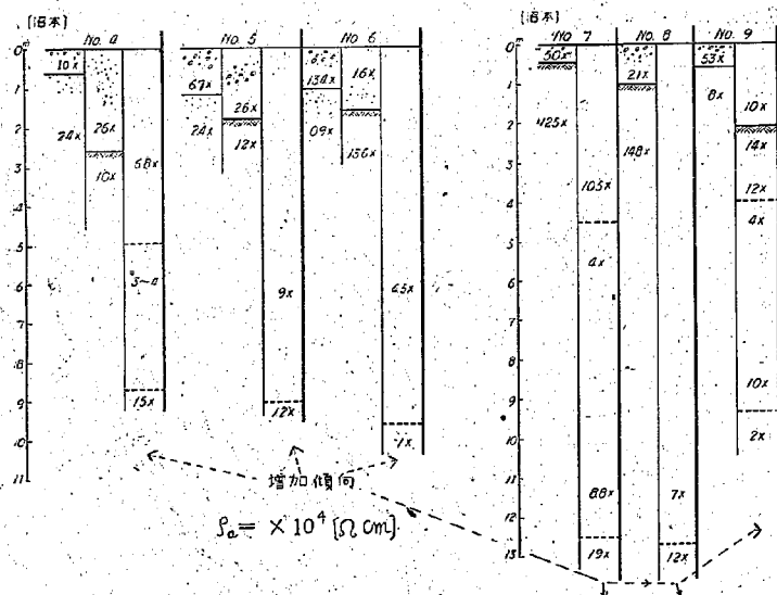
圖-19. \rho_a と地表よりの深さとの關係を示す
