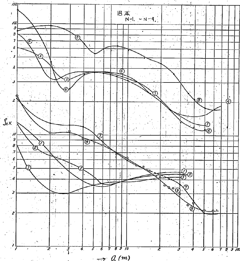
圖-18. 電氣抵抗式實驗に於ける各實測線の \rho_a \sim a 曲線
