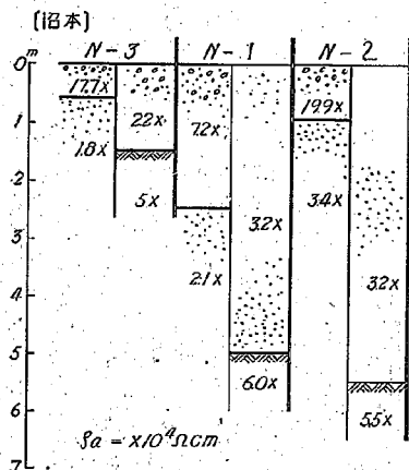
(a) \rho_a と地表よりの深さとの関係を示す
