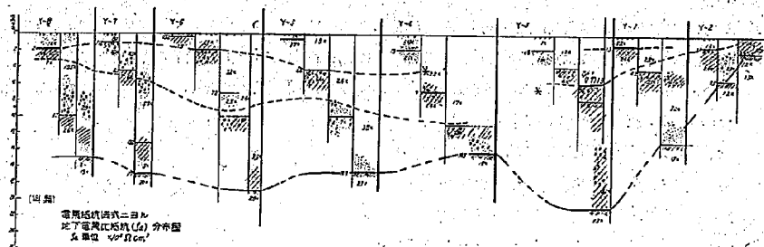
図-25. 各測定線に於ける \rho_a と深さとの關係を示す
