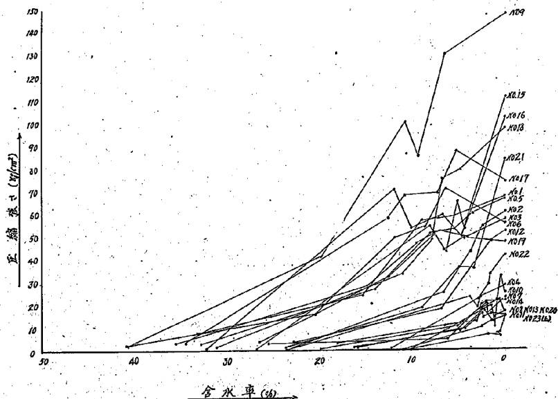
圖-3 含水量と壓縮強さとの關係
