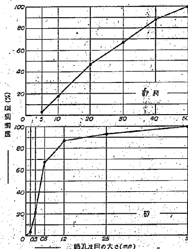
圖-7 砂利・砂の粒度
