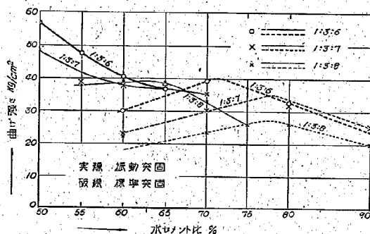
図-11 水セメント比と曲げ強さとの関係 (細粗骨 材比 1:2.33, 1:2.66)
