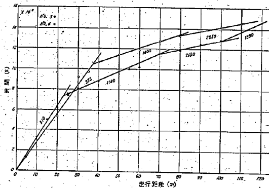
圖-4 I 地域盆地に於ける弾性波式實驗の走時曲線 ( d-v 曲線)
