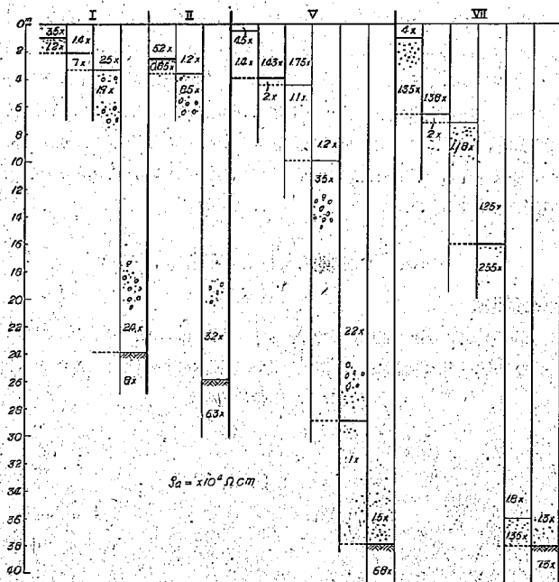
図-10 \rho_a と地表よりの深さとの關係を示す
