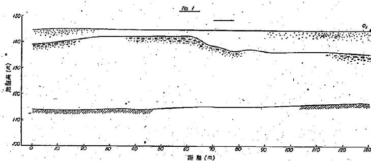
図-6 各測定線に於ける地下構造断面を示す
