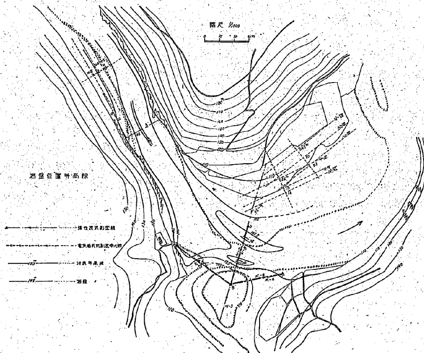
圖-12. 第 II 地域平面圖
