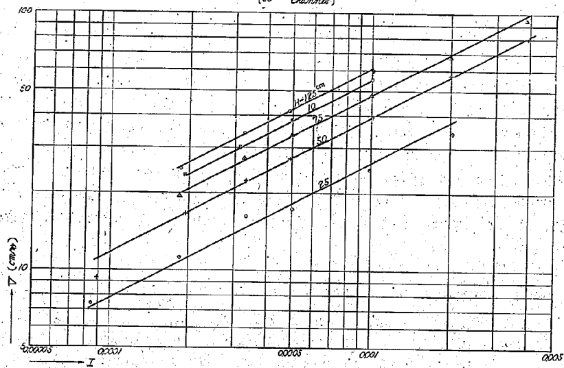
圖-12 幅 70 cm 水路の結果、測點 23 (附表-3)
