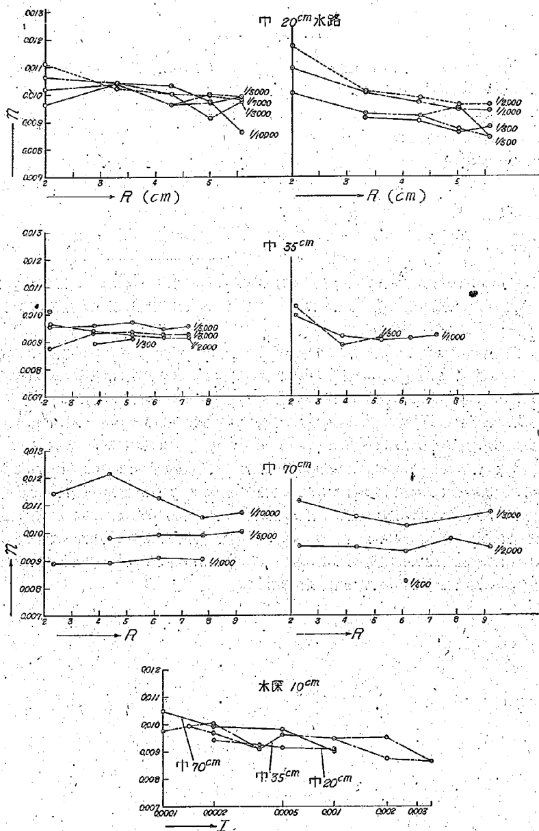
小型水路に於ける流速公式の實驗的研究 圖-20 マンニング指數を採つた場合の R 及 I の變化による n の變化
