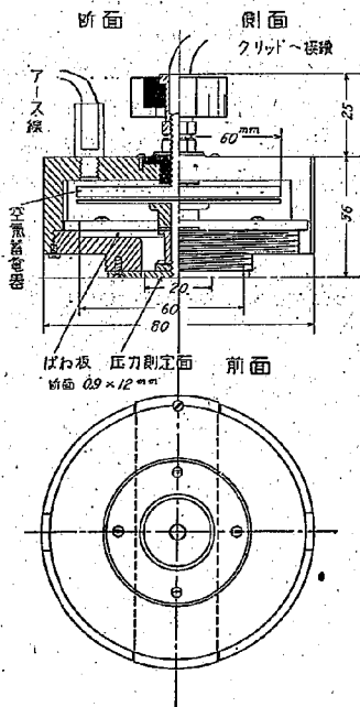
圖—2 (a) 受壓器構造圖
