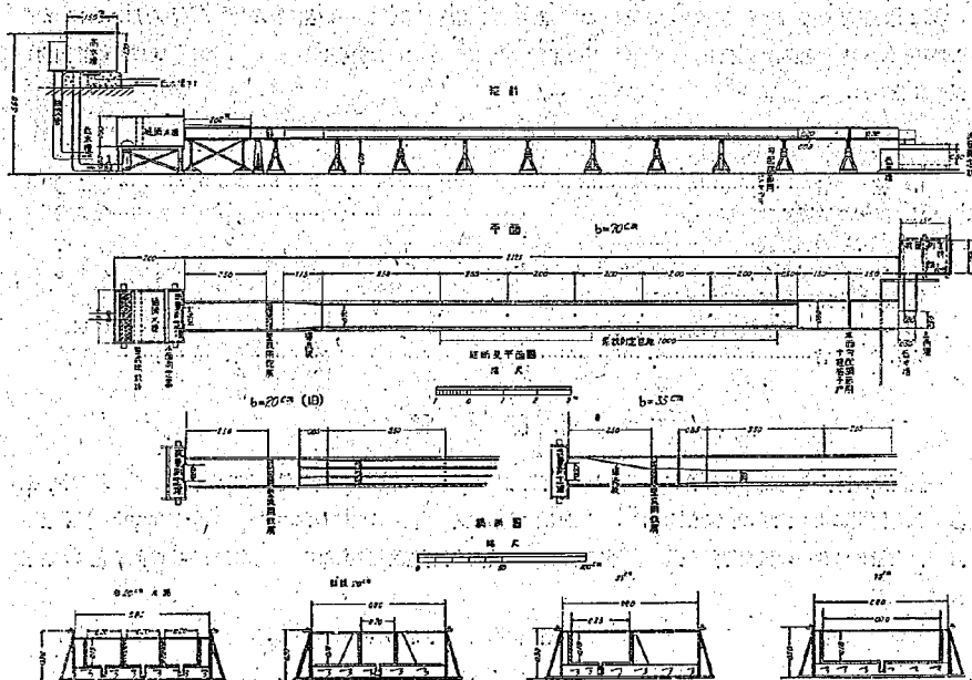
圖—1 試験水路の圖
