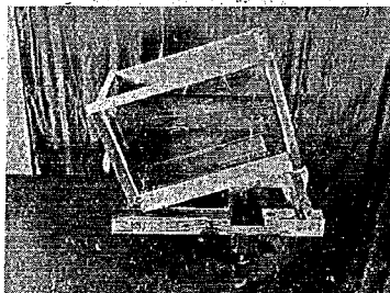
圖-16 面の滑り抵抗測定装置
