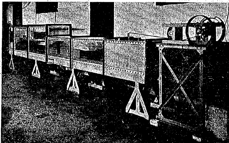
圖-1 (a) 試驗水槽及波起し裝置
