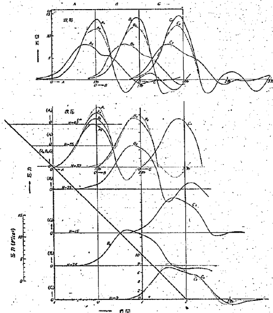
圖-18 45° 傾斜面のみの場合の試験結果 (a) h'=10 cm
