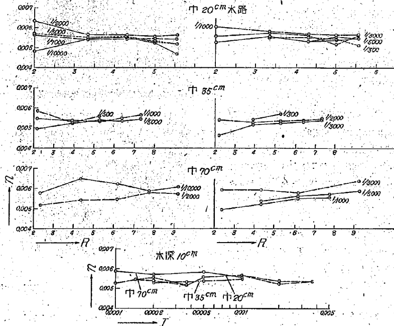
圖-14 R 及 I の變化による n の變化。3 式の平均指數を探り v = \frac{1}{n} R^{0.75} I^{0.54} を採用した場合
