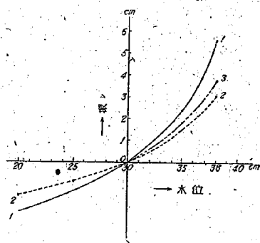
圖-4 壓力檢定曲線
