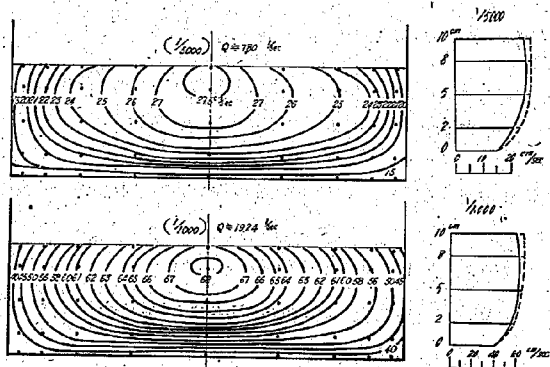
圖一9 幅 70 cm 水深 10 cm 底勾配 1/5000 の流速分布。
