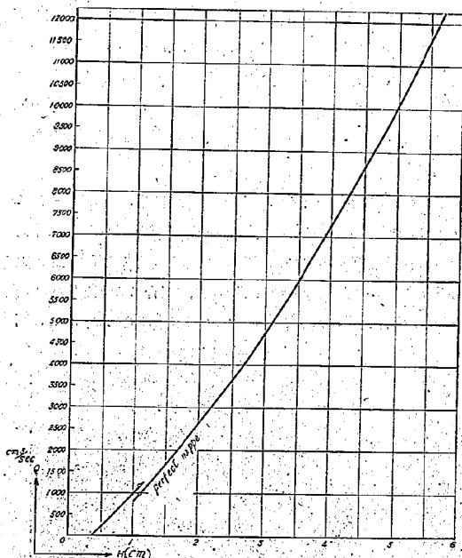
図-6 流量測定堰の検定曲線
