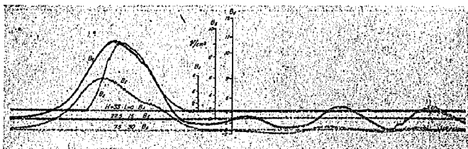
寫真—13 試驗 No. 24 (表—3 及圖—15(a)參照) 階段狀二段壁 h'=10 cm
