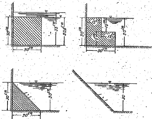
圖-10 試験に使用した異形壁面
