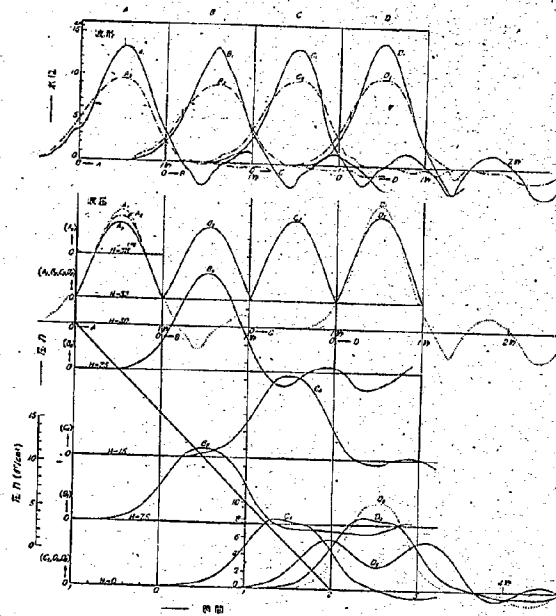
図-17 45°傾斜面上に鉛直壁のある場合の試験結果
