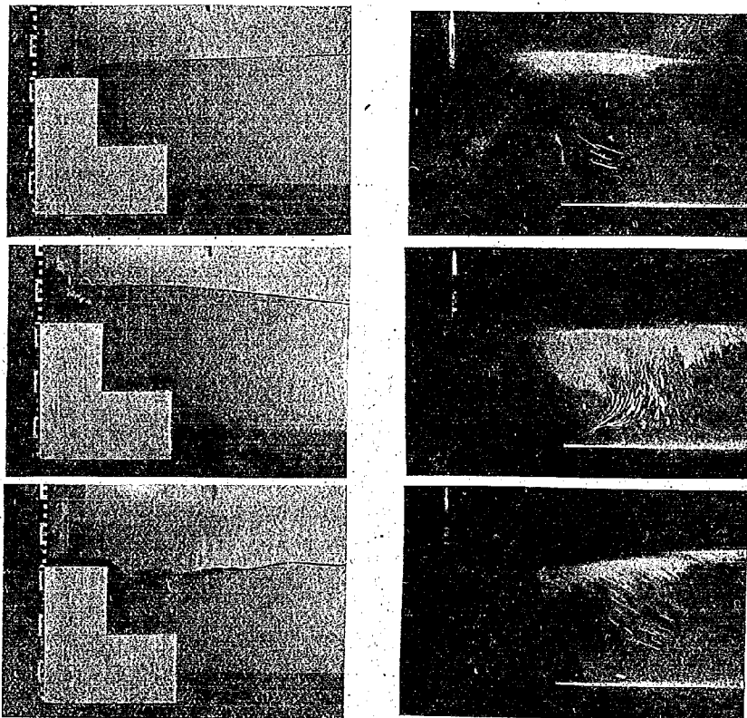
圖—16 階段状二段壁の前面に於ける波形及水の質点部分の運動状態
