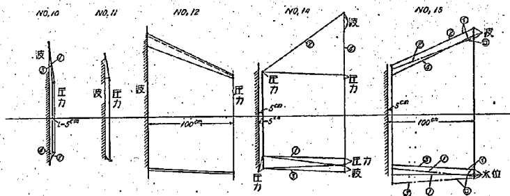
圖-8 底面に作用する圧力の整理結果——鉛直壁の場合
