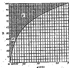
圖一2 小名濱砂篩分曲線
