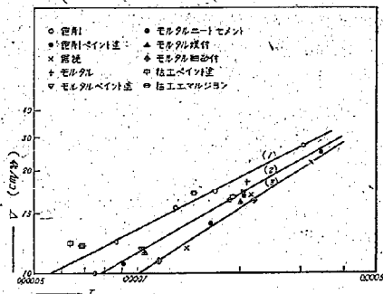
圖-18 各種水路に於ける試驗結果、 底勾配は何れも水平
