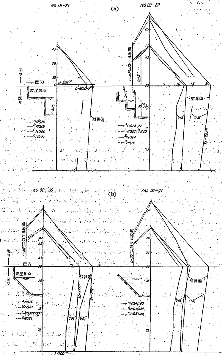
圖-19 異形壁面に於ける測定結果の綜合
