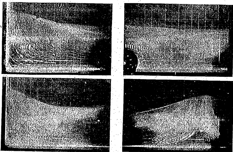
圖-5 鉛直壁に於ける水の質部分の運動狀況
