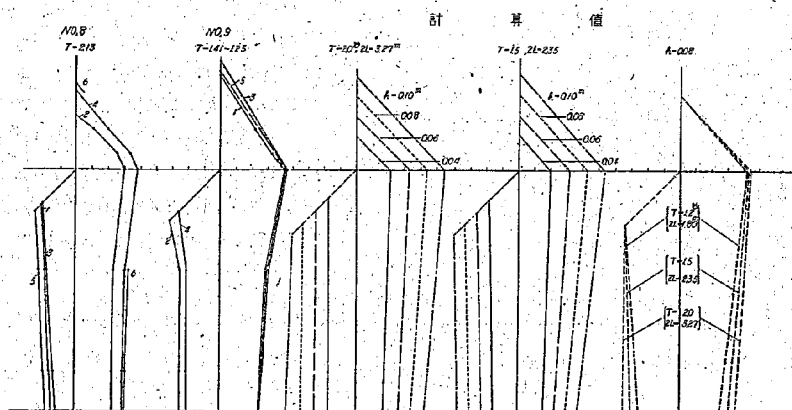
圖-8 底面に作用する圧力の整理結果——鉛直壁の場合
