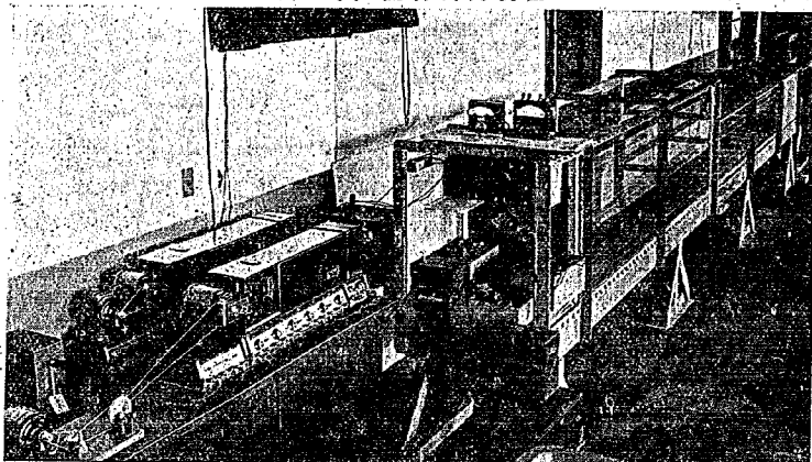
圖—1 (b) 壓力測定裝置
