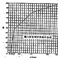
圖—5 鴨川模型用砂礫篩分曲線
