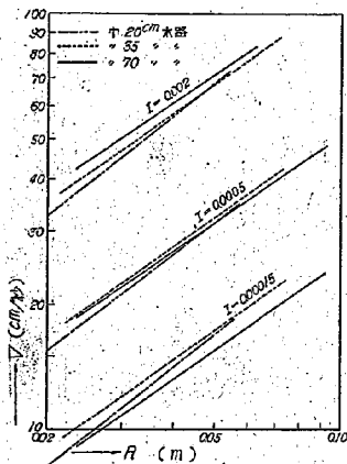
圖-13 R と流速との關係。3 種の幅の水路の中 I=0.00015, 0.0005 及 0.002 だけを示した。
