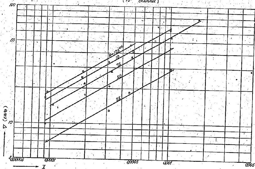
圖-12 幅 70 cm 水路の結果、測點 23 (附表-3)
