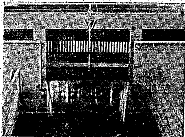
圖—4 流量測定堰
