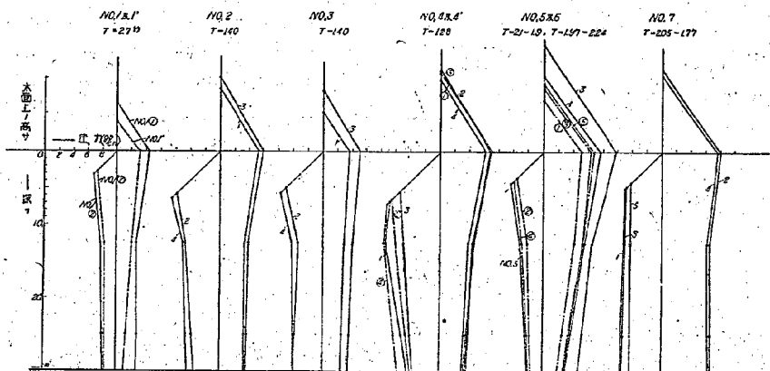
圖-7 鉛直壁に作用する圧力の試験結果と計算値との比較
