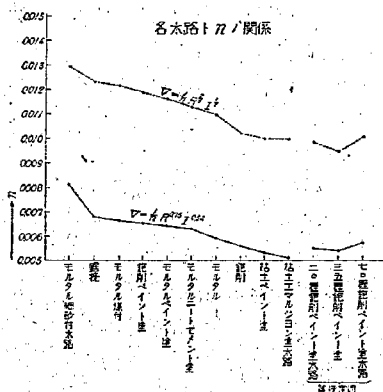
圖-19 各種水路のマンニング係数及新式
