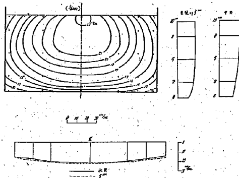
圖一8 幅 35 cm 水深 10 cm 底勾配 1/5000 及 1/1000 の流速分布 右の流速分布断面図の破線は中心 實線は左壁より 8.75 cm の断面である。
