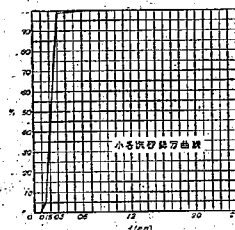
圖二 小名濱砂篩分曲線
