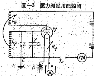
圖-3 壓力測定用配線圖
