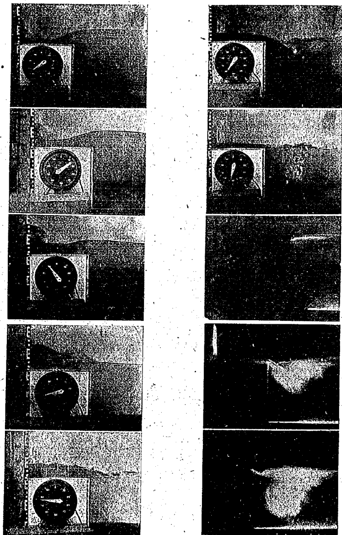
圖-14 階段状一段壁の前面に於ける波形及水の質質部分の運動状態
