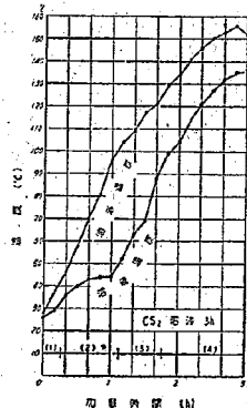
圖一〇 加熱速度と温度上昇との関係
