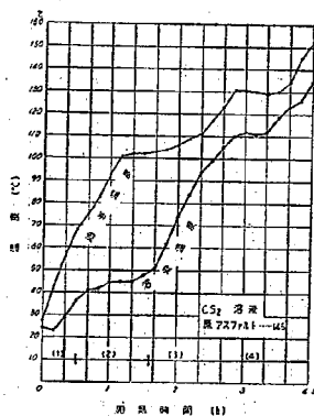
圖一七 加熱速度と温度上昇との関係
