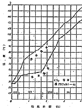
図-4 加熱速度と温度上昇との関係
