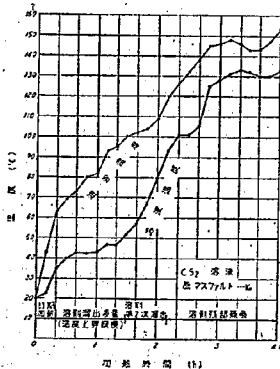
図-3 加熱速度と温度上昇との関係
