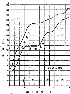
圖-14 加熱速度と温度上昇との關係
