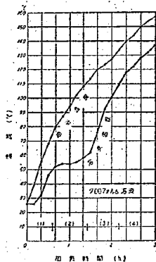
圖-12 加熱速度と温度上昇との關係
