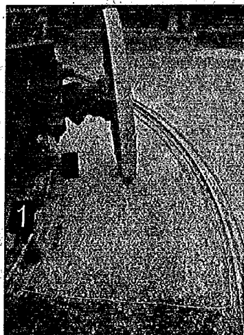
No. 1 生石灰混合砂利道 荷重 (吨) { 純バルーン・タイヤ 2,094.8 混合路綫 { バルーン 2,056.1 鉄 輪 49.0
