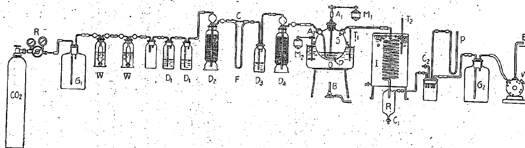
圖-2 アスファルト回収装置
