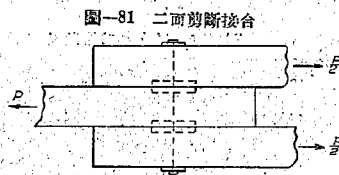
図-81 二面剪断接合
