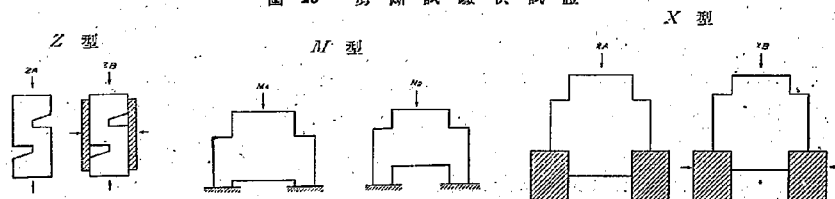
圖—23 剪 断 試 験 供 試 體
