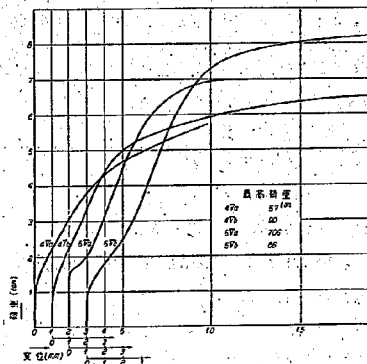
圖-80 4V, 5V の荷重-変位曲線
