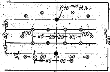
圖—114 ボルト2本コマ形鉄 18個の配置
