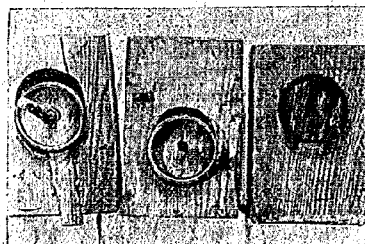
圖—36 破壊後の 4Ia1
