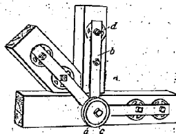
圖-6 S. B. U. デュベルを用いた格點
