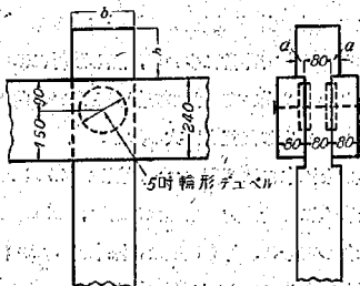
圖—119 輪形デュベル部材切欠併用接合試験供試體
