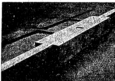
図—113 添木附片側切缺接合の破損状況
