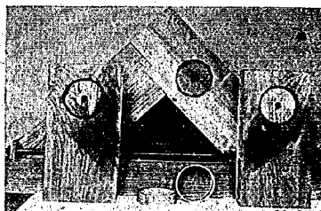
圖-72 4Db の破壊状況
