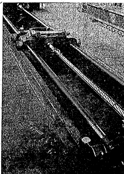
写真--3 C種鋼索の引張試験状況 (引張試験機にて80種積荷したる状態)
