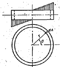
圖-83 輪形デュベルの横方向の應力分布
