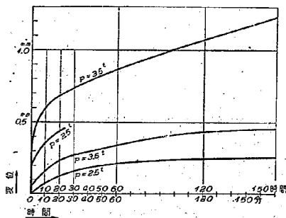
図-85 G. S. スパイク・デュベルの長時間載荷試験表
