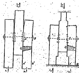
圖-50 引張及壓縮試験の部材の彎曲傾向
