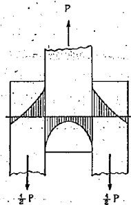
圖-2 ボルト接合の減込變形
