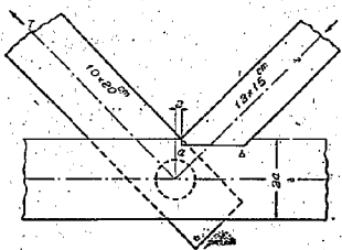
圖-66 45^\circ の斜材を有する供試體
