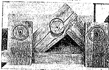
図-74 5Db の破壊状況
