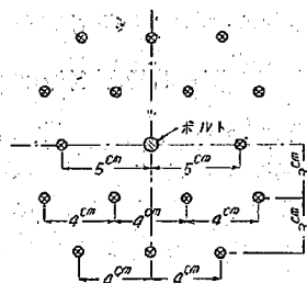
圖—107 コマ形紙配置
