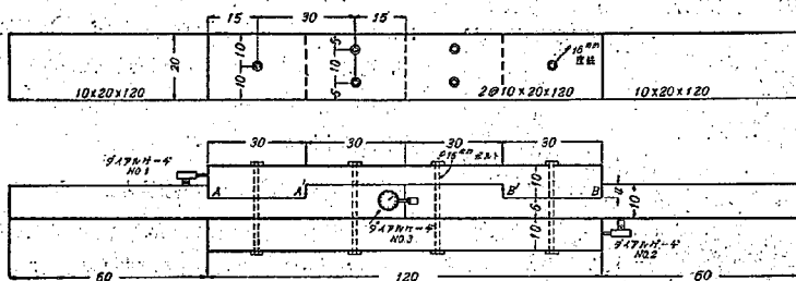
圖—110 添木附片側切缺接合供驗體
