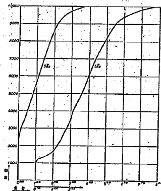
圖-62 5Ia 及 5IIb の荷重-變位曲線
