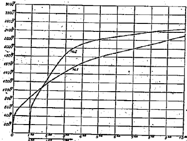
圖-95 ボルト接合の荷重變位曲線
