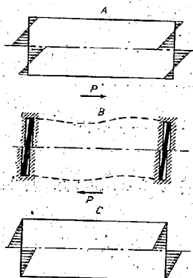
図-84 輪形デュベルトの応力分布の種々の型
