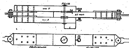
圖—31 引張試験供試體
