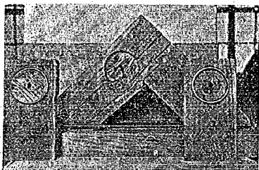
図-73 5Da の破壊状況
