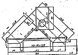
圖-66 45^\circ の斜材を有する供試體
