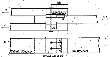
圖-97 鋸接合供試體
