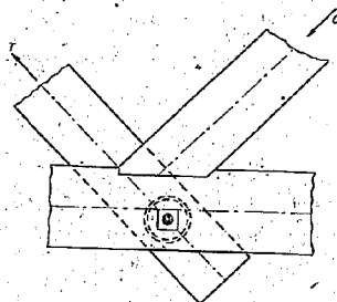
圖-93 格點の構造
