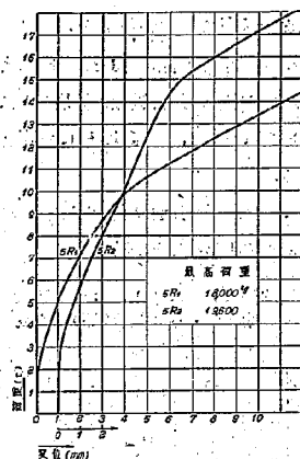
圖-121 sR_1 , sR_2 の荷重-變位曲線
