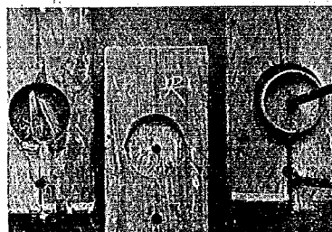
圖—37 破壊後の 4Ia2
