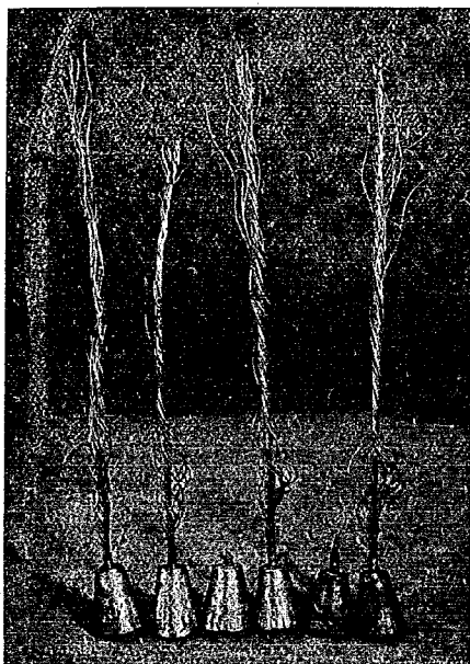
写真--2 C種鋼索用子繩の引張試験後の破断状況
