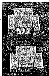
圖—28 XA の破壊状況
