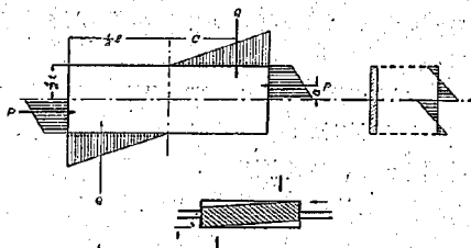
圖-3 デュベル應力分布
