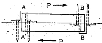
図-53 輪形具デュベル廻轉止め金具
