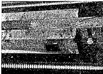
圖-40 4/b' の中央部材の破壊
