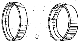
図-19 Locher 型輪形デュベル
