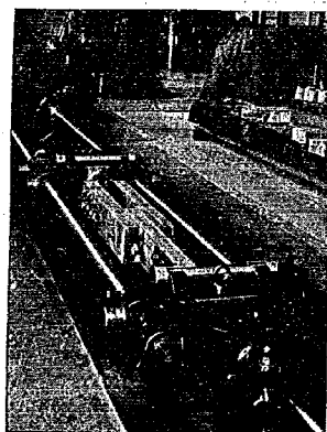
圖—32 引張試験機と供試體
