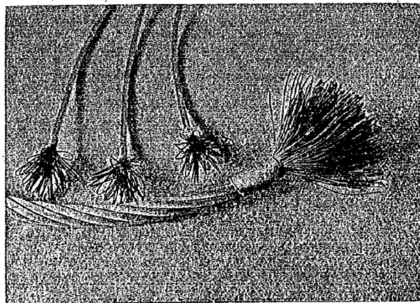
寫眞—1 C種鋼索及び子繩の端部にして合金鑄込み前の狀態
