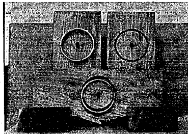
圖-79 5Vb の破壊状況
