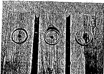
圖-43 4/61 の破壊狀況
