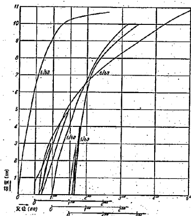
圖—46 荷重と部材間遊離
