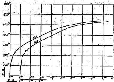
圖一104 荷重—變位曲線
