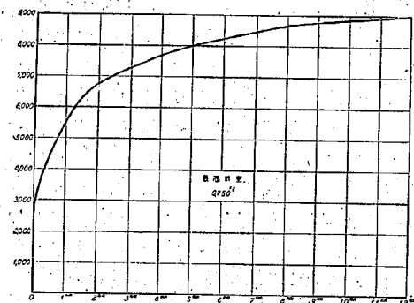
圖-108 荷重—変位曲線
