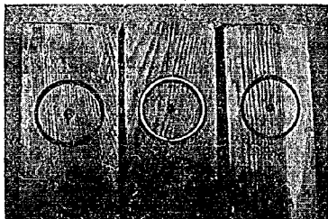
圖-58 5Ib No. 1 の破壊状況
