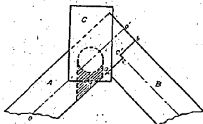
圖-70 弦材と對角材
