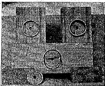
圖-78 5Va の破壊状況
