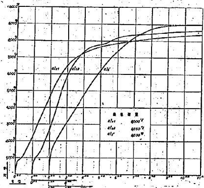
圖-39. 4Ia 及 4Ib' の荷重—變位曲線
