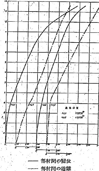
圖—98 鰭接合の荷重—變位及荷重—遊離曲線
