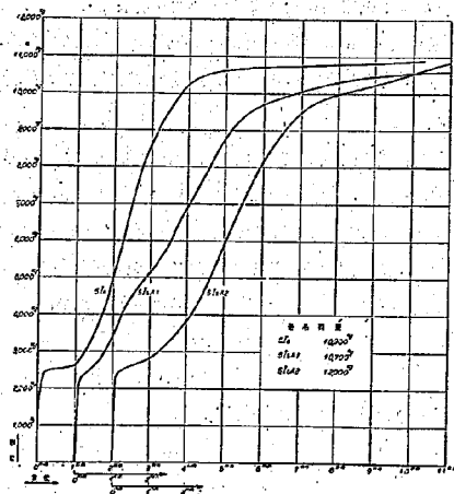
図-56 5/a 及 5/bA の荷重一變位曲線
