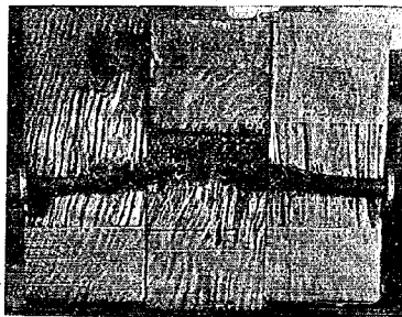
圖-96 ボルトの彎曲
