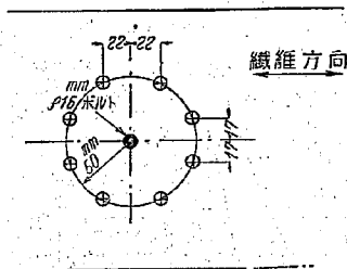
圖一103 コマ形紙8個の配置
