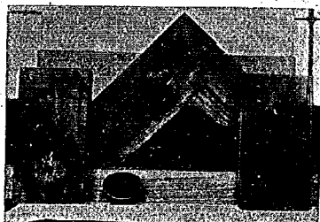
圖-71 4Da の破壊状況
