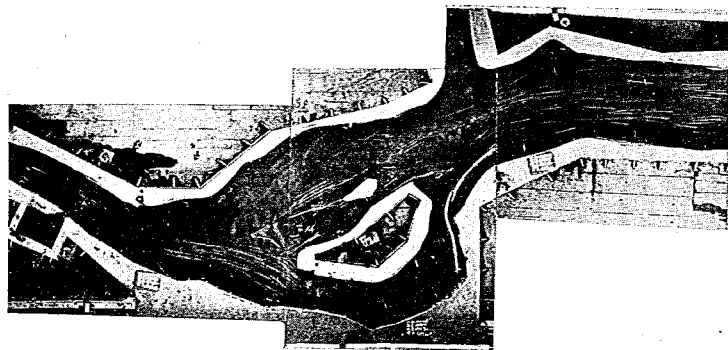
寫真-2(a) 現狀大洪水 寫真露出時間 t=1 秒 實驗番號A-36
