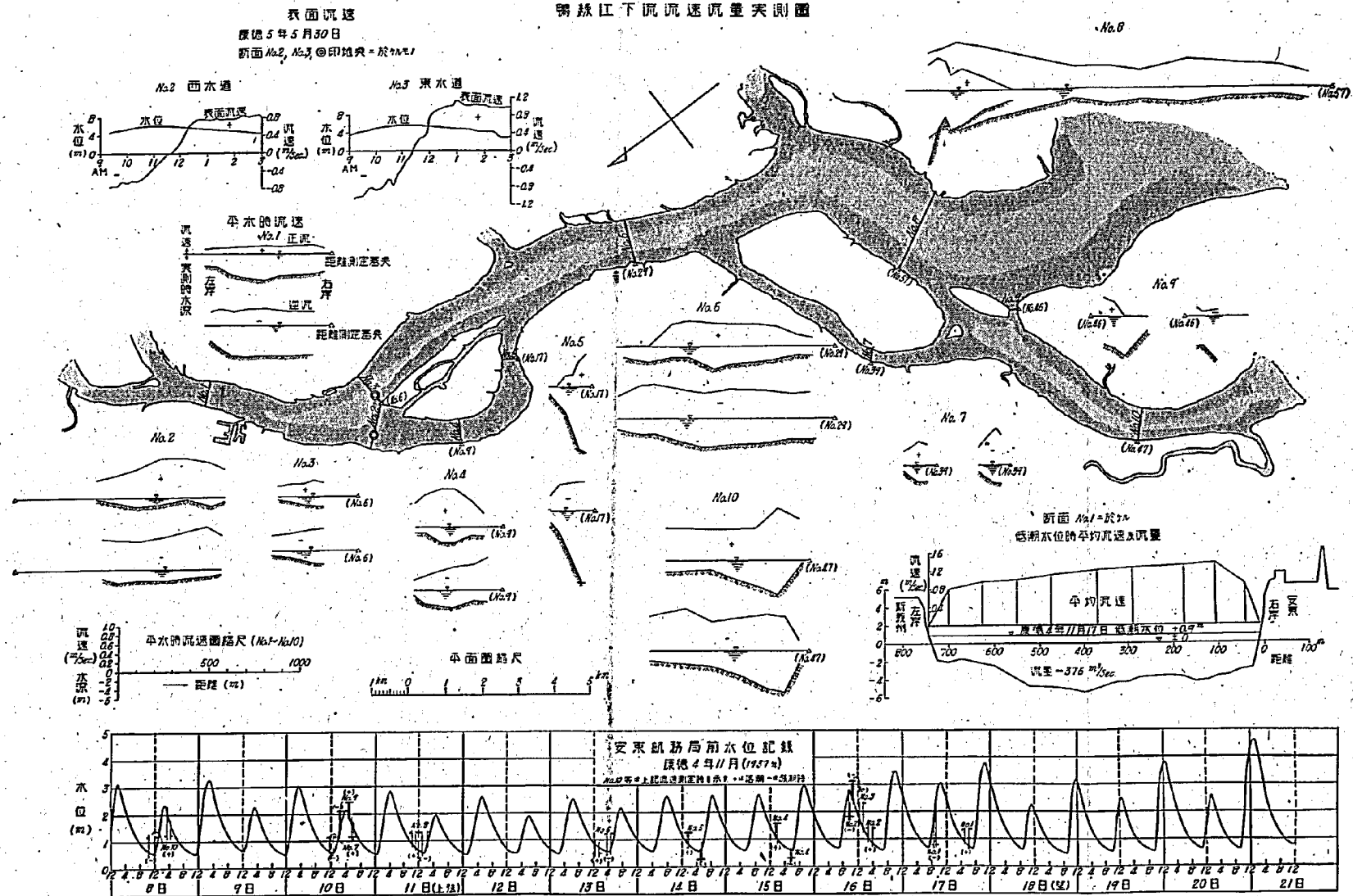
圖-4 鴨綠江下流平水時流速實測圖
