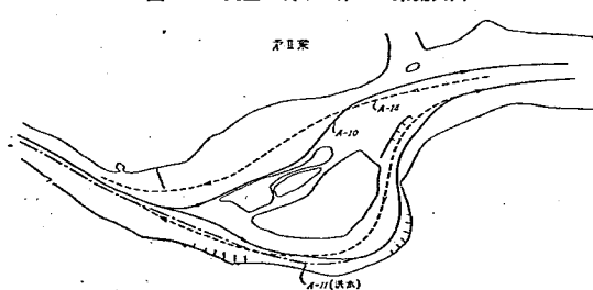
圖一六 模型に於ける第 II 案流向圖
