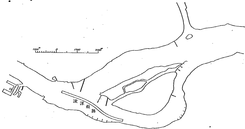
圖-20 試験結果を綜合して得た最も良いと思はれる水制の配置圖 (大體は第 II 案と同様であるが圖中の太線は第 II 案に追加したもの)
