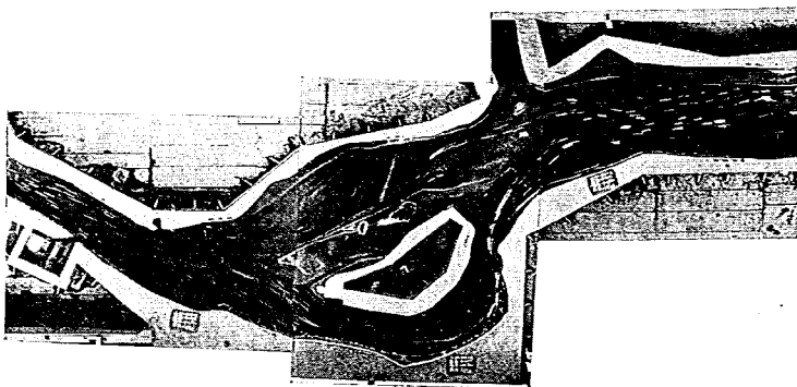
寫眞-3(d) 第Ⅳ案平水順流
