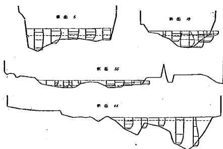
圖—27 平水時順流流速分布圖 第 II 案 (A—10)
