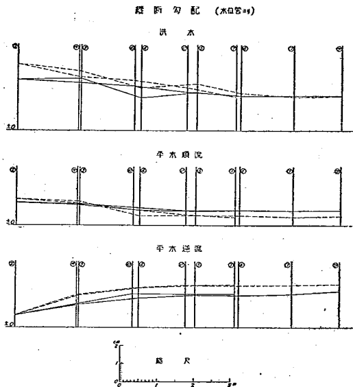
図-11 模型内水面の縦断勾配 ②等は同番號の水位管の位置を示す
