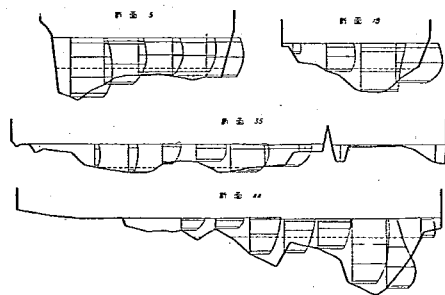
圖-23 洪水時流速分布圖 第 II 案 (A-11)
