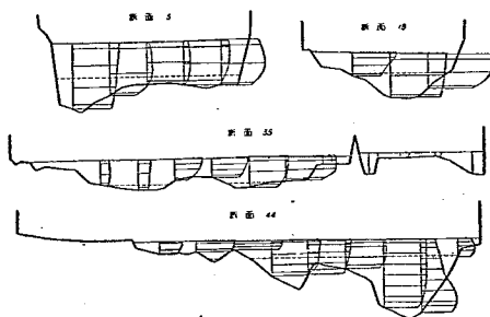
圖—25 平水時順流流速分布圖 現 狀 (A—5)
