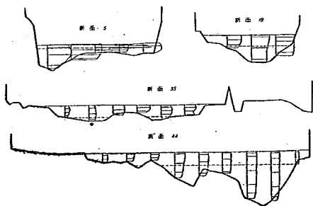
圖—29 平水時逆流流速分布圖 現狀 (A—7)
