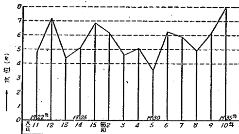
圖-5 1922 年 (大正 11 年) 以降年最高水位 (新義州營林署貯木場調査; 水位基準面明らかならず)
