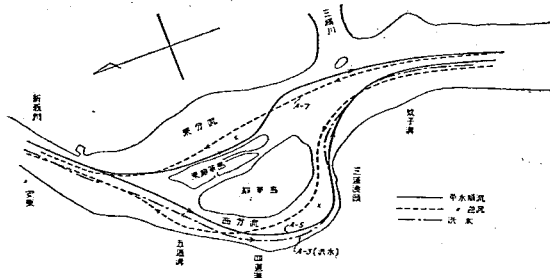
圖一五 模型に於ける第 I 案流向圖
