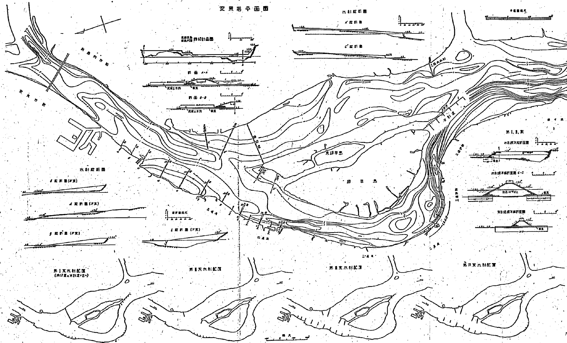
圖-2 安東港平面圖—1937 年 10 月の地形 平面圖の I, II 等は第 II 章に述べる計畫案の第 I 案, 第 II 案等の水制の配置を示したものである
