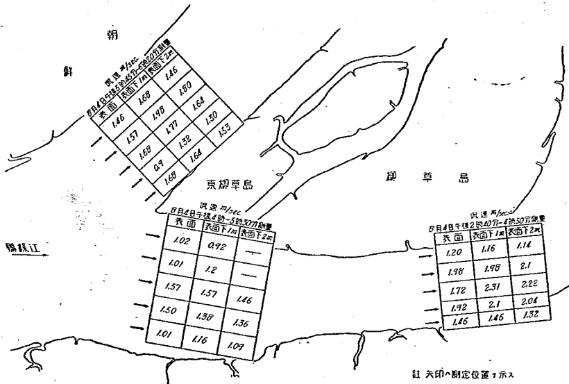
圖一7 1937年(康德4年)8月洪水時流速實測
