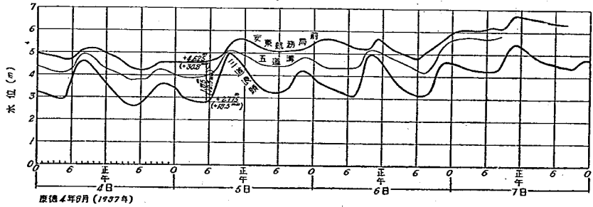
圖一6 1937年(康德4年)8月4~7日洪水水位
