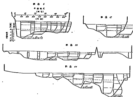
圖-22 洪水時流速分布圖 第 I 案 (A-8)
