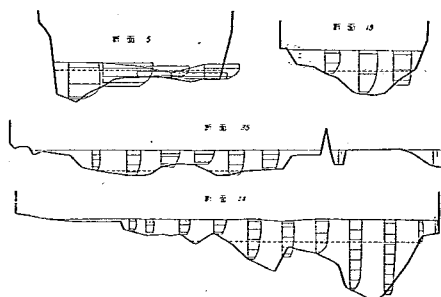
圖-32 平水時逆流流速分布圖 第 III 案 (A-15)
