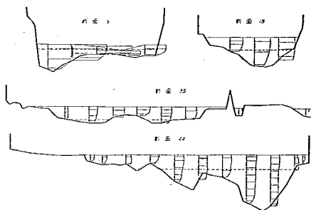
圖-31 平水時逆流流速分布圖 第 II 案 (A-14)
