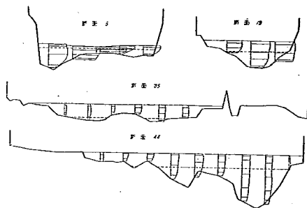
圖-30 平水時逆流流速分布圖 第 I 案 (A-6)
