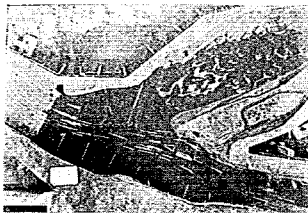
寫眞-8 合流點附近流向又河底移動狀態
