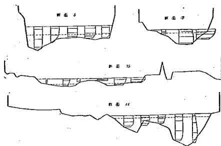
圖—28 平水時順流流速分布圖 第 III 案 (A—17)
