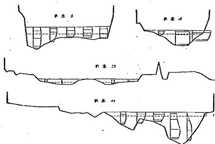
圖—26 平水時順流流速分布圖 第 I 案 (A—9)
