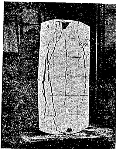
寫眞—5 破壊後の供試體Ⅱ
