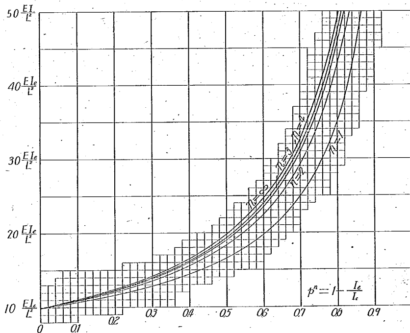
圖-3 \frac{PL^2}{EI_e} と \frac{I_e}{I_c} の關係
