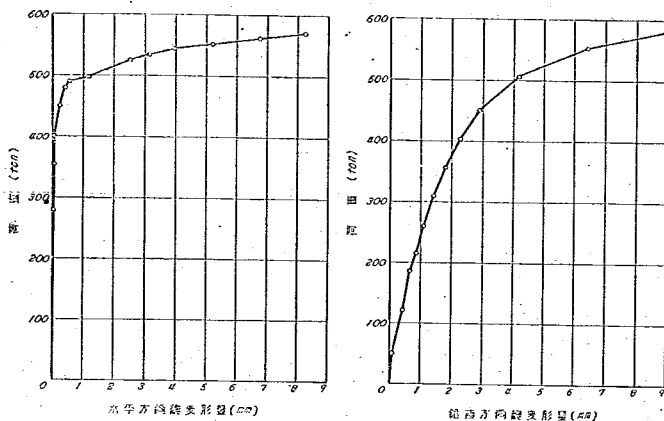
圖-6 供試體Ⅰに於ける荷重と總變形量との關係
