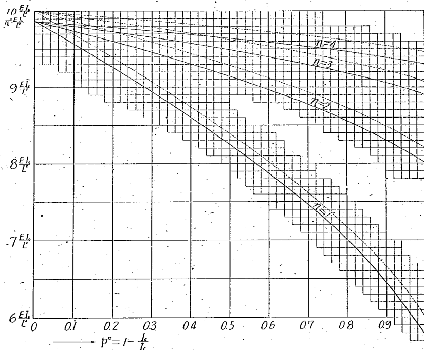
圖-2 p^n = 1 - \frac{I_c}{I_c} と 4a^2 = \frac{PI_c^2}{EI_c} の關係
