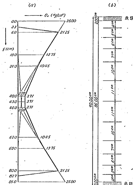
圖-3 引張應力の分布並びに引張鉄筋間隔の決定
