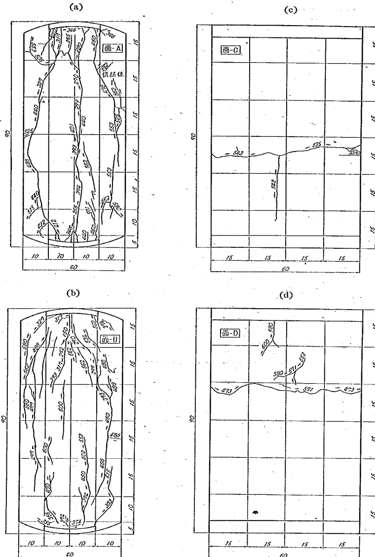
図-5 供試体 I の亀裂状態
