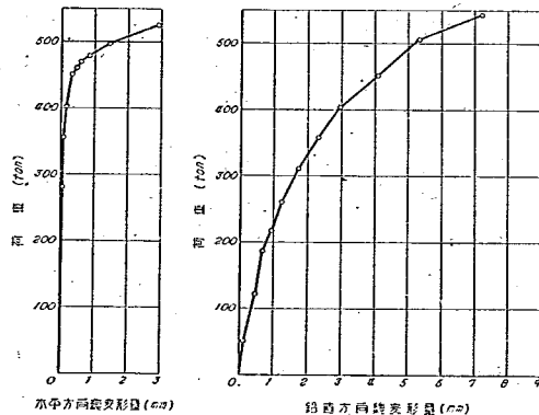
圖-8 供試體Ⅱに於ける荷重と總變形量との關係
