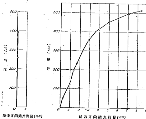
圖—10 供試體 III に於ける荷重と總變形量との關係
