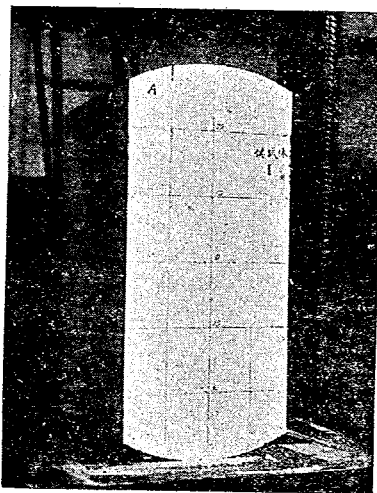
写真-4 載荷前の供試体 II
