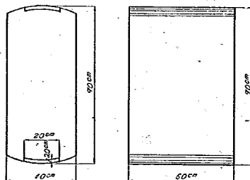
圖一 ロッカーの形狀及び寸法
