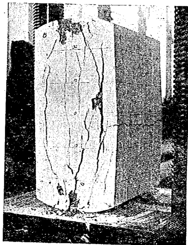
寫眞—5 破壊後の供試體Ⅱ
