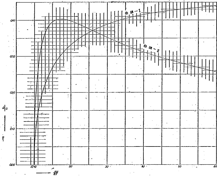
図-3 \frac{PL^2}{EI} と \frac{y_0}{L} の関係
