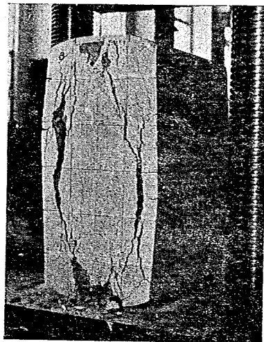
寫眞—3 破壊後の供試體Ⅰ
