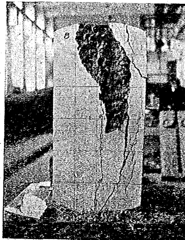
写真—7 破壊後の供試体Ⅲ
