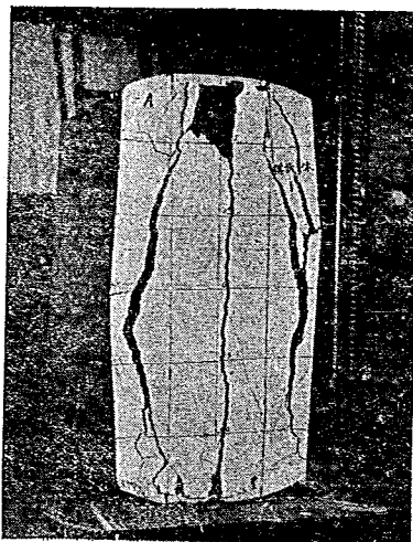
寫眞—3 破壊後の供試體Ⅰ
