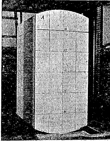
写真—6 載荷前の供試体Ⅲ
