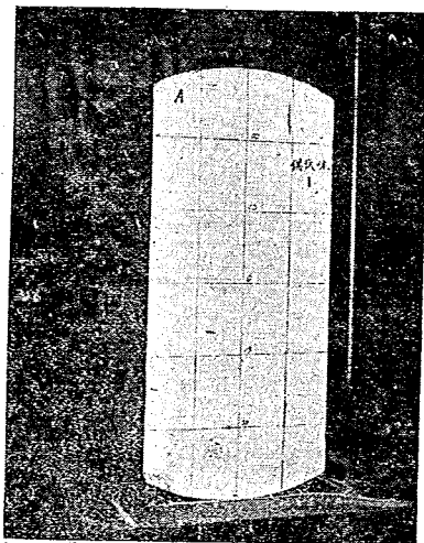
写真-2 載荷前の供試体 I
