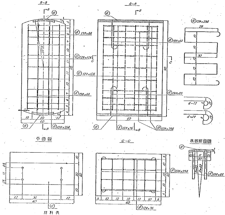
図-4 鉄筋コンクリートロッカー構造図
