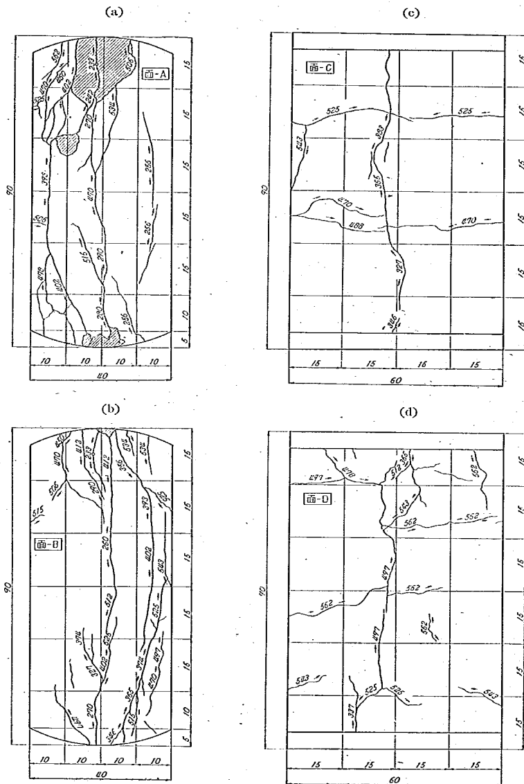
圖-9 供試體Ⅲの亀裂状態
