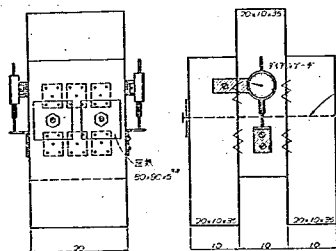
圖-1 「噛合せデュベル」接合試験體 Ⅳ 6
