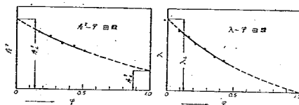
圖-42 k^2 \sim \varphi , \lambda \sim \varphi 標準圖
