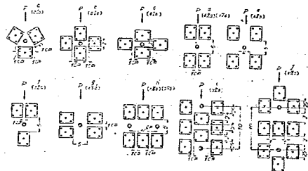
図-4 デュベル配置図
