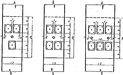
図-20. 3Ⅱa, 4Ⅱa, ⅣⅢ6 のデュベル配置
