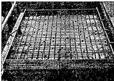
寫眞-1 コンクリート打ち直前の状況
