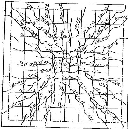
図-20 破壊に達するまでの板の下面の龜裂進行状態
