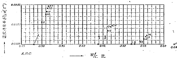
圖-3-5; k^2 \sim W/C の關係
