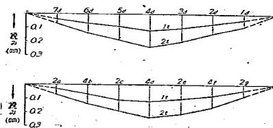
図-20 破壊に達するまでの板の下面の龜裂進行状態
