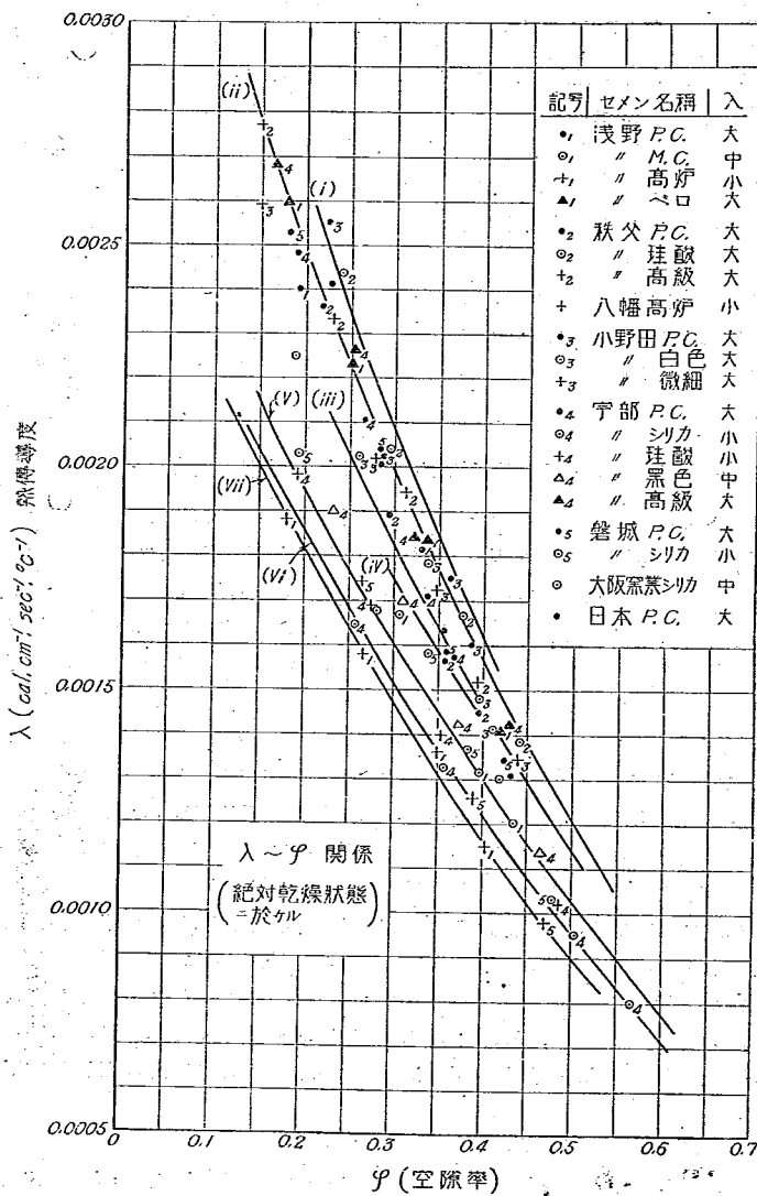
圖-43 \lambda \sim \phi 一覽圖
