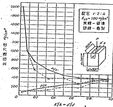
図-6 \frac{A'}{A} = \frac{d'}{d} と \frac{P}{A} 及び \frac{P}{A'} との関係
