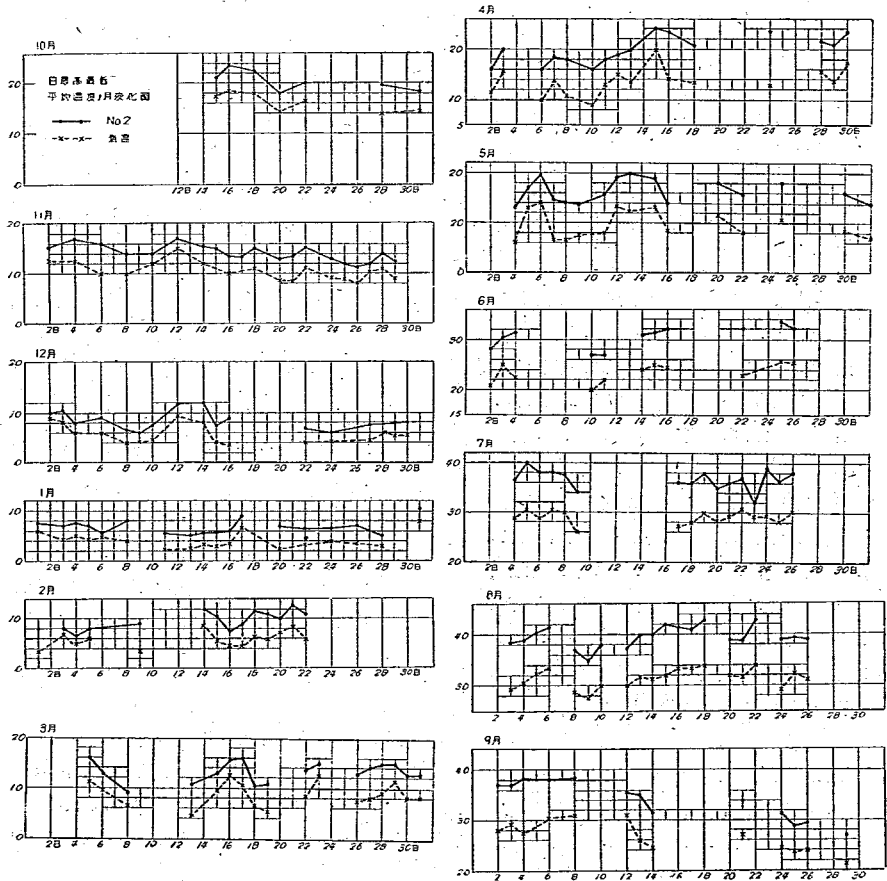
圖—10 舗装コンクリート版表面温度及気温の日平均温度の月變化
