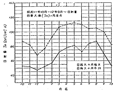
図-6 日射量日最大の月平均 J_0 及月最大の年変化圖
