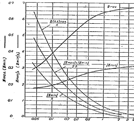
図-4; \alpha' J_0 \Phi_{\max} と h との關係を示す
