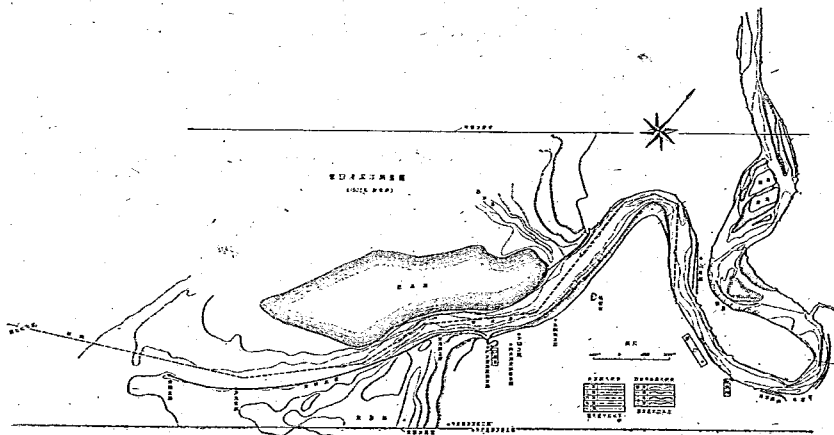
圖-15 遼河々口深淺測量圖
