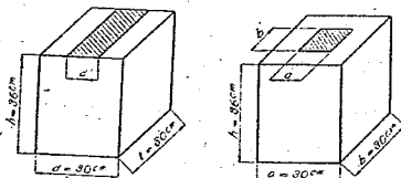
圖-5 供試體の寸法
