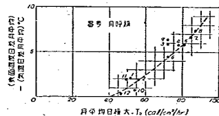
図—14 (表面温度日差月平均) - (気温日差月平均) と日射量日極大月平均 ( J_0 ) との関係
