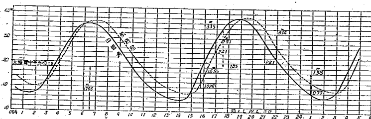
圖-21 航務局一四道溝水位曲線圖
