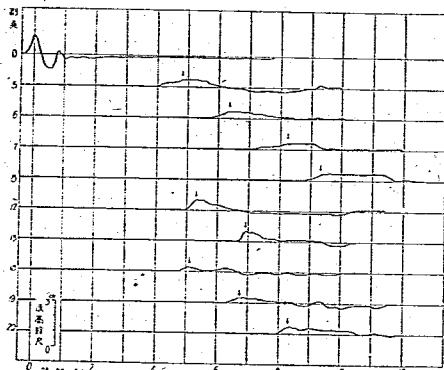
圖-36 押波の形圖
