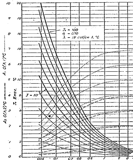
図-4; \alpha' J_0 \Phi_{\max} と h との關係を示す
