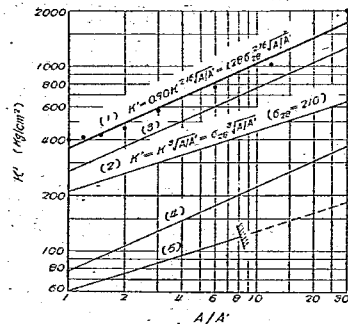
圖—8 示方書規定の公式と試験結果との比較 (帯荷重の場合)
