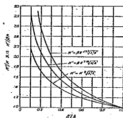
図-10 \frac{A'}{A} と \frac{K'}{K} 又は \frac{K'}{\beta K} との関係
