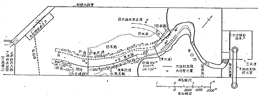
圖—20 a 模型平面圖
