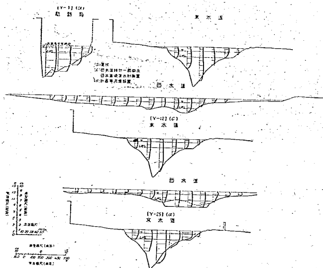
圖-32 上潮時，中等潮位，試驗(Y-1) 現状 t = 1 秒
