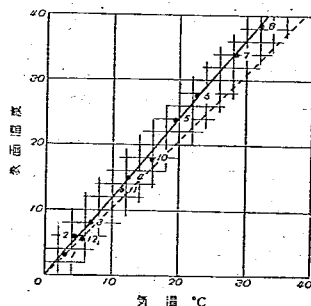
圖-11-a, b 鋪裝表面温度と気温の日最大最小温度月平均
