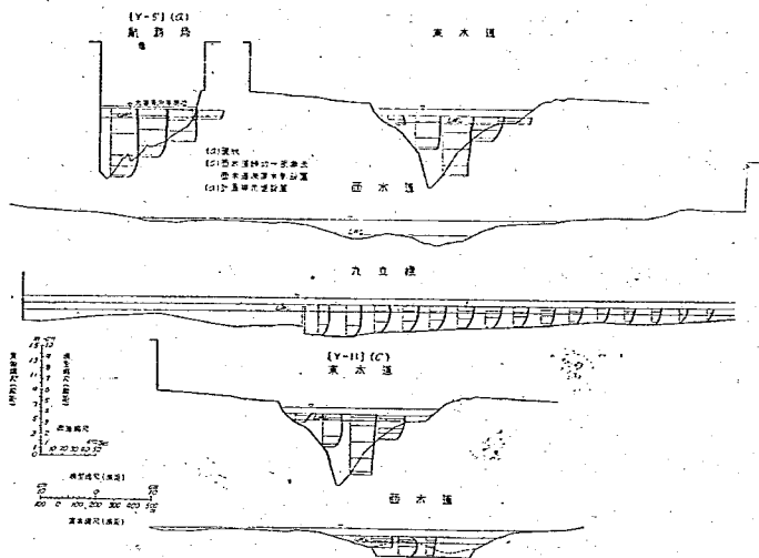
圖-29 下潮時, 低潮位, 試験 (Y-5') 現状, t = 1 秒
