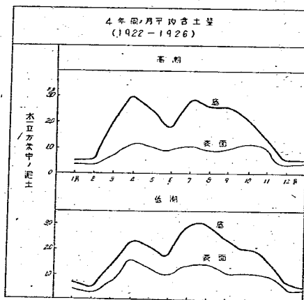
圖-11 港内に於ける河水の含土量
