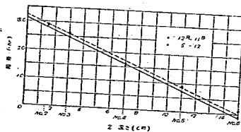
圖—9—b Fourier 級數展開 式第一項相差と深 さ z との關係圖
