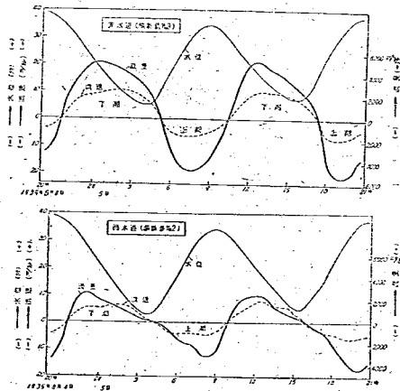
圖一九 東西水道の貨河水位流速、流量
