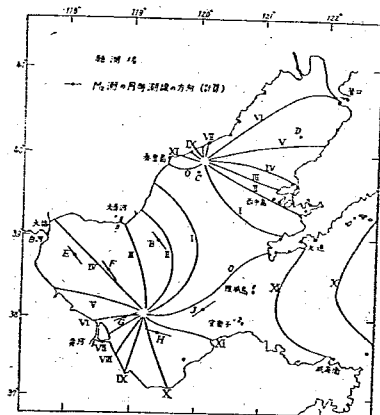
圖-5 渤海灣に於ける同時潮圖及潮流圖
