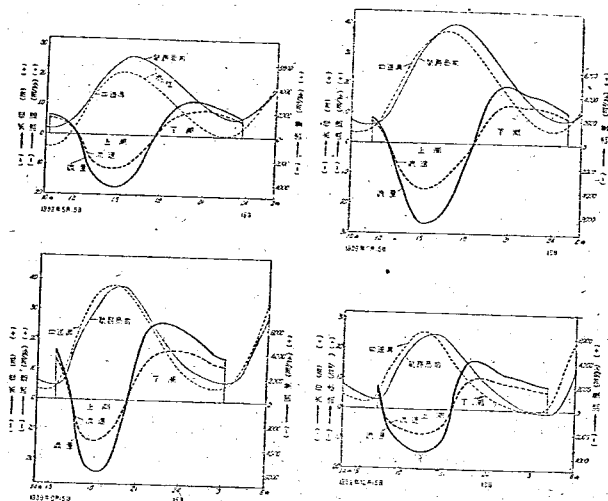
圖一八 西水道締切内外の水位
