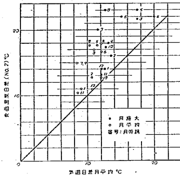
図—13 表面温度日差と気温日差月平均との関係
