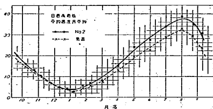
圖-11-a, b 鋪裝表面温度と気温の日最大最小温度月平均
