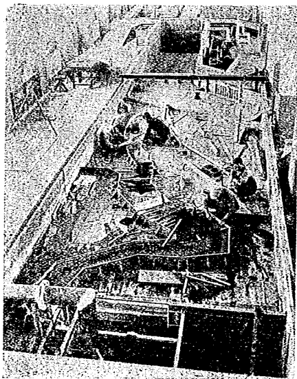
圖—20 b 模型製作中の寫眞
