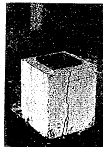
寫眞-11 A' = 18 \times 18 = 324 \text{ cm}^2 の場合
