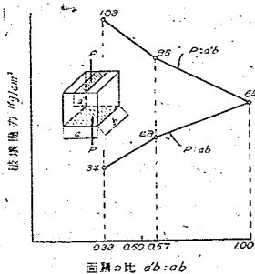
圖-4 コンクリートに就いての Graf の實驗結果
