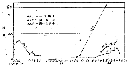
圖-9 實河流量圖
