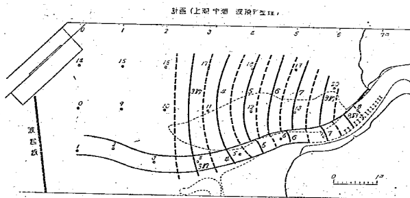
圖-38 押波の傳播状況 (計畫)
