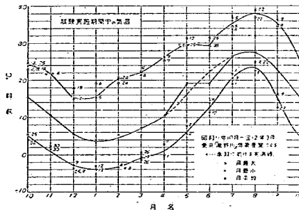
図-7 試験現場に於ける気温日最大最小の月最大最小値図
