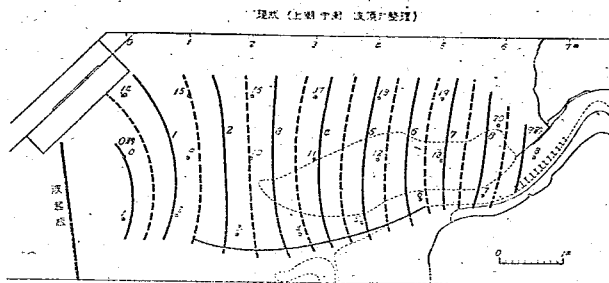
圖-37 押波の傳播状況 (現狀)
