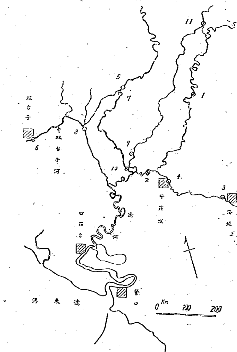
圖-8 遼河流量調査位置平均平面圖
