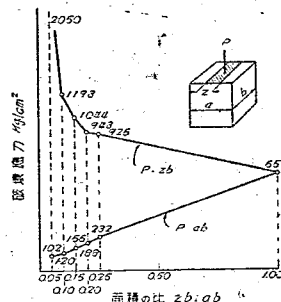
圖-3 砂岩に就いての Bach の實驗結果
