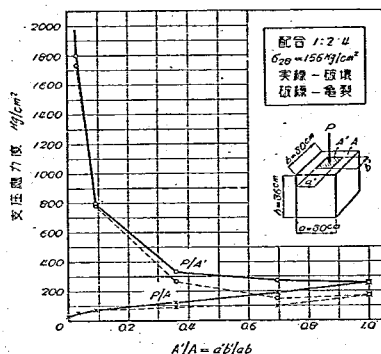
図-7 \frac{A'}{A} = \frac{a'b'}{ab} と \frac{P}{A} 及び \frac{P}{A'} との関係
