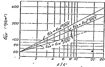
図-12 筆者の提案せる式と現行規定の式との比較
