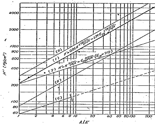
図-9 示方書規定の公式と試験結果との比較(点荷重の場合)
