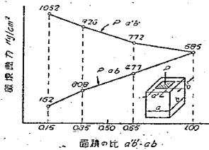
圖-4 コンクリートに就いての Graf の實驗結果
