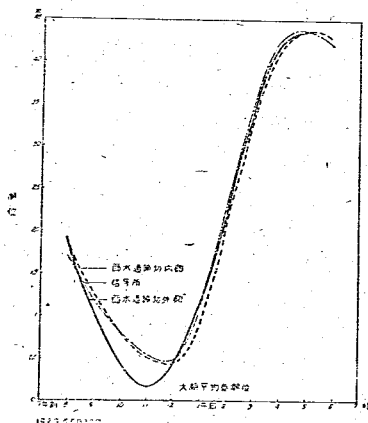
圖一八 西水道締切内外の水位
