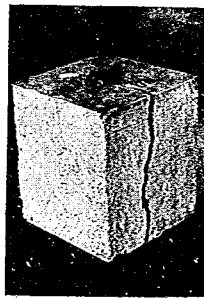
寫眞-13 A' = 5 \times 5 = 25 \text{ cm}^2 の場合
