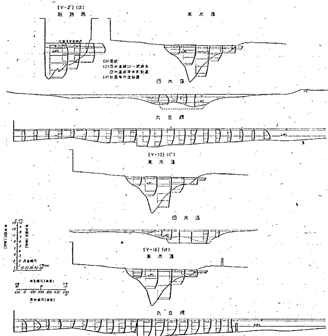
圖-24 模型流速曲線、下潮時、中等潮位
