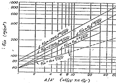
図-11 (6) 式又は (8) 式に於ける係数を 1 とした場合の許容支圧應力度
