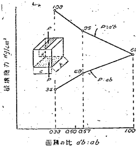
圖-4 コンクリートに就いての Graf の實驗結果
