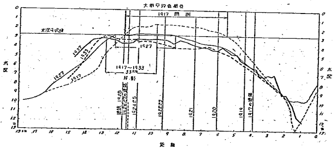
圖-14 導流堤の延張に伴ふ門洲の移動縦斷圖
