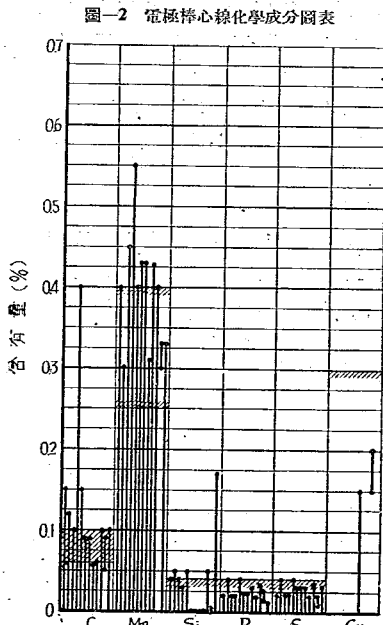
圖-2 電極棒心線化学成分圖表
