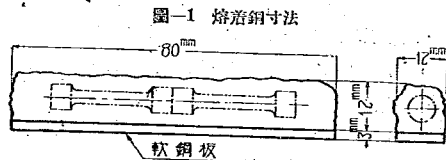
圖-1 熔着鋼寸法
