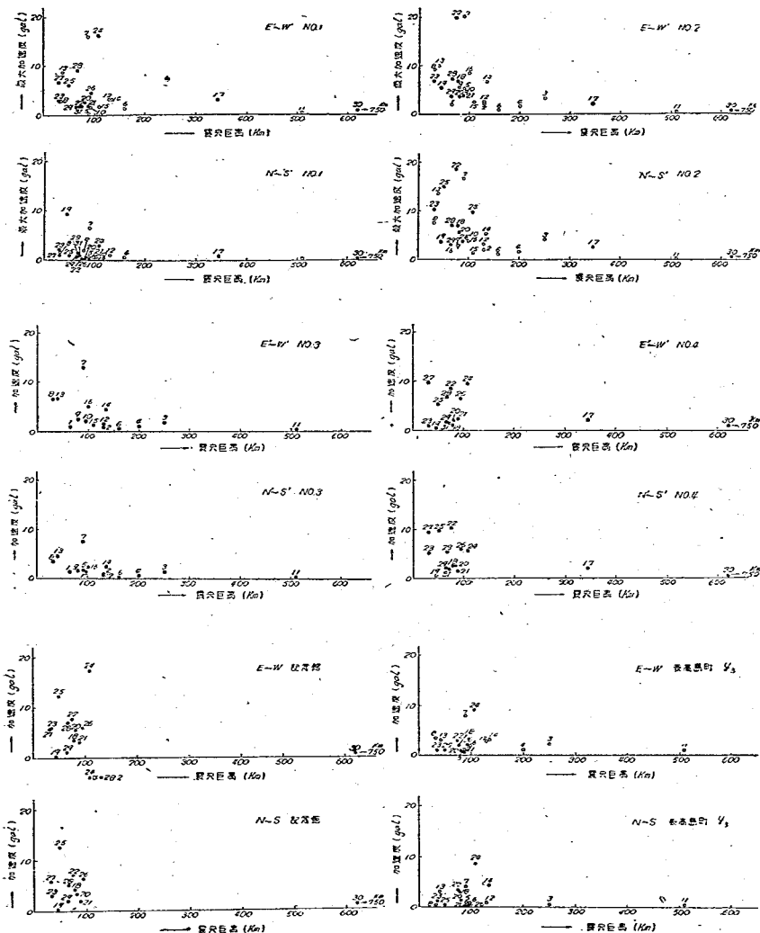
図-2 震央距離と各地點の最大加速度
