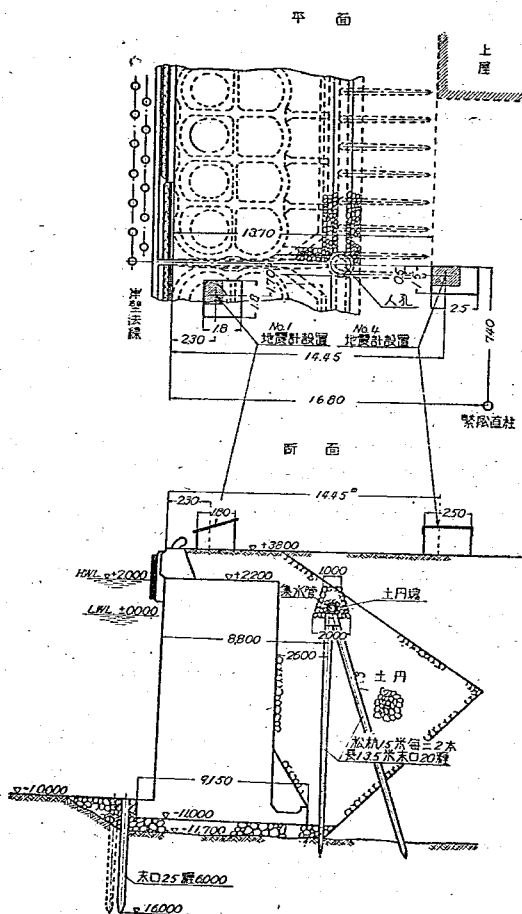
圖一1 地震計 No. 1 及 No. 4 設置位置
