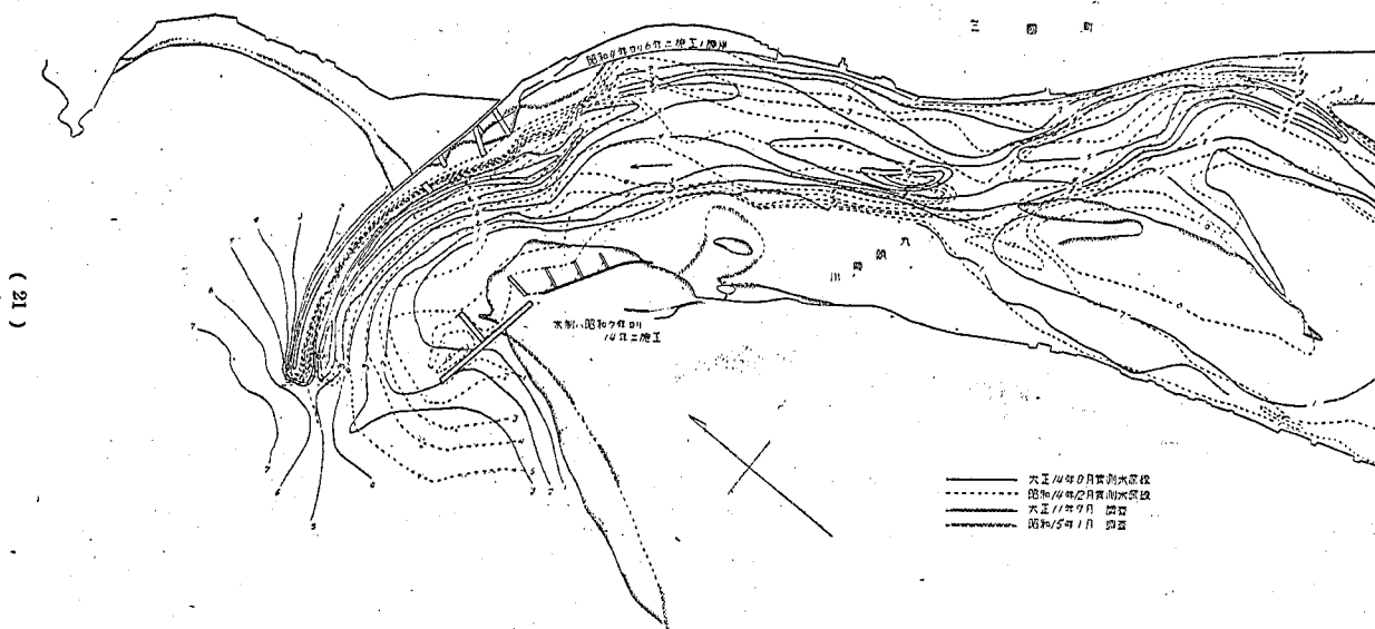
圖—43 九 頭 龍 川 河 口 (縮尺 1/12,000)
