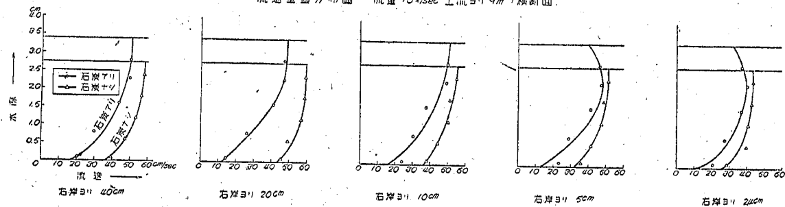
流速垂直分布圖 流量 10 l/sec 上流ヨリ 9m 1 横断面
