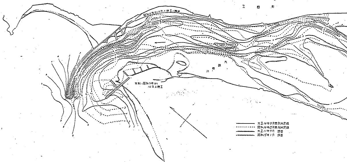
圖—43 九 頭 龍 川 河 口 (縮尺 1/12,000)
