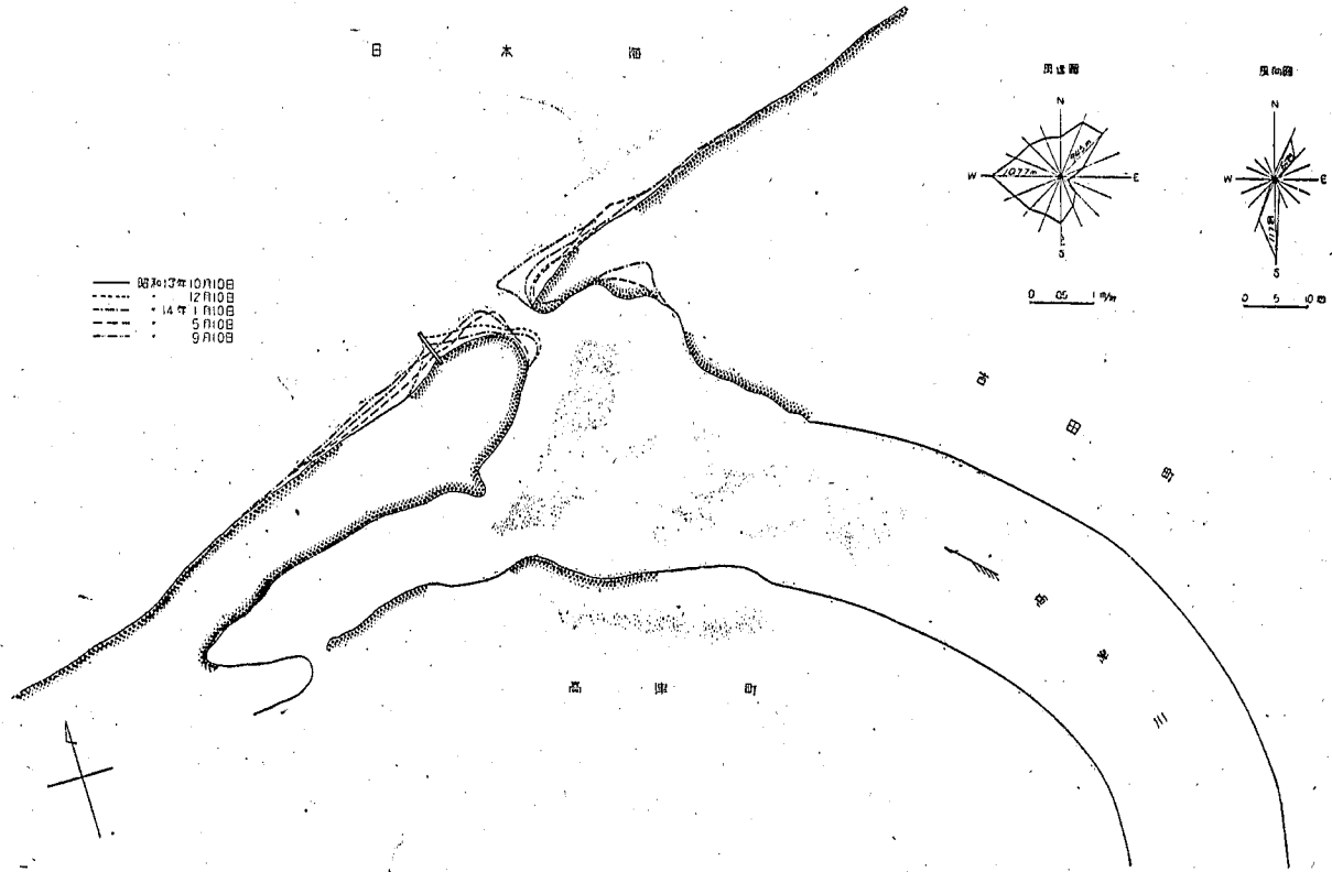
圖—47 高 津 川 河 口 圖 (縮尺 1/9,500)
