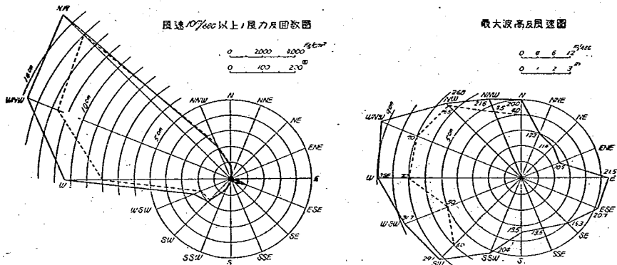
圖-31 浜田港風圖
