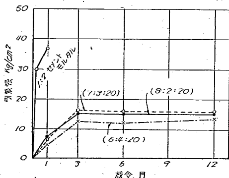
圖-9 玄武土・石灰混合物の引張強に及ぼす材齢の影響
