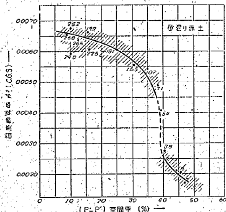
図-8 赤土(砂質赤土)温度伝導率 \lambda^2 ~ 空隙率 関係
