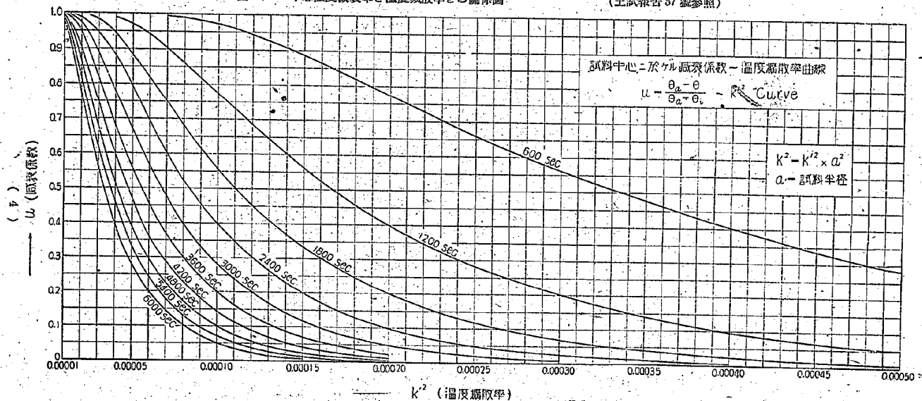
圖-1 中心温度減衰率と温度濕散率との關係圖
