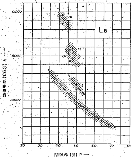
圖-5 (b) 熱傳導度 \lambda と空隙率 P との關係
