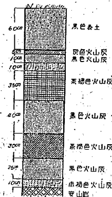
図—20 横岳附近の地層見取図
