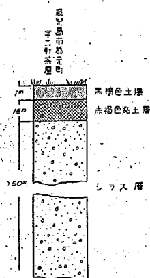
圖—3 シラス層見取圖—(2)
