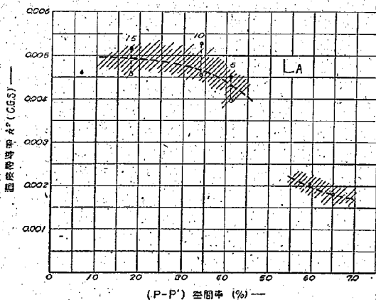
圖-4 (a) 温度傳導率 k^2 と空隙率 ( P-P' ) との關係
