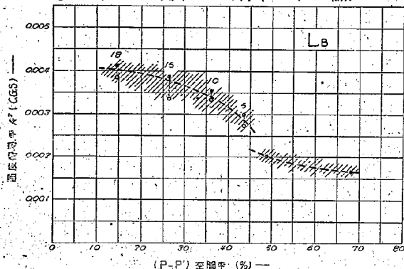
圖-5 (b) 熱傳導度 \lambda と空隙率 P との關係
