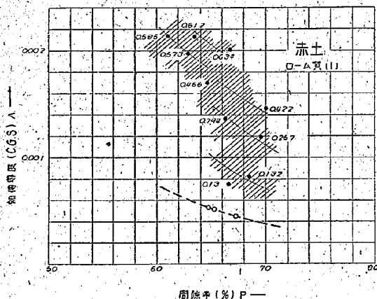
圖-9 ローム質赤熱傳導度 ( \lambda ) と空隙率 P との關係
