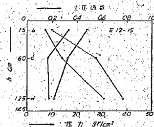
図-25 振動による静土圧の増加 (試験E)
