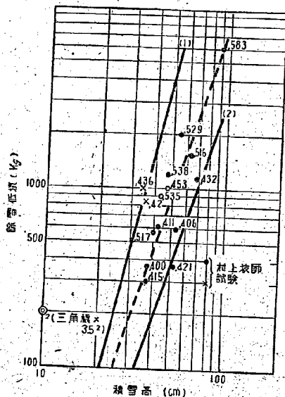
圖-8 前鋤型除雪車の除雪抵抗
