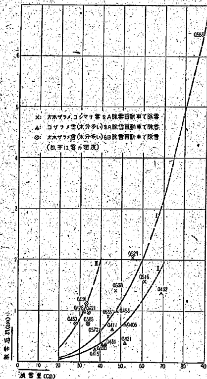
図-15 積雪量と除雪抵抗
