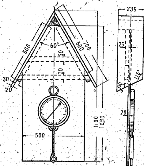
図-6 三角櫓
