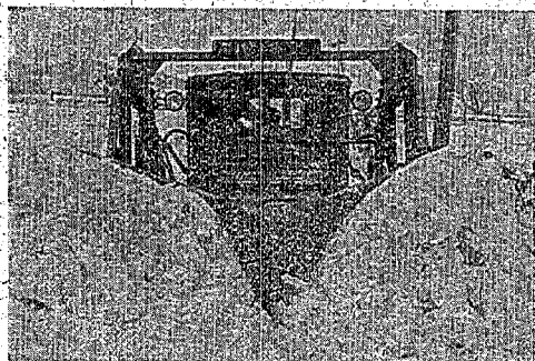
圖一6 走行路(8)に入らんとしてゐる人除雪自動車、積雪 70 cm
