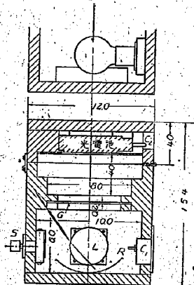
圖-1 測定器の構造
