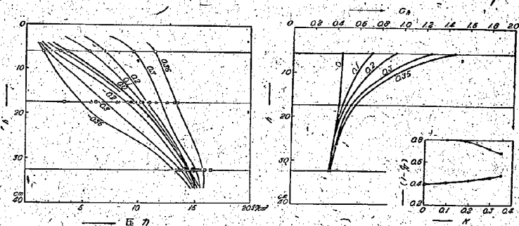
圖-8 固定支點 H=30 cm の第1回最初の振動
