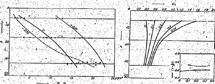
図-13 同上第2回目の振動
