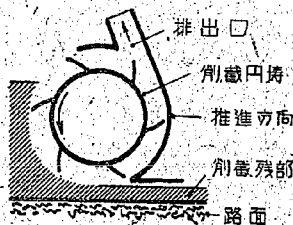
寫眞-8 削地除雪車(II-2型除雪機構)
