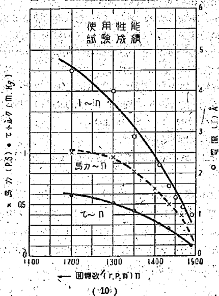
圖-10 使用電動機性能試験成績 (a)
