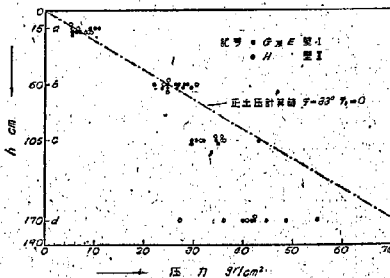
図-25 振動による静土圧の増加 (試験E)
