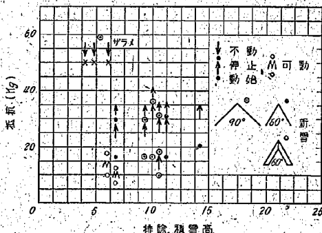
圖-7 三角櫓の推進抵抗
