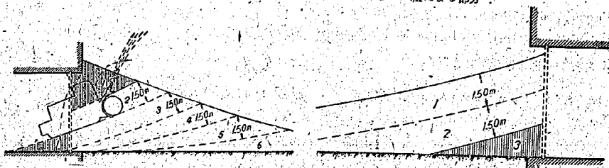
圖—5 隧道出入口に於ける除雪説明圖
