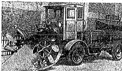
(2) Sno-flyer 回轉除雪車(II-1型除雪機構)
