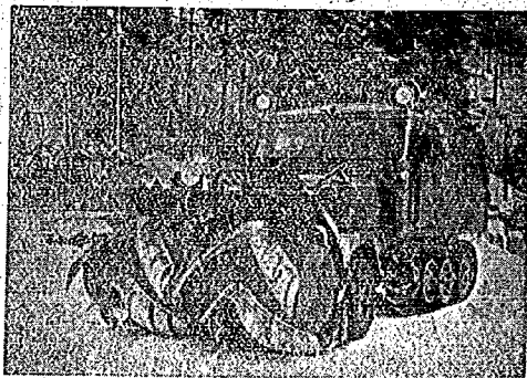
寫眞-8 削地除雪車(II-2型除雪機構)
