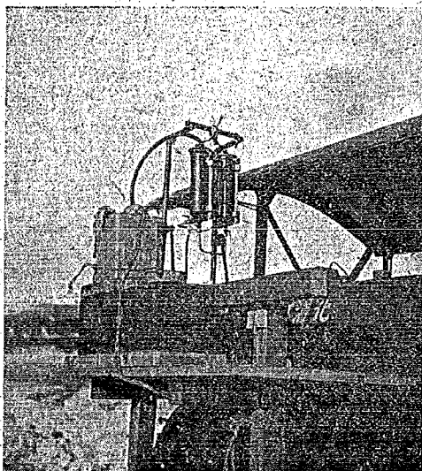
圖—4 B除雪自動車の燃料消費測定器
