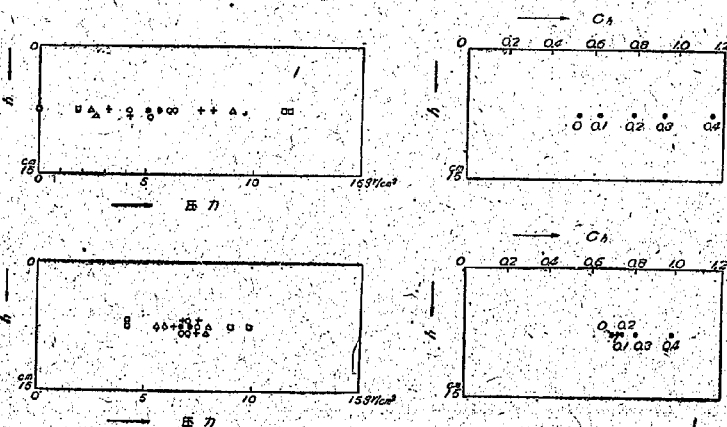
図-10 固定支點 H=15 cm の試験結果
