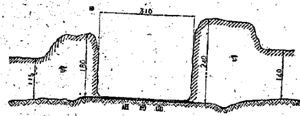
圖一11 走行路(8)の圖一10と同じ箇所の断面圖
