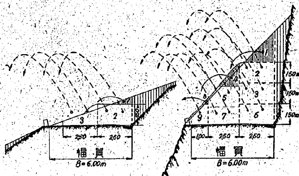
圖-4 除雪作業説明圖
