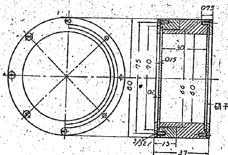
圖-3 試料器の構造
