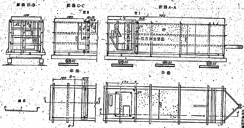
圖-15 大型振動函
