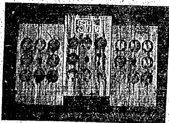
圖-16 5H 9 の破壊状況
