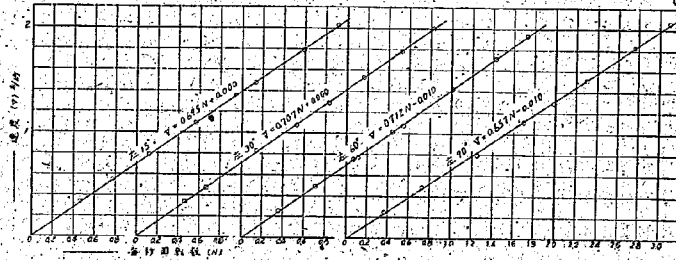
図-11 同上 前上り及び前下りの場合の係數
