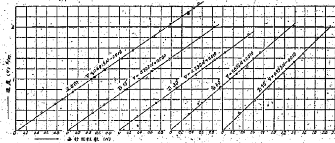
図-10 同上 左に傾けた場合の係數
