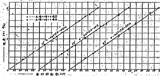
図-12 同上 支持棒を左右横に傾けた場合の係數
