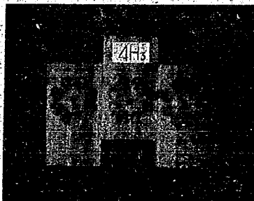
圖-10 4Hの破壊状況
