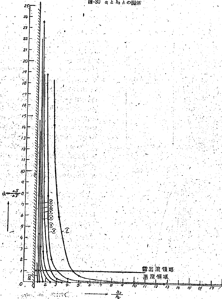
図-30 \alpha と h_2 との関係
