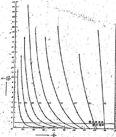
図-22 \beta と h_0 との関係
