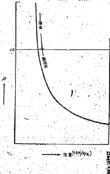
圖-39 \beta と流量との関係
