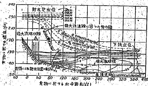
圖-21 Madden Dam の傾斜水叩の實驗
