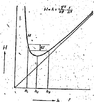
図-13 H と h との関係
