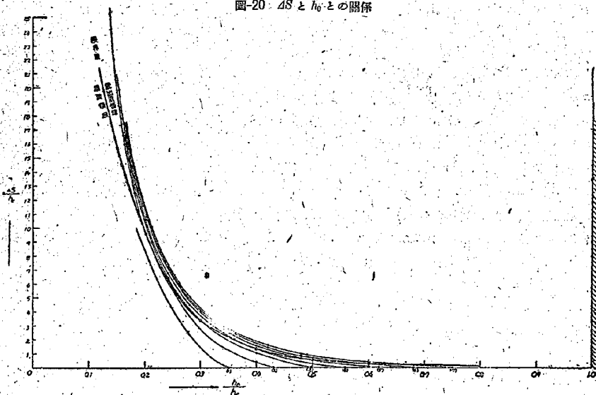
圖-20 \Delta S と h_0 との關係
