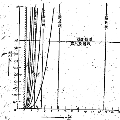
圖-32 \gamma と h_2 との関係
