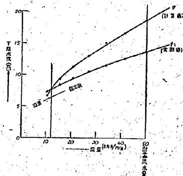
図-47 h_2 , h_2' と流量との関係
