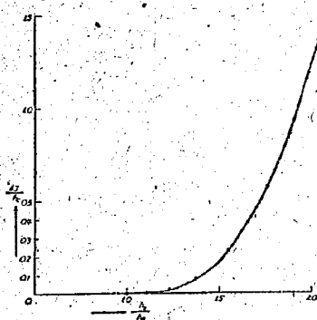
図-16 \Delta J と h_2 との関係
