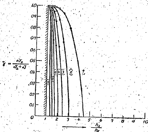
圖-32 \gamma と h_2 との関係
