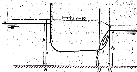
圖-41 水平固定床土上の完全跳水
