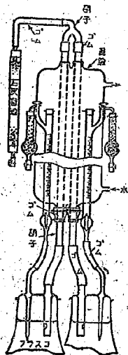
圖-1 遊離石灰滴定装置(略圖)
