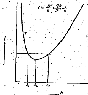
図-12 I と h との関係
