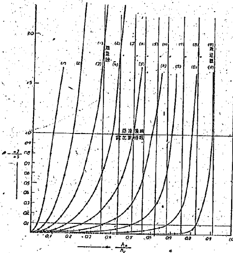
図-22 \beta と h_0 との関係
