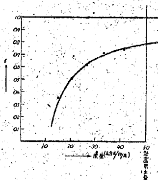
図-53 \gamma と q との關係
