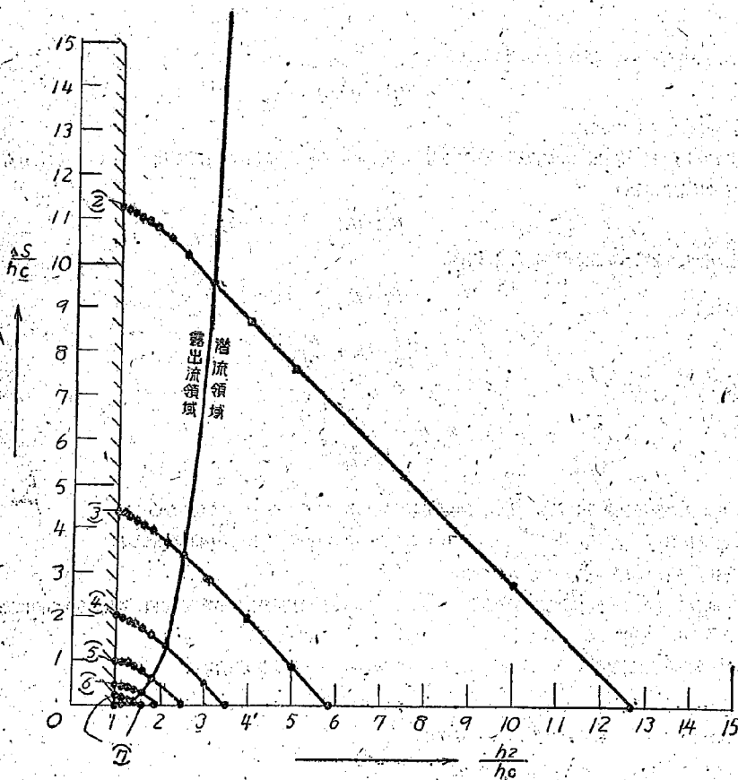
図-29 \Delta S と h_2 との関係
