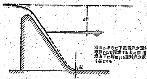
図-4 潜流の場合の虚射流水深 h_1
