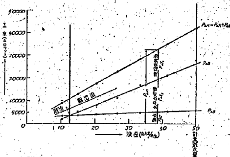
図-50 P_{\Delta H} , P_{\Delta S} , P_{\Delta J} と流量との関係
