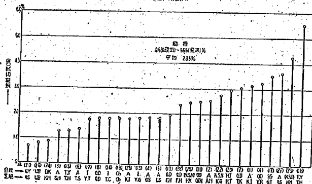
図-3 セメントの遊離石灰量 % (会社, 工場別)
