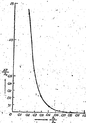
図-17 \Delta J と \frac{h_1}{h_2} との関係
