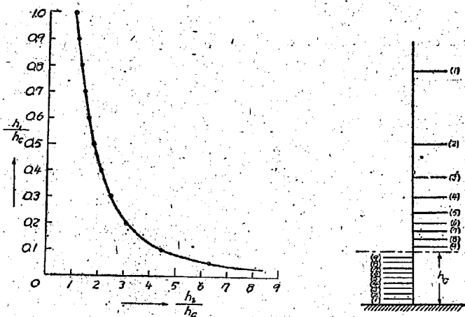
圖-14 h_1 と h_2 との關係
