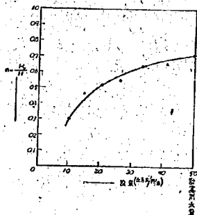
図-49 \eta と流量との関係
