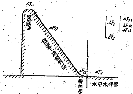
図-4 潜流の場合の虚射流水深 h_1
