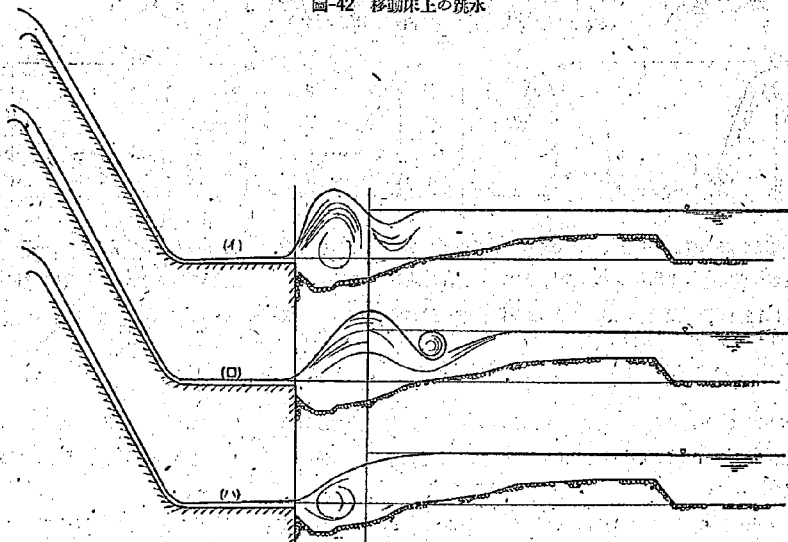
図-42 移動床上の跳水
