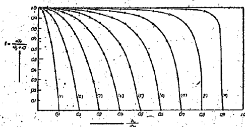
図-23 \gamma と h_0 との関係
