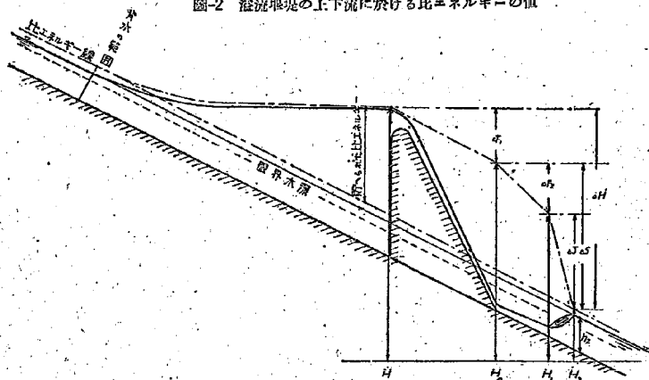
圖-2 溢流堰堤の上下流に於ける比エネルギーの値
