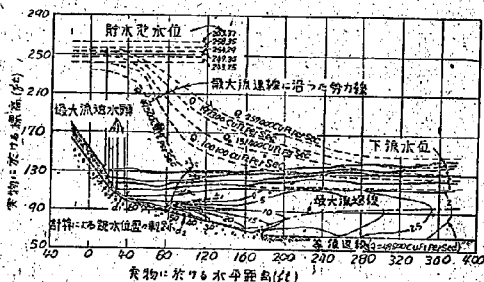
圖-21 Madden Dam の傾斜水叩の實驗
