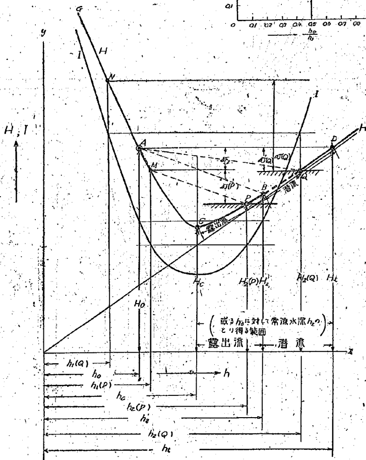
図-28 h_0 一定, h_2 變數とした場合の潜流, 限界流, 露出流
