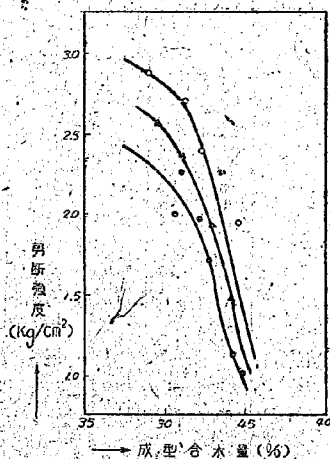
圖-6 褐色土, 成型壓力 2.5 \text{ kg/cm}^2
