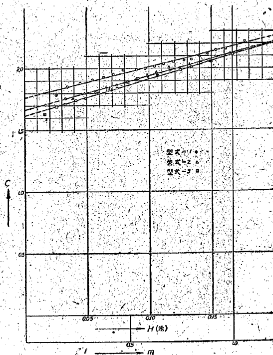
圖-10 溢流深と溢流係數との關係
