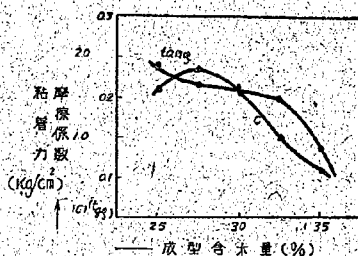
圖-14 紅土, 成型壓力 10 kg/cm 2
