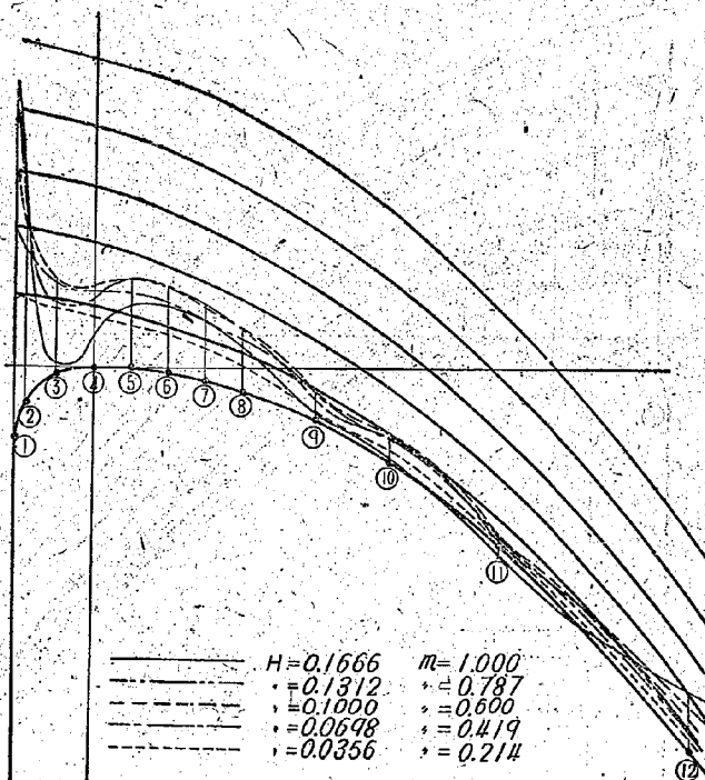
図-12 型式-1 徑間中央に於ける水脈横斷形状及堤頂面の受ける静水圧
