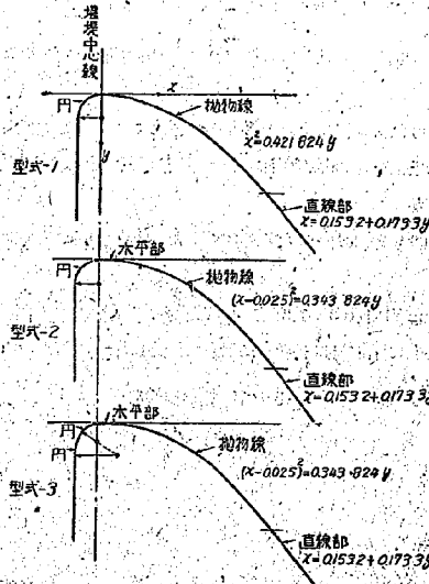
図-2 複型堤頂部縦断形状
