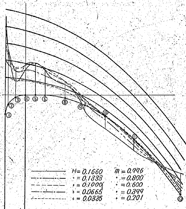
圖-13 型式-2 徑間中央に於ける水脈縦斷形狀及堤頂面の受ける靜水壓
