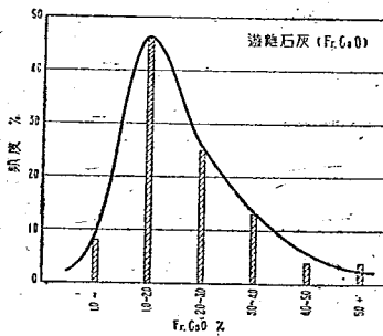
図-2 (5) Fr.CaO 含有量～頻度図
