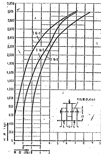
圖-18 竹ボルトと鉄ボルトの試験後の彎曲の差異
