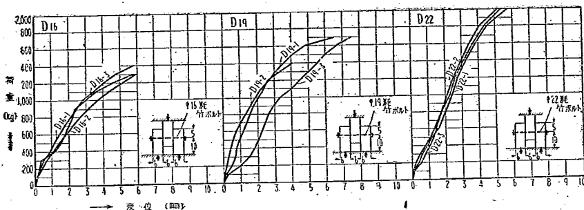
D-類の荷重-変位曲線
