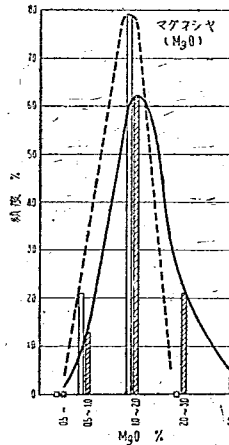
図-2 (6) MgO 含有量～頻度図
