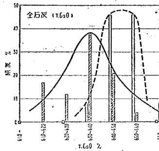
図-2 (4) T.CaO 含有量～頻度図
