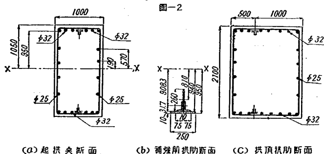
(a) 起拱肋断面
