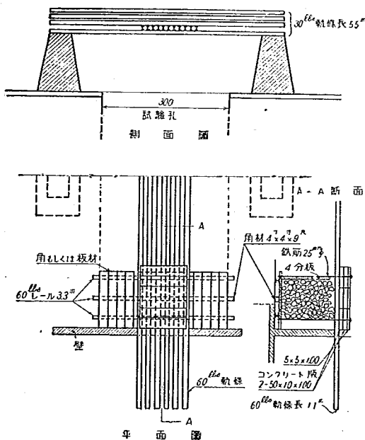
圖一 荷重配置圖
