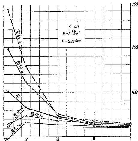
圖-25 (a) フロー量比較圖
