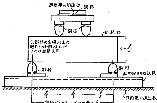
3等分中央荷重法によるコンクリートの曲げ試験装置の1例
