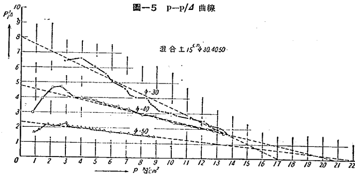
圖-5 p-p/A 曲線
