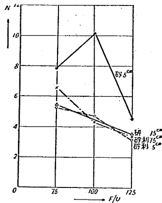
圖-8 N-F/U 曲線
