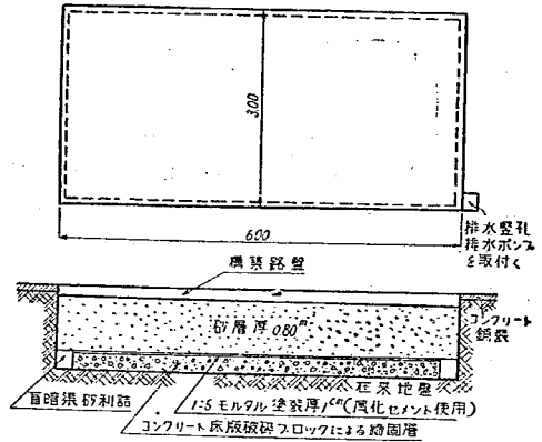
圖-2 基礎構造
