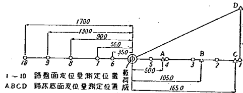
圖-3 ダイヤルゲージ配置圖
