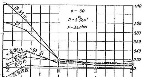
圖-25(b) フロー量比較圖
