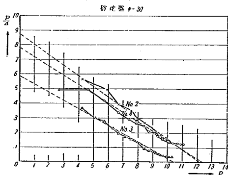
圖-4 p-p/A 曲線, \frac{p}{A} = Mp + N (直線と假定した場合)
