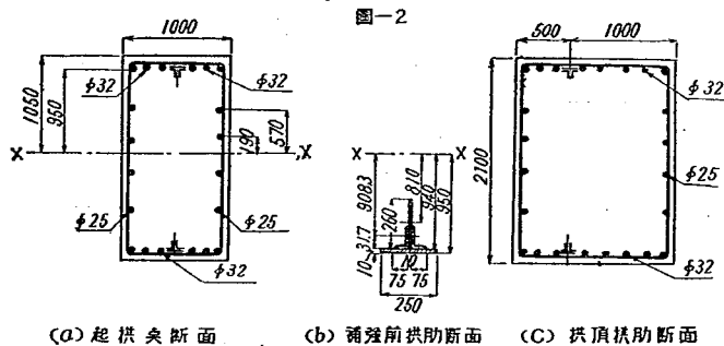
(a) 起拱肋斷面
