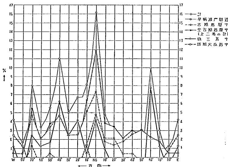
圖-7 解析前斷層頻度圖
