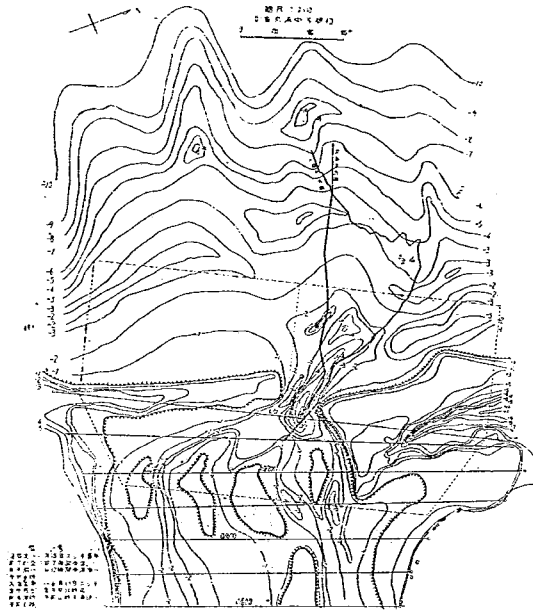
図-16 川内川河口平面並退入潮流方向圖
