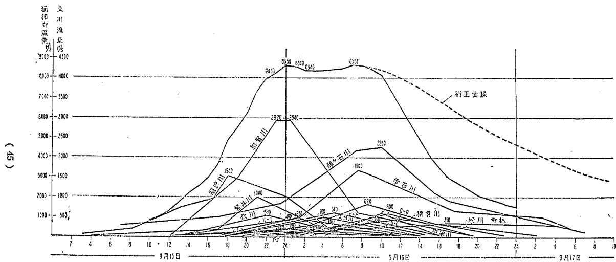
圖-31 北上川狐禪寺洪水流量曲線
