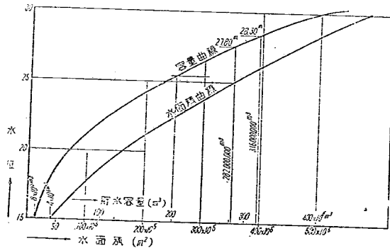
図-33 一ノ關平時水面積曲線及容量曲線
