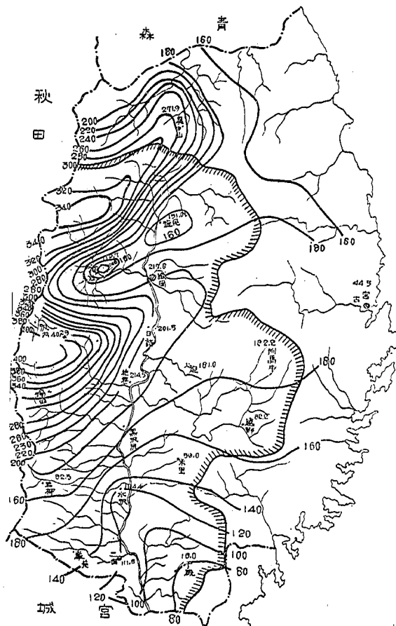
圖-53 (D) 北上川上流域連日雨量分布圖(昭和 22 年 7 月 29 日~8 月 4 日)
