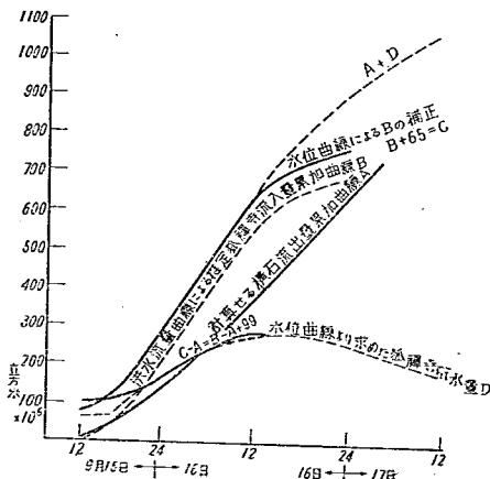
圖-34 狹禪寺洪水流量補正曲線
