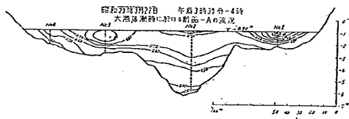
圖-22 流速分布圖
