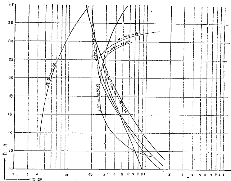
図-51 狭窄部に於ける水面勾配
