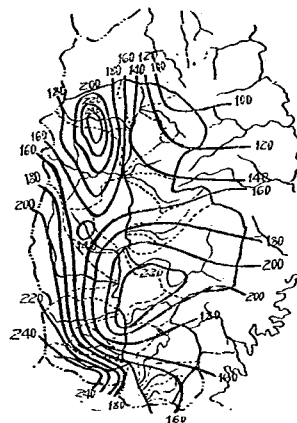
図-16 昭和 22. 6. 12~15 日 4日連続雨量分布圖
