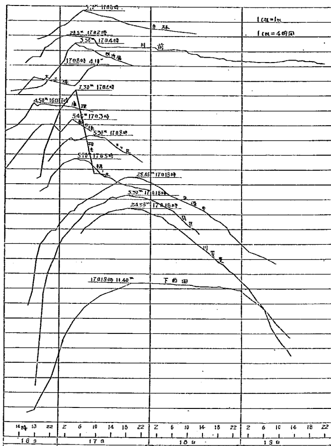
図-44 (イ) 北上川本川水位曲線 昭和23年9月洪水(アイオン颱風)
