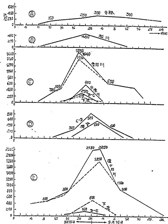
図-29 北上川本川及支川合流点洪水流量曲線 (カザリン洪水)
