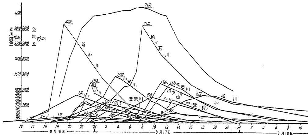
圖-48 昭和23年9月洪水 利根川洪水流量曲線
