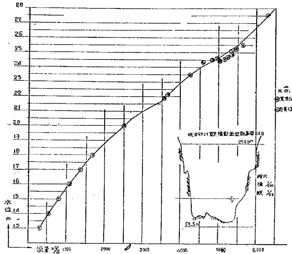
図-52 狹部水位相当流量
