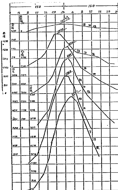
圖-30 北上川洪水流量曲線
