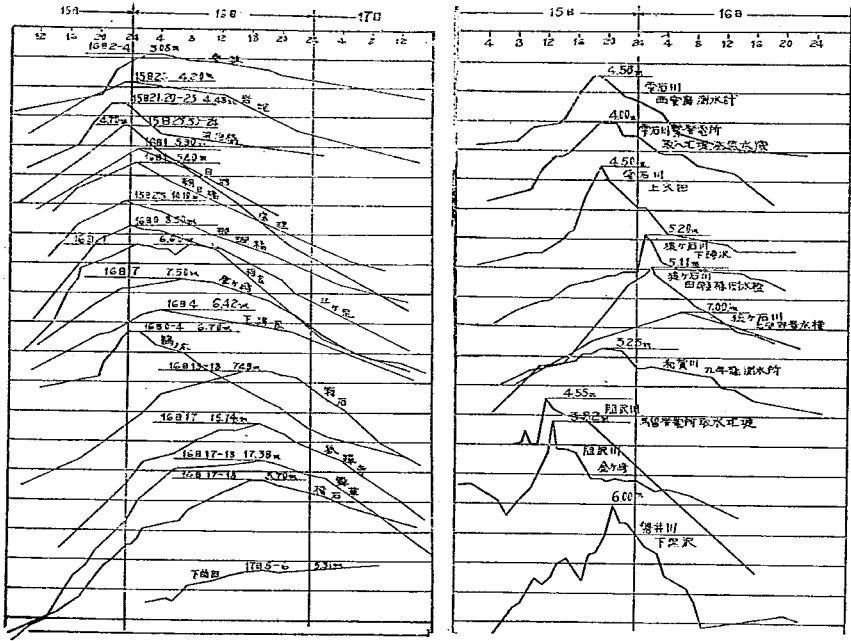
図-18 北上川支川高水位曲線 昭和 22. 9 (カザリン颱風時)
