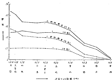
図-15 潮波振幅の減衰状態
