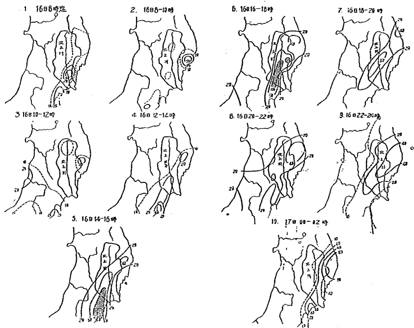
圖-43 北上川上流域 2時間雨量分布圖
