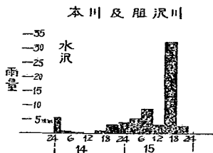
図-17 北上川流域カザリン颱風洪水に伴う時間雨量 (昭 22. 9)
