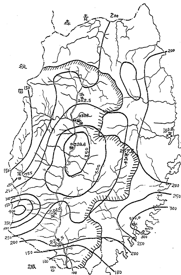
圖-53 (C) 北上川上流域連日雨量分布圖(大正 9 年 8 月 5~12 日)
