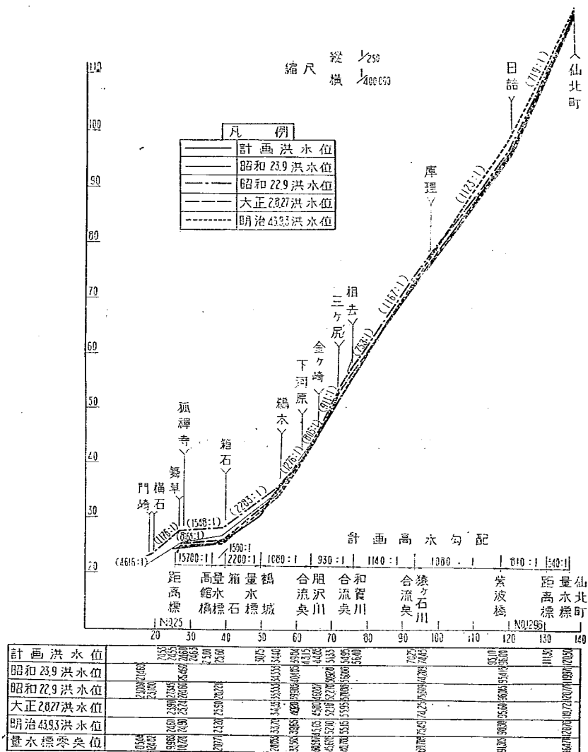
圖-20 北上川最高水位縦断面圖
