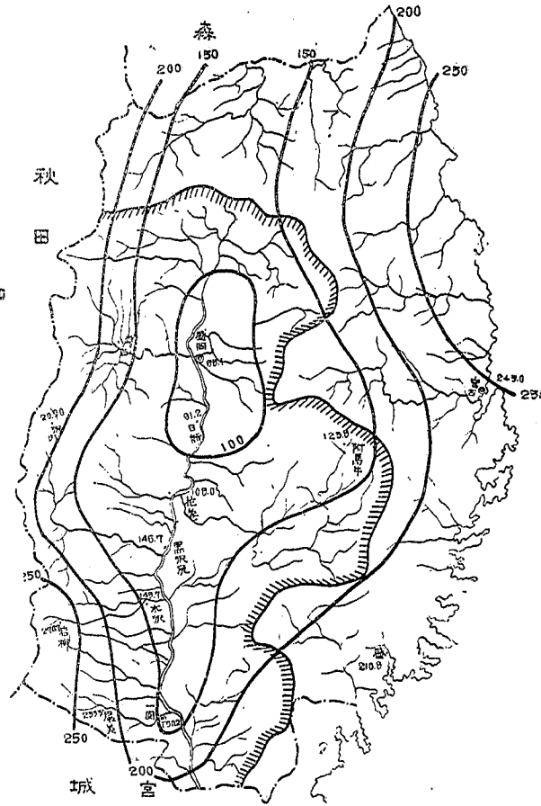
圖-53 (B) 北上川上流連綿雨量分布圖 (大正 2 年 8 月 25~29 日)
