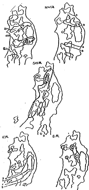
図-6 各風向による収斂域の位置
