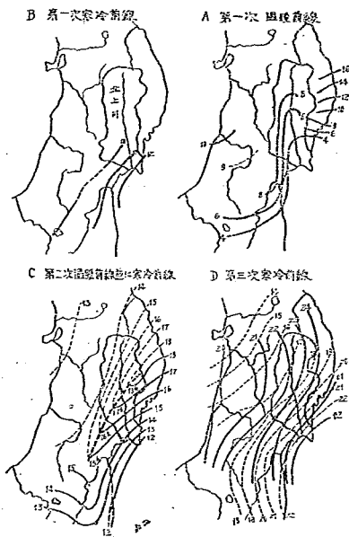
図-39 前線移動状況
