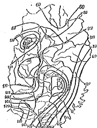
図-13 昭和 22. 9. 14 日雨量分布圖
