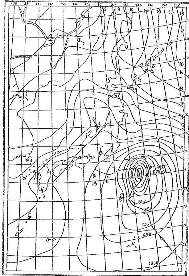
圖-35 昭和 23 年 8 月 13 日 15 時天氣圖
