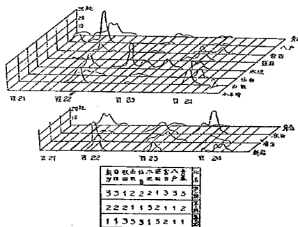
圖-9 各地降水の變化
