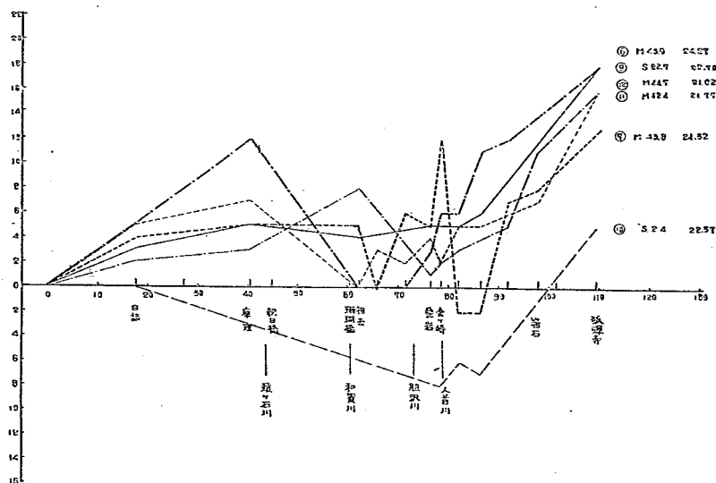
図-54 (B) 北上川上流域本川出水時間
