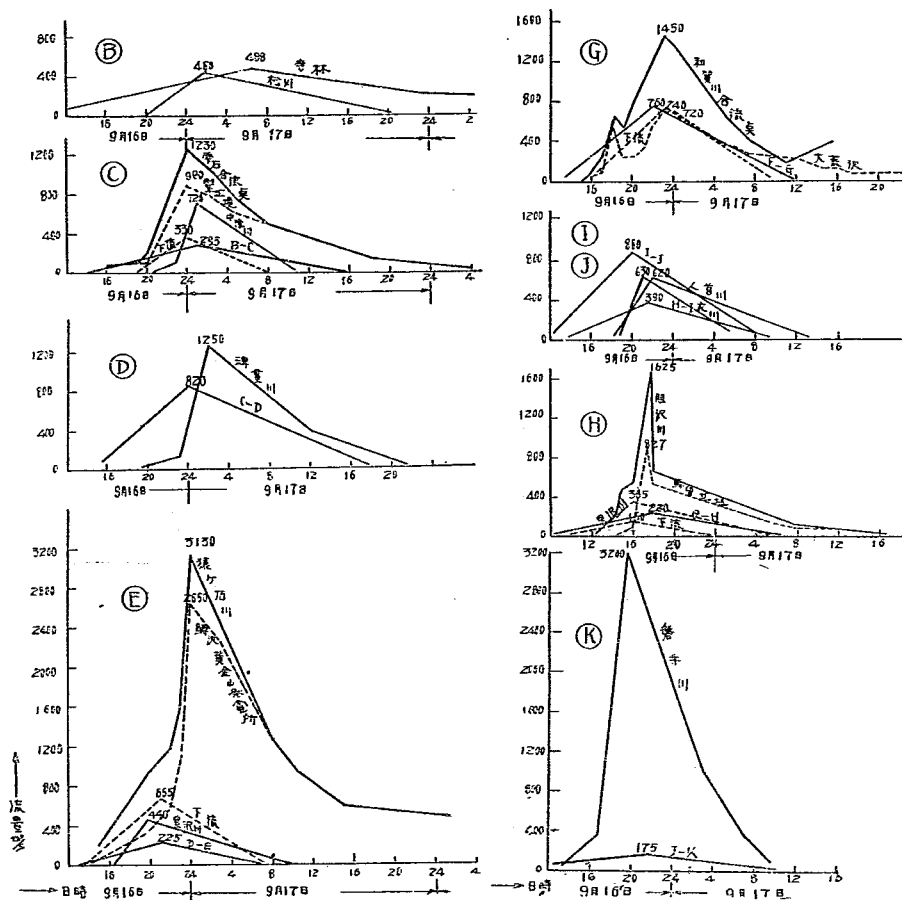
図-47 北上川本川支川合流点洪水流量曲線
