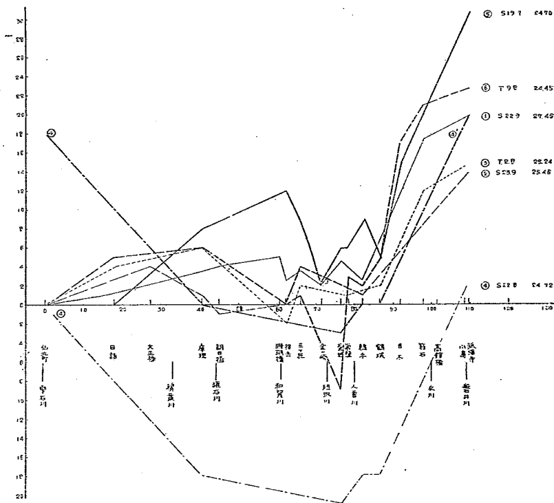
圖—54 (A) 北上川上流域本川出水時間
