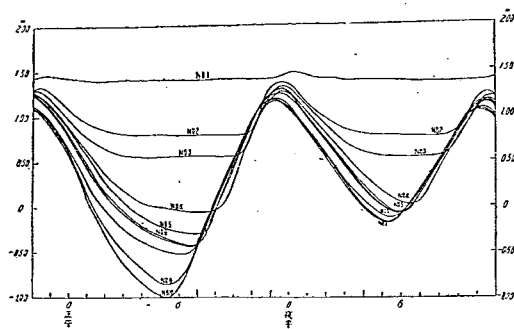
図-11 大潮時に於ける水位圖 (昭和 23 年 5 月 25 日) 基準面東京灣中等潮位
