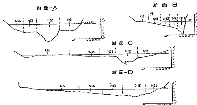
圖-17 流量實測断面圖
