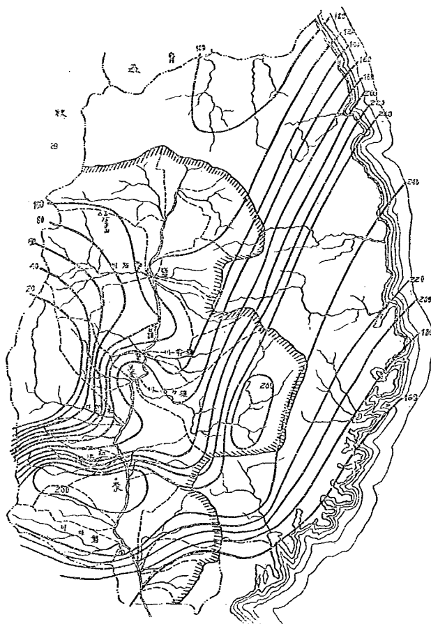
図-41 昭和 23. 9. 16 日 (アイオン颱風) 北上川上流域雨量分布図
