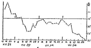
圖-8(A) 雨域中心の移動
