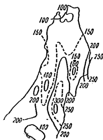
圖-4 東北地方最大日雨量分布圖
