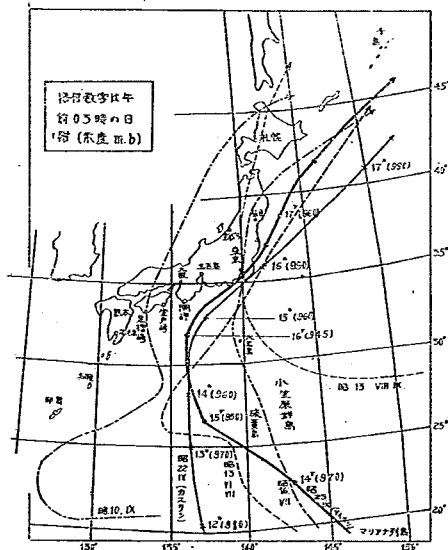
圖-12 カザリン颱風経路圖(昭和 22. 9. 10~18) アイオン颱風経路圖(昭和 23. 9. 10~19)
