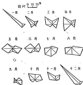
図-2 限之城風向圖 (昭和 15~19 年別月合計)
