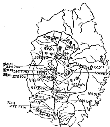
圖-3 北上川支流流域平均高度
