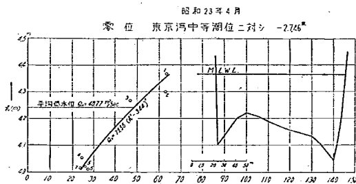
圖-25 荒瀬低水流量曲線
