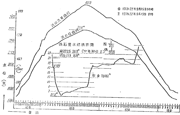
図-32 横石壺水深洪水水位及洪水流量曲線
