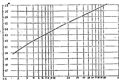
圖—56 狐禪寺確率洪水位
