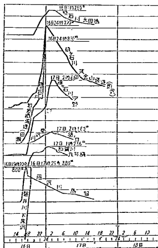
図-44 (ロ) 北上川各支川水位曲線 (アイオン台風)
