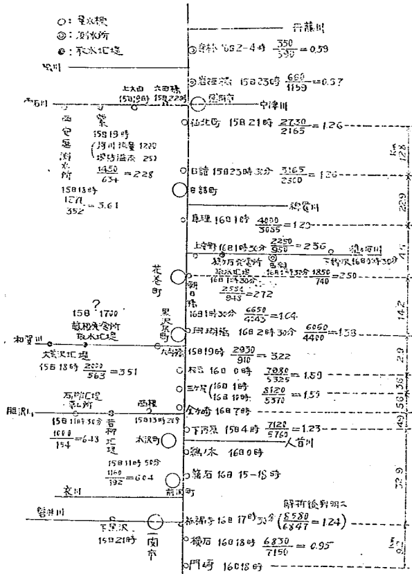
図-21 観測最大流量及时刻圖 (昭 22. 9)
