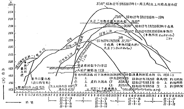
図-19 北上川狐禪寺洪水曲線
