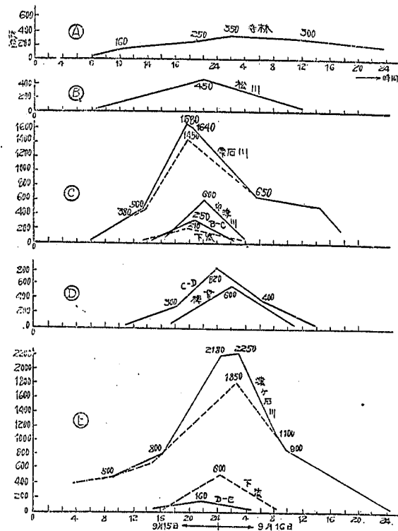
圖-29 北上川本川及支川合流點洪水流量曲線 (カザリン洪水)
