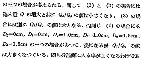
る。(2)の場合にも D_0=1.0\text{cm} , D_1=0.0\text{cm} , D_2=1.5\text{cm} , D_3=0.0\text{cm} の二つの場合があるが、前者の方が後者より小さい Q_1/Q_2 の値を與える。即ち本流側の堰上げ高が分流側のそれに比べて大きい程、つまり本流側の分岐点以後の勾配が分流側のそれよりも緩なる程、分流側に流入する水量が多いわけである。(3)の場合にも D_0=0\text{cm} , D_1=1\text{cm} , D_2=0\text{cm} , D_3=1.5\text{cm} の二通りの場合をあげたが、此の時は本流側の勾配が分流
