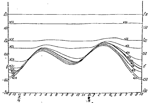
圖-12 小潮時に於ける水位圖 (昭和 23 年 7 月 30~31 日 (月令 23.7)) 基準面東京灣中等水位
