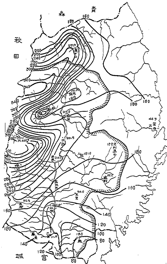
圖-53 (D) 北上川上流域連續分布圖 (昭和 22 年 7 月 29 日~8 月 4 日)
