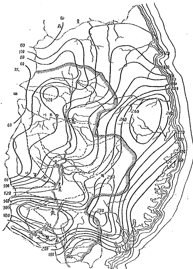
図-42 昭和 23. 9. 15~17 日 (アイオン台風) 北上川上流部雨量分布図
