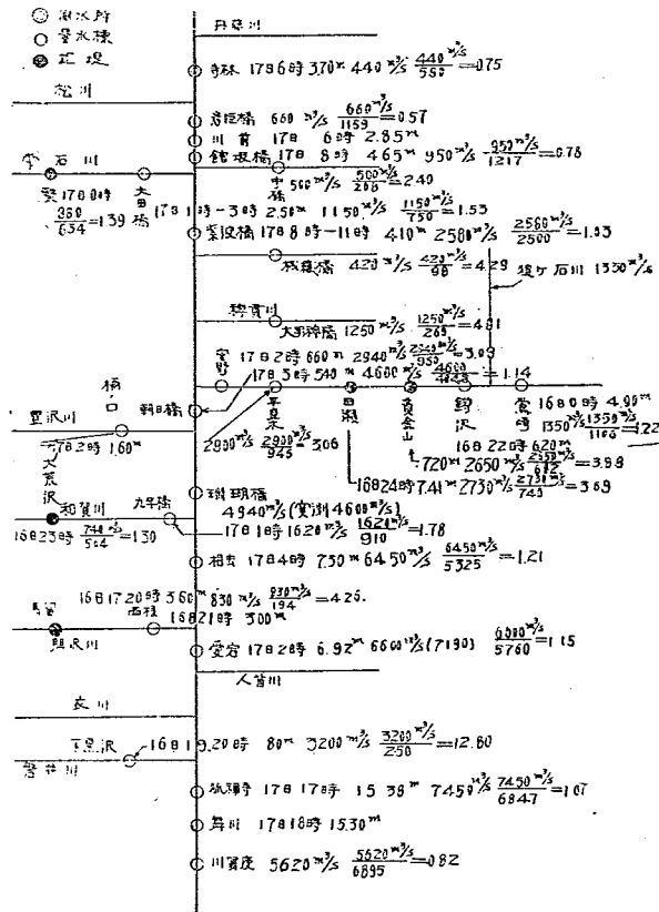
図-45 北上川上流アイオン颱風洪水観測流量 (23. 9)
