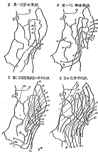
圖-39 前線移動状況
