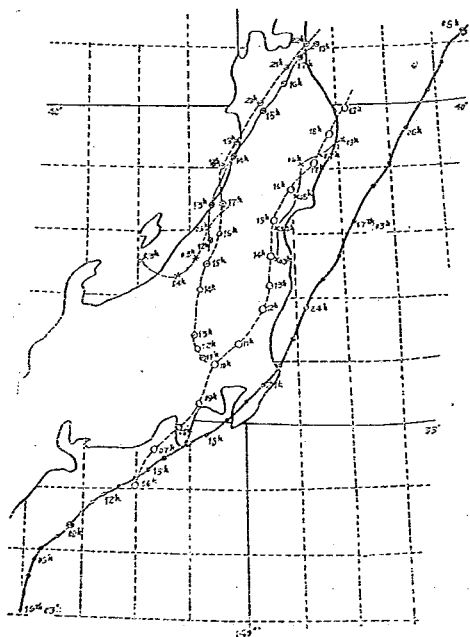
圖-38 颱風の進路並びに低氣壓の進路
