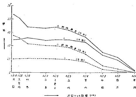
図-15 潮波振幅の減衰状態
