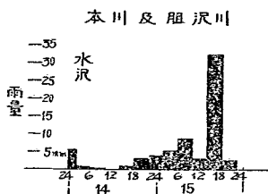
図-17 北上川流域カザリン颱風洪水に伴う時間雨量 (昭 22. 9)
