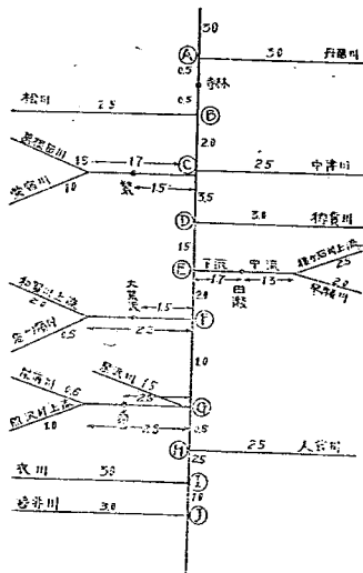
圖-28 洪水到達時間 (單位 hr) 時間流量實測地點
