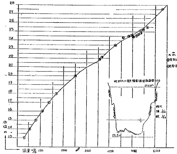
図-52 狹部水位相当流量
