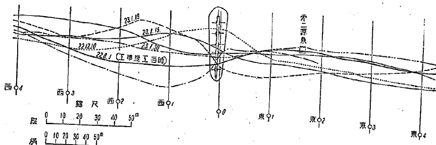
図-14 皆生海岸汀線変化図
