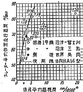
図-5 グレーダ-速度と切刃磨耗量との関係
