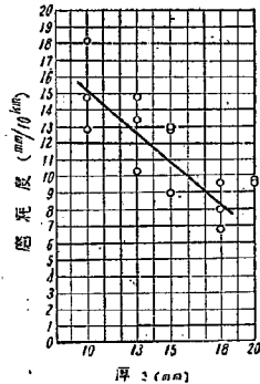
図-6 切刃の厚さと磨耗度 (THA1)
