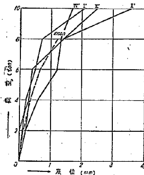
図-12 No. 3 B 系変位曲線
