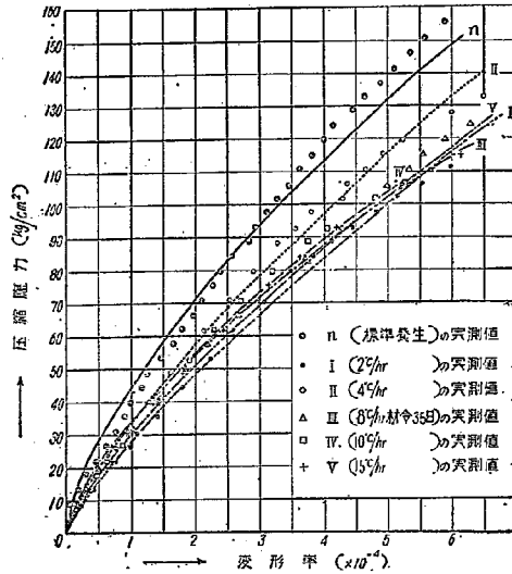
図-14 圧縮に対する変形率 (材令 28 日)
