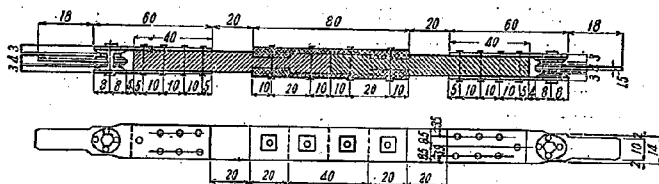
図-2 供試験機取付一般図 (cm 単位)
