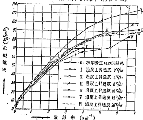
図-13 圧縮に対する変形率 (材令 7 日)
