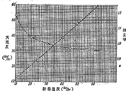
図-5 計器速度
