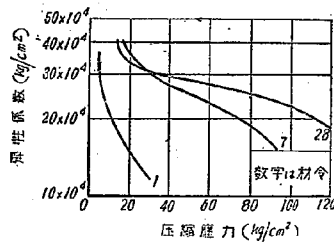
図-21 温度上昇速度毎時 20°C の場合の弾性係数
