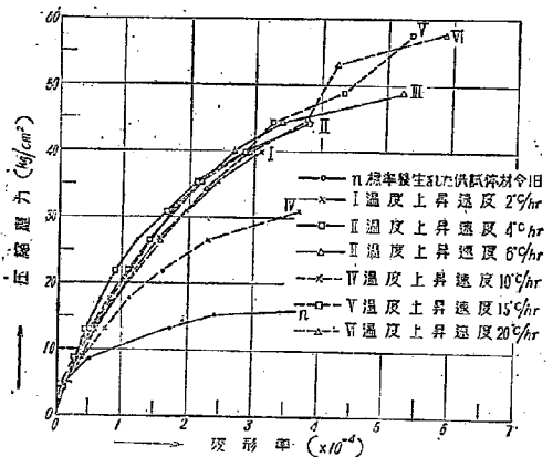
図-12 圧縮に対する変形率 (材令 1 日)
