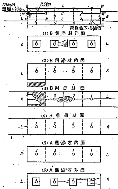
図-5 No.1 供試体破壊状況図
