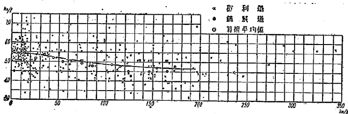
図-11 ペドメーター凹凸回数 (回/km) と走行率 (km/h)
