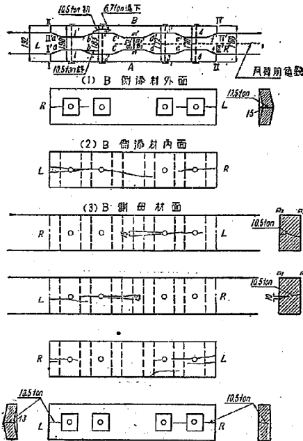
図-14 No.3 供試体破壊状況図
