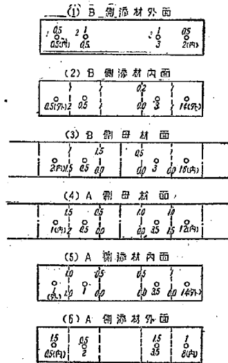
圖-25 No.5 供試体
