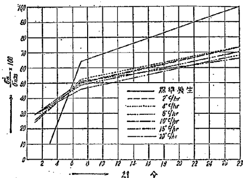
図-10 圧縮強度の比較
