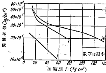
図-19 温度上昇速度毎時 10°C の場合の弾性係数
