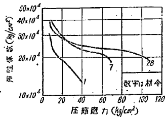
図-16 温度上昇速度毎時 2°C の場合の弾性係数
