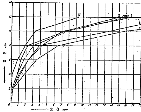
図-16 No. 4 A 系変位曲線
