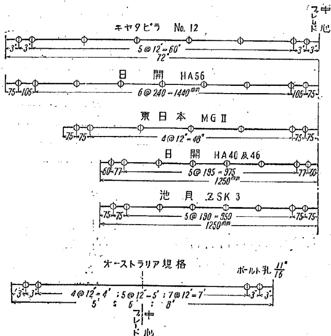
図-1 各種グレーダのブレード・ボルト孔のピッチ
