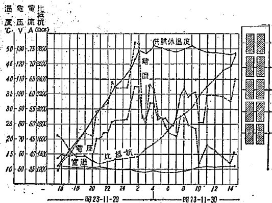
図-5 温度上昇速度毎時 4°C の場合の温度および電氣的経過
