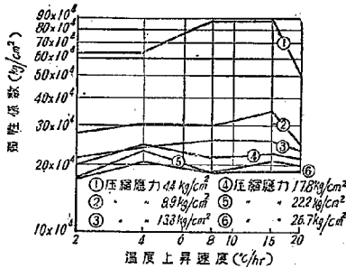
図-22 材令 1 日における温度上昇速度と弾性係数 図-23 材令 7 日における温度上昇速度と弾性係数
