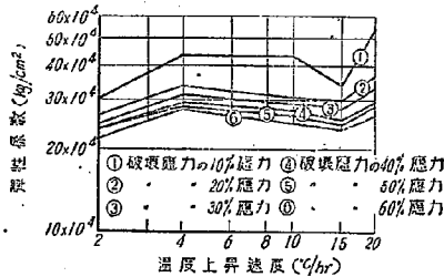
図-24 材令 28 日における温度上昇速度と弾性係数
