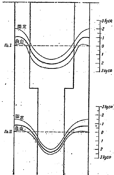
図-34 単位荷重 1 kg に対するボルトの曲げモーメント
