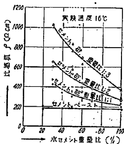
図-1 ペーストおよびモルタルの比抵抗
