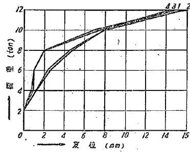
図-18-1 No. 4 C 系変位曲線
