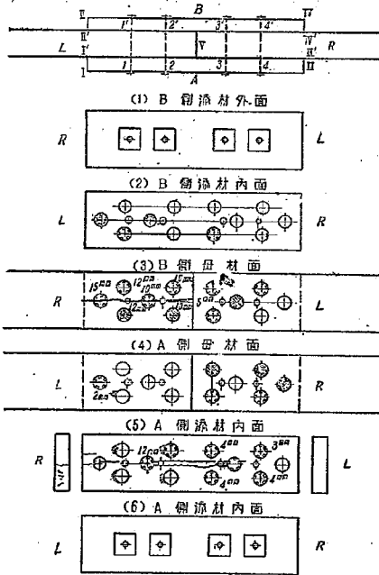
圖-29 No. 6 供試體破壞狀況圖
