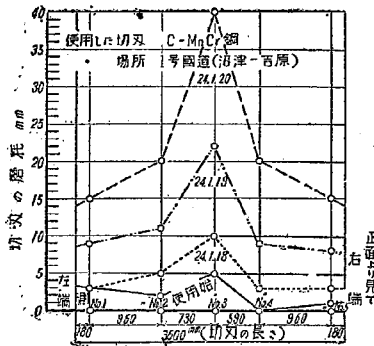
図-2 切刃の磨耗の進む状態 (その 1)
