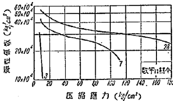
図-15 標準発生をしたコンクリートの弾性係数
