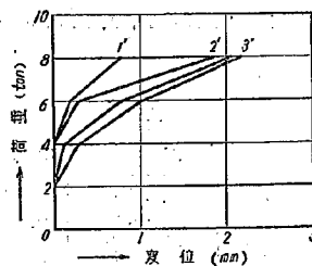
図-13-2 No. 3 C 系変位曲線
