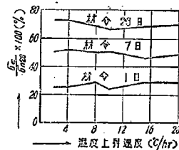
図-11 温度上昇速度と \sigma_c/\sigma_{ns} \times 100 との関係
