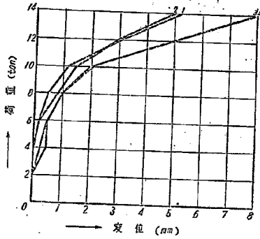
圖-28-1 No. 6 C' 系變位曲線
