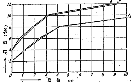
図-18-2 No. 4 C' 系変位曲線
