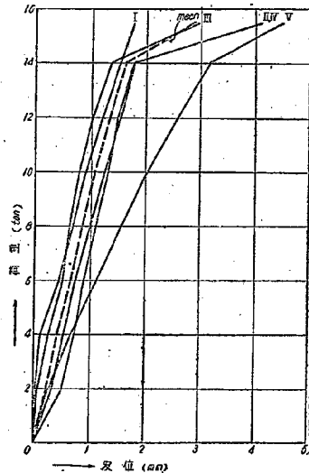
図-4 No.1A 系変位曲線
