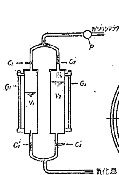
図-3 ガソリン消費量計
