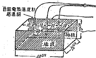
図-3 供 試 体
