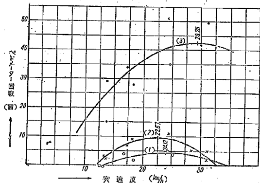
図-7 速度と衝撃係数の関係
