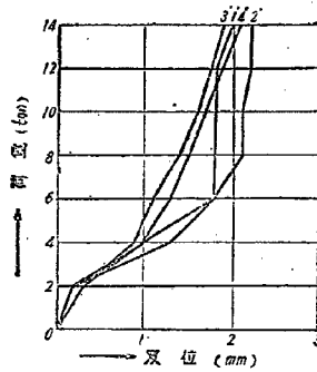
圖 23-2 No.5 C 系変位曲線
