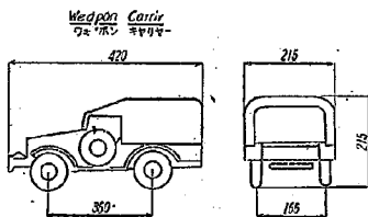
図-2 試験自動車
