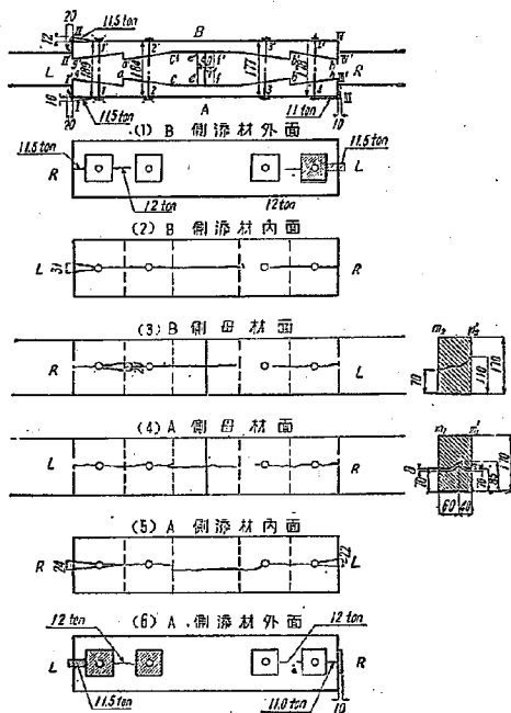
圖-20 No.4 供試体
