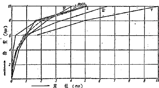
図-11 No. 3 A 系変位曲線
