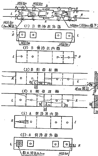
圖-24 No.5 供試体破壊状況図
