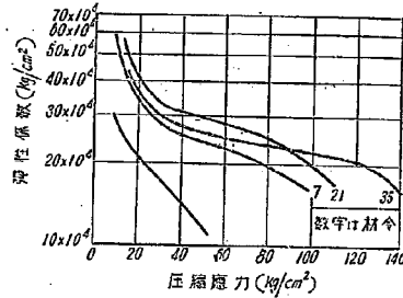
図-18 温度上昇速度毎時 8°C の場合の弾性係数
