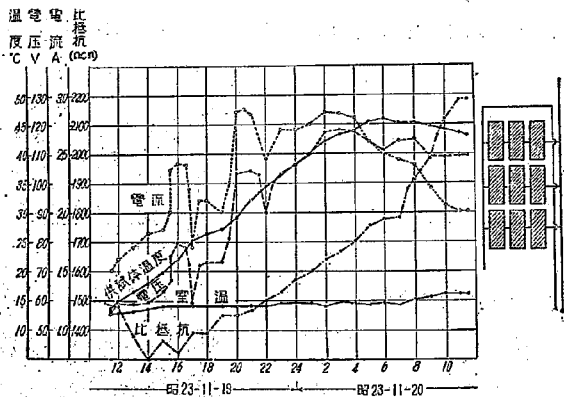
図-4 温度上昇速度毎時 2°C の場合の温度および電氣的経過
