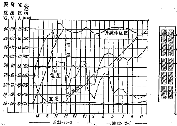
図-6 温度上昇速度毎時 8°C の場合の温度および電気的経過
