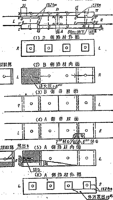
図-9 No. 2 供試体破壊状況図
