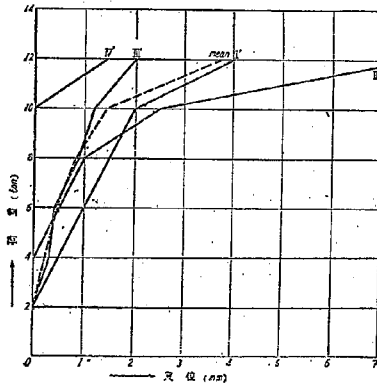
図-17 No. 4 B 系変位曲線
