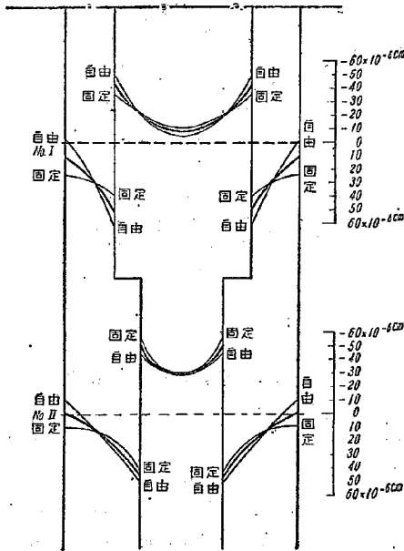
図-33 単位荷重 1 kg に対するボルト変形
