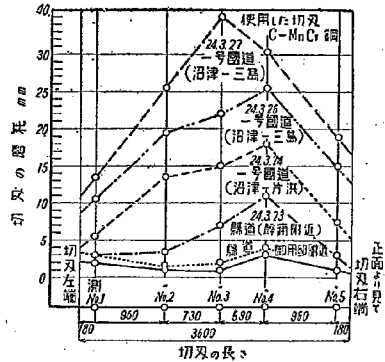
図-3 切刃の磨耗の進む状態 (その 2)
