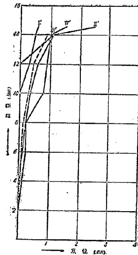
図-22 No.5 B 系変位曲線
