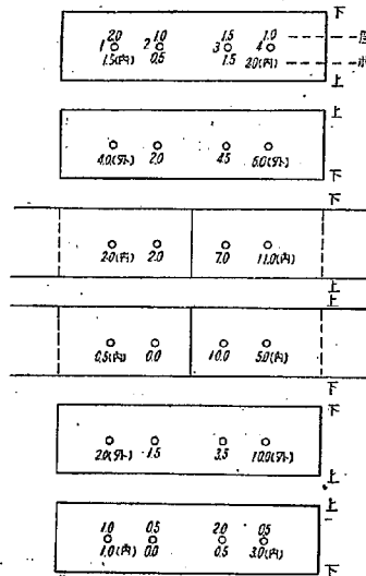
圖-30 No. 6 供試體
