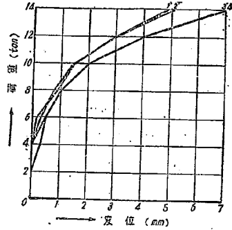
圖-28-2 No. 6 C' 系變位曲線
