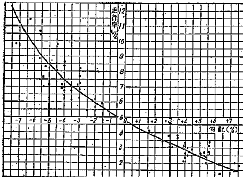
図-10 こう配とガソリン消費量との関係
