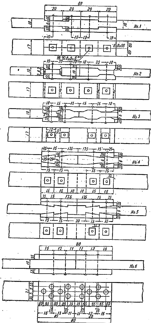
図-1 供試体一般図 (cm 単位)
