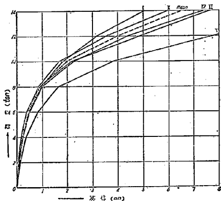
図-26 No.6 A 系変位曲線
