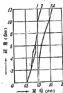
図-8 No. 2 C 系変位曲線
