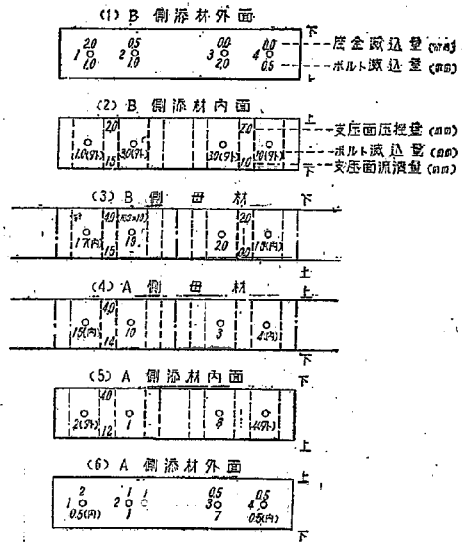
図-15 No.3 供試体
