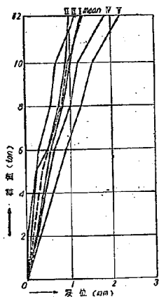
図-6 No. 2 A 系変位曲線
