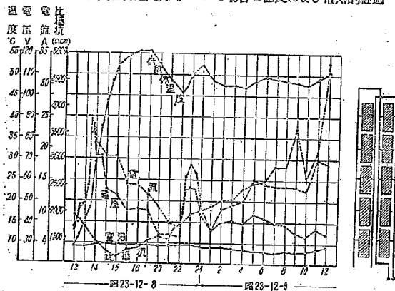
図-7 温度上昇速度毎時 10°C の場合の温度および電気的経過
