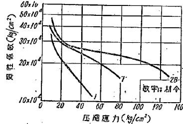
図-20 温度上昇速度毎時 15°C の場合の弾性係数
