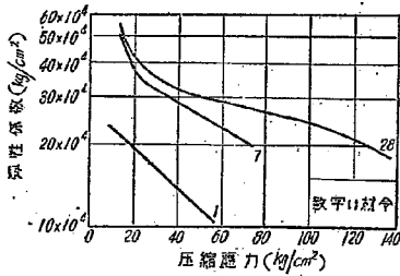
図-17 温度上昇速度毎時 4°C の場合の弾性係数
