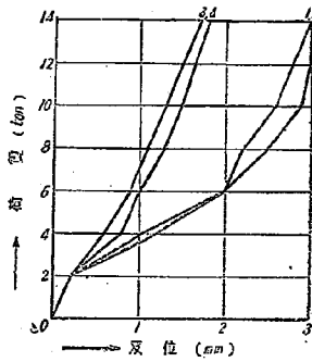
圖-23-1 No.5 C 系変位曲線
