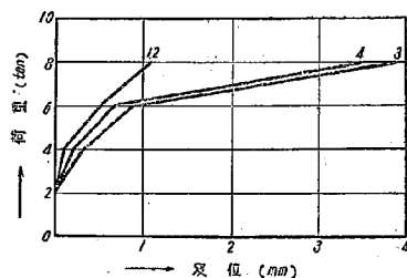
図-13-1 No. 3 C 系変位曲線
