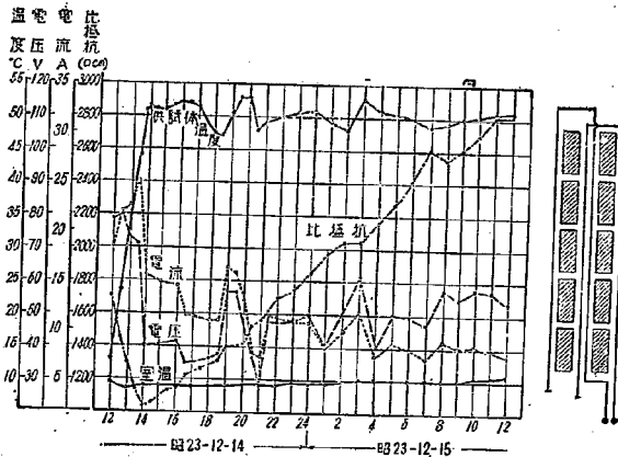
図-8 温度上昇速度毎時 15°C の場合の温度および電気的経過
