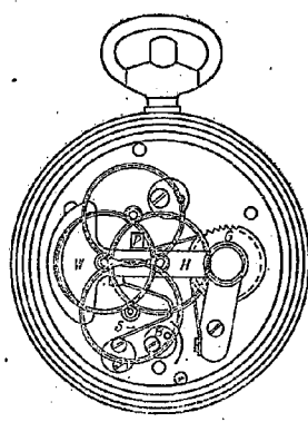
図-4 ペドメーター
