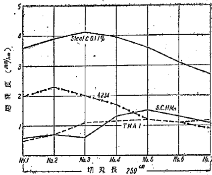
図-4 切刃の磨耗の進む状態 (その 3 小型機)
