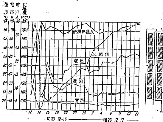
図-9 温度上昇速度毎時 20°C の場合の温度および電気的経過
