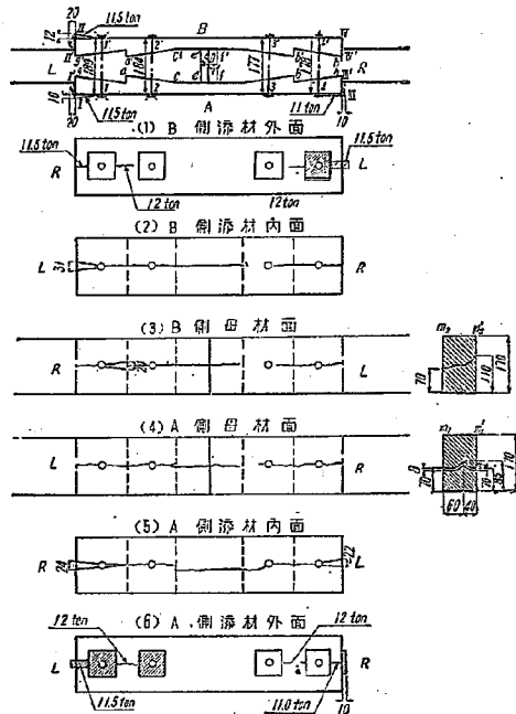
図-20 No.4 供試体
