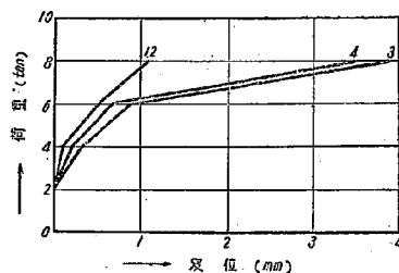
図-13-1 No. 3 C 系変位曲線
