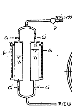
図-3 ガソリン消費量計
