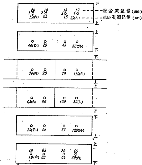
圖-30 No.6 供試體
