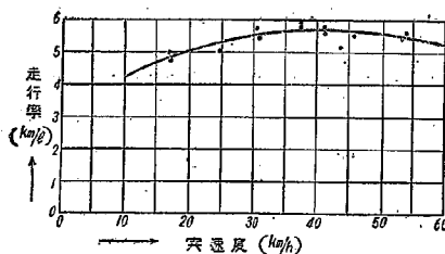
図-6 速度と燃料消費の関係
