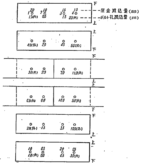
圖-30 No.6 供試體
