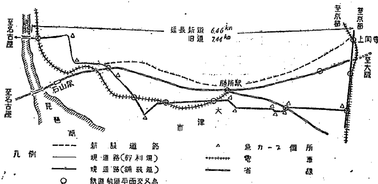
图-12 大津国道新旧比较图
