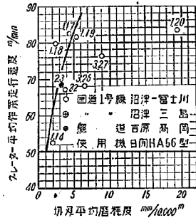
図-5 グレーダー速度と切刃磨耗度との関係
