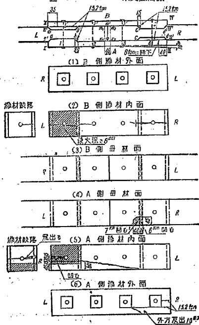
図-9 No. 2 供試体破壊状況図
