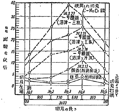
図-3 切刃の磨耗の進む状態 (その 2)
