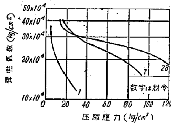
図-21 温度上昇速度毎時 20°C の場合の弾性係数
