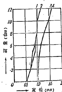
図-8 No. 2 C 系変位曲線
