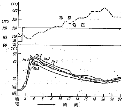
図-12 III 型の温度および電気的経過
