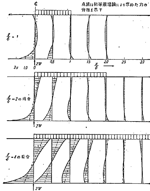
図-9 \frac{\pi b}{2W} N_x(x, y) の分布
