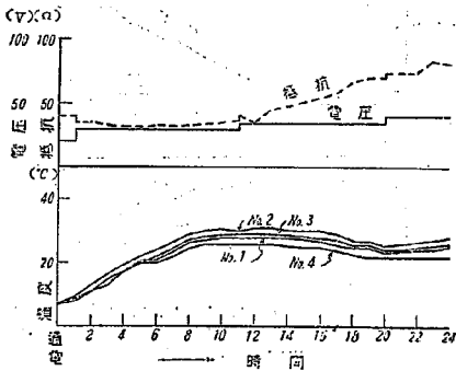
図-16 VII 型の温度および電気的経過
