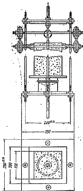
図-18 引抜試験装置
