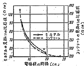
図-8 電極板の間隔を変えた場合のモルタルおよびコンクリートの見掛けの比抵抗
