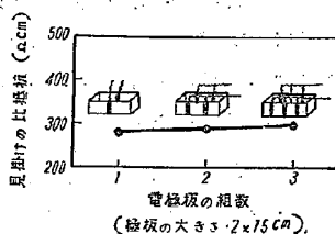
図-2 電極板の組数と見掛けの比抵抗との関係
