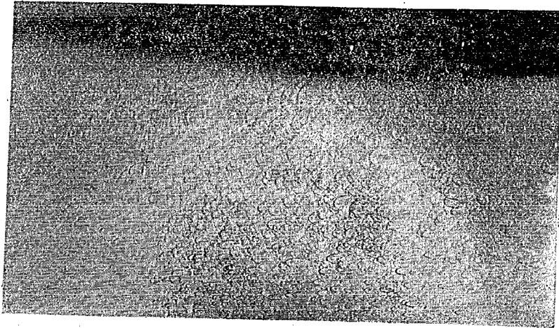
F. Ahlborn によつて撮影された浅水表面波の水分子軌道。露出時間は約 1/2 周期。写真の左半分と右半分とを組合せて考えれば、分子軌道は図-2 の如きものであることがわかる。
