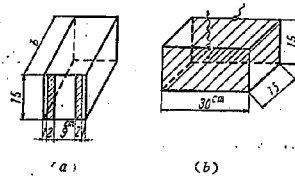
図-5 コンクリートの見掛けの比抵抗測定用供試体
