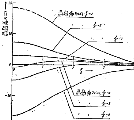
図-11 縁材の軸力 P_2(x) , P_3(x) の分布
