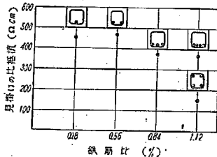
図-3 鉄筋量と見掛けの比抵抗との関係
