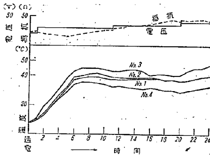
図-14 V 型の温度および電気的経過
