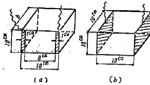
図-4 モルタルの見掛けの比抵抗測定用供試体
