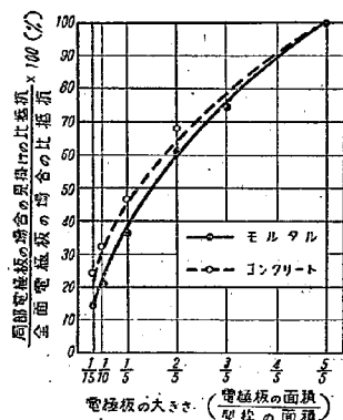
図-1 電極板の大きさと見掛けの比抵抗との関係
