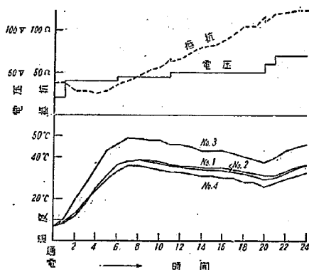
図-10 I 型の温度および電気的経過
