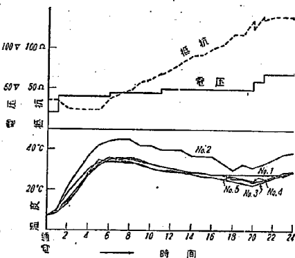
図-11 II 型の温度および電気的経過
