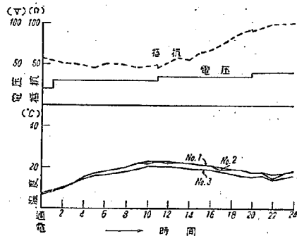
図-17 VIII 型の温度および電気的経過
