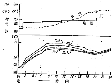
図-13 IV 型の温度および電気的経過
