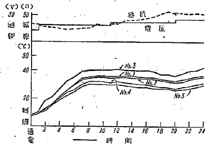
図-15 VI 型の温度および電気的経過
