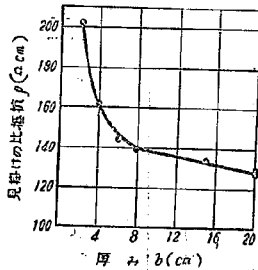
図-6 厚みの変化によるモルタルの見掛けの比抵抗
