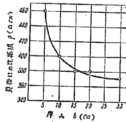
図-7 厚みの変化によるコンクリート見掛けの比抵抗
