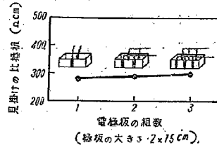
図-2 電極板の組数と見掛けの比抵抗との関係
