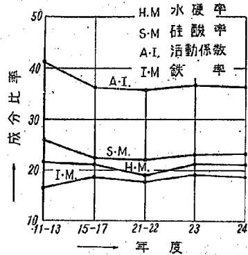
図—4 年度別セメント成分比率
