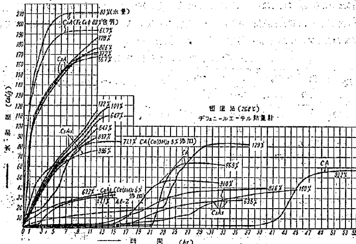
図-4 C_3A_{11} \cdot 11H_2O 系: 水和熱-時間 (恒温浴 26.8°C)
