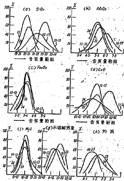
図-3 年度別ポルトランドセメント主成分の含有量および程度
