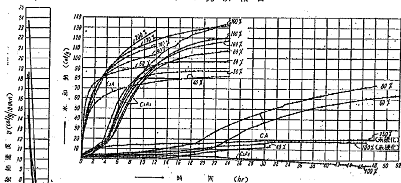
圖—10 C_mA-H_2O 系：水和熱—時間 (恒溫法) 0^{\circ}C
