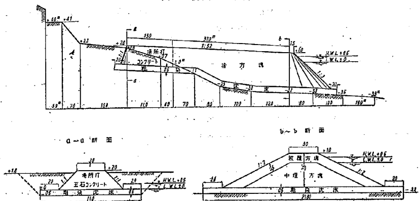
圖-4 防砂堤 C 設計圖
