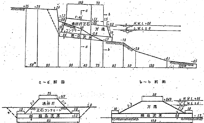
図-6 防砂堤・J 設計図
