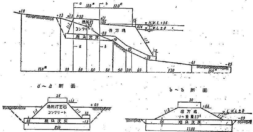
図-5 防砂堤・D 設計図
