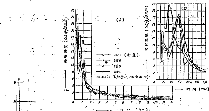
図-5(A~B) C_3A-H_2O 系: 発熱速度-時間, 恒温法 (26.8°C)
