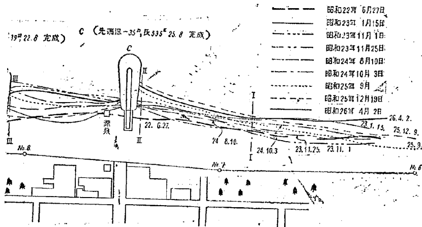
図一 鳥取県皆生海岸に於ける防砂突堤と汀線の変化
