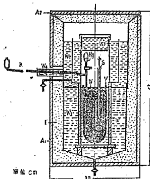
図一 水熱量計
