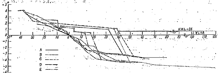
図-12 各防砂堤 A, B, C, D, E の縦断の比較
