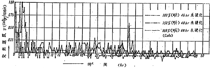
図—14 C_3A-H_2O 系: 発熱速度—時間 0^\circ C (恒温法) 48hr
