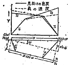
図-12 傾斜層の走時曲線
