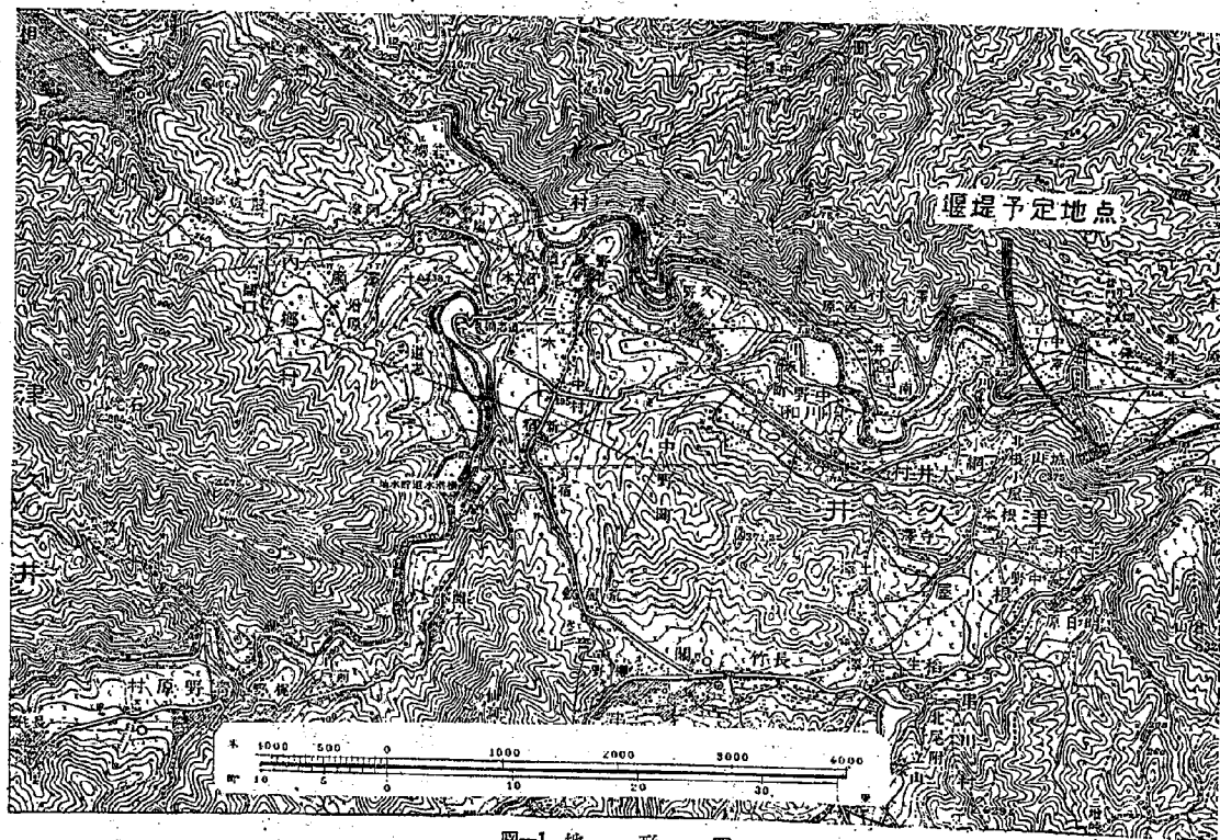
圖-1 地形圖
