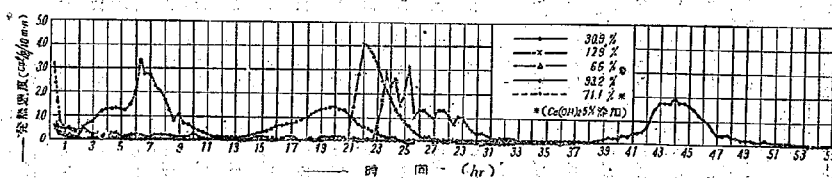
図-7 OA-H_2O 系: 発熱速度-時間 恒温法 (26.8°C)
