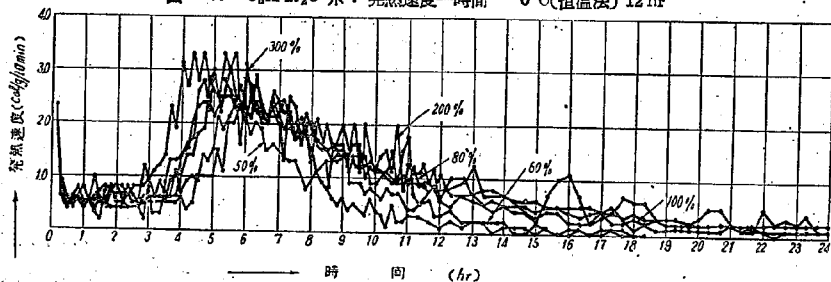
圖—12 C_6A-H_2O 系：發熱速度—時間 0^{\circ}C (恒溫法) 24hr
