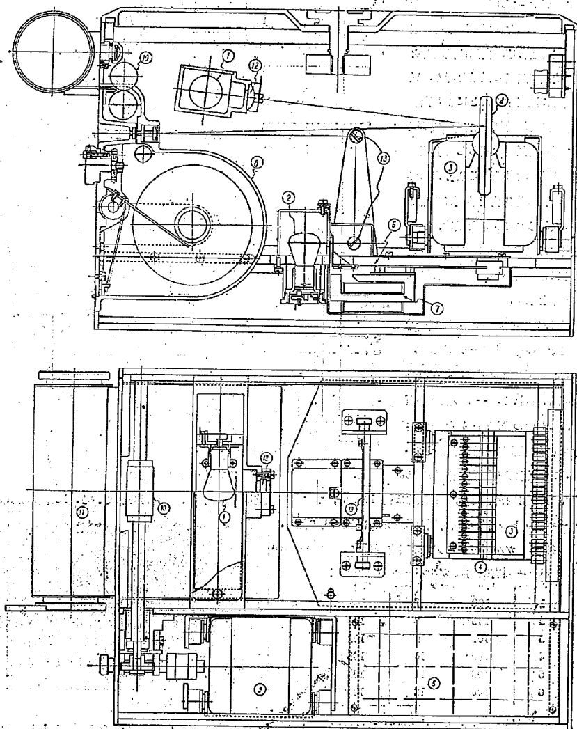
圖—9 記錄器断面圖
