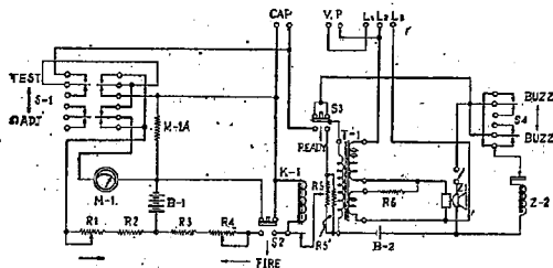
図-10 爆破器の結線図
