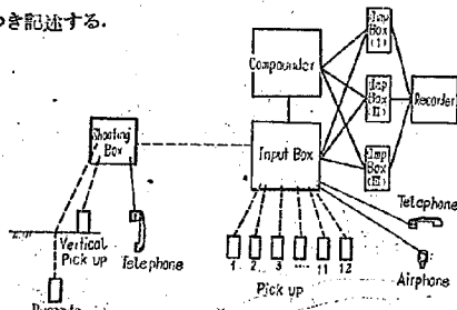
図-3 系 統 図
