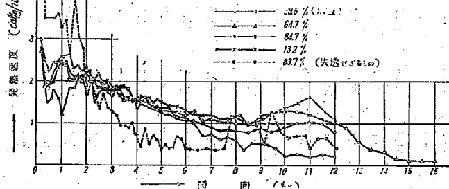
図-6 C_5A_3-H_2O 系: 発熱速度-時間 恒温法 (26.8°C)
