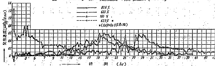
図-8 C_3A_5-H_2O 系: 発熱速度-時間, 恒温法 (26.8°C)
