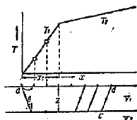
図-11 水平二層の走時曲線
