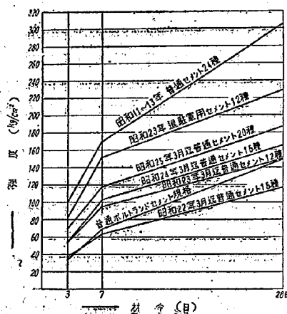
図-6 圧縮強度
