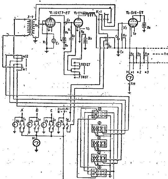
図-8 増幅制禦器の結線図
