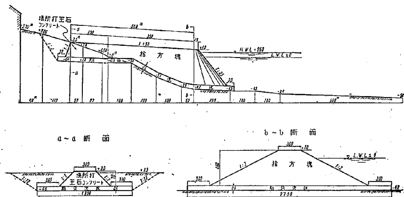
圖-3 防砂堤 B 設計圖
