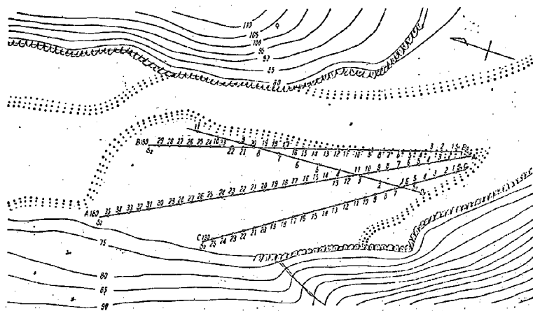
図-2 堰堤附近拡大図並びに測定線図
