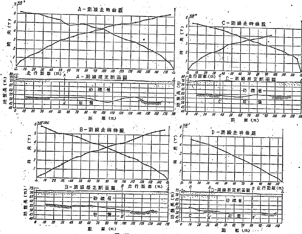
圖-13 走時曲線
