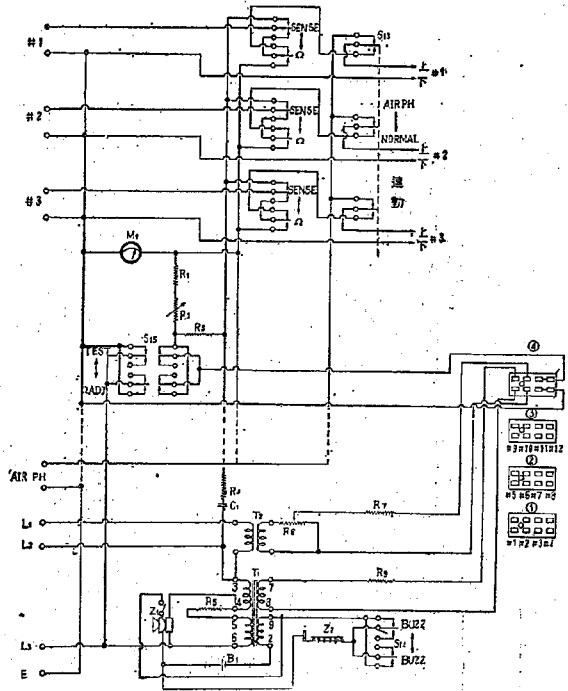
図-8 入力試験器の結線図
