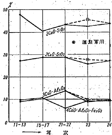
図-2 年度別ポルトランドセメントの水溶性成分 (Bogue 法により算出)
