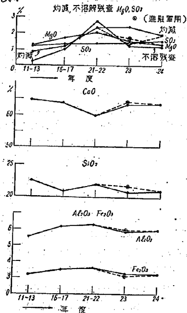
図-1 年度別ポルトランドセメントの化学成分
