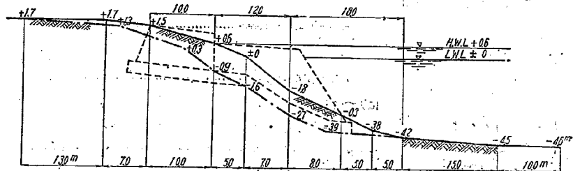
図—15 防砂堤 D に於ける海岸の縦断形状、鎖線は昭和25年6月頃、実線は昭和26年5月頃のもの。
