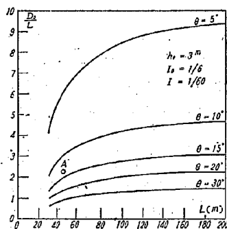
図-19 点 A は皆生海岸の防砂堤 A を示す。
