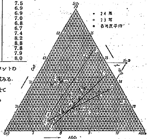
図-5 本邦セメントの \text{CaO}-\text{SiO}_2-\text{Al}_2\text{O}_3 三元組成図
