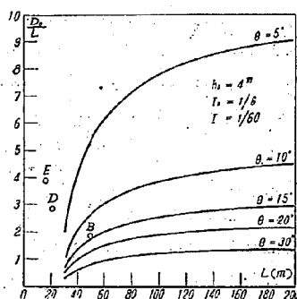
図-20 点 B, D, E は皆生海岸の防砂堤 B, D, E を示す。
