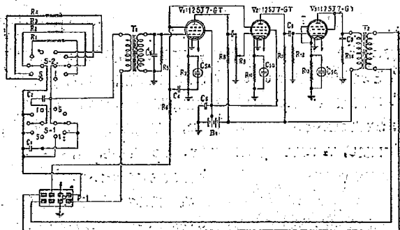
図—5 増幅器の結線図
