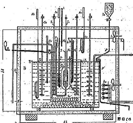
圖—3 Diphenyl-ether 熱量計装置(配管図)
