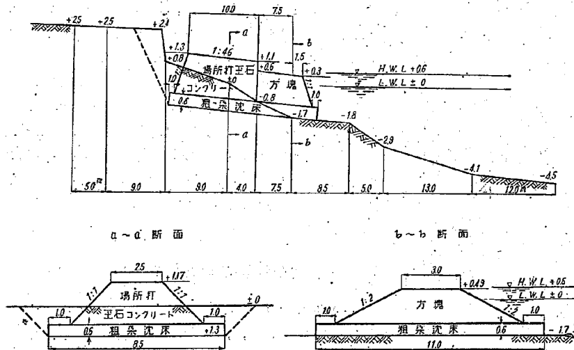
圖一-6 防砂堤 E 設計圖
