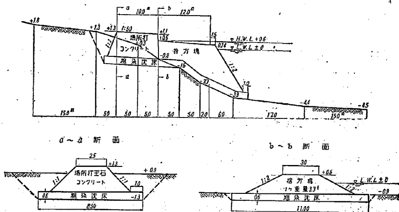
圖一5 防砂堤・D 設計圖
