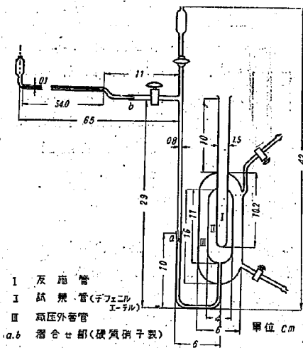
図-1 熱量計の寸法
