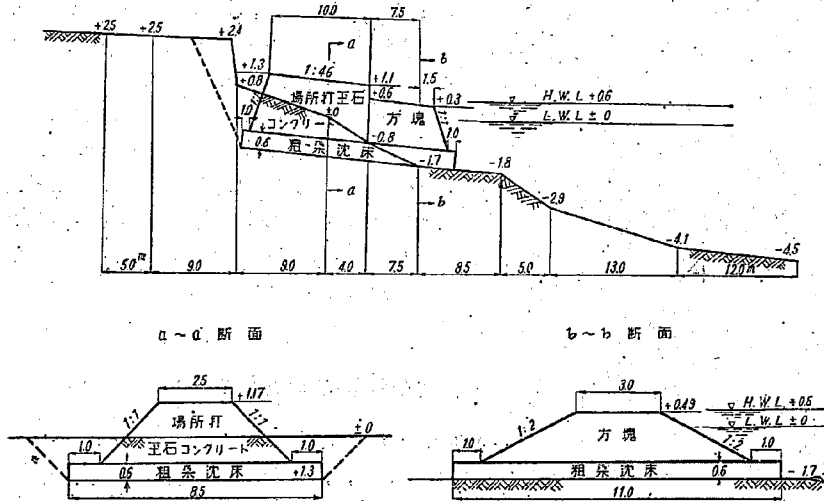
図-6 防砂堤・J 設計図
