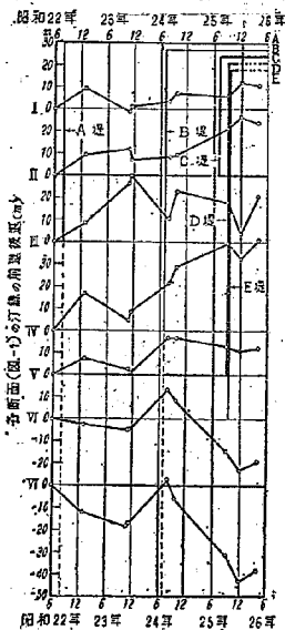
図-7 皆生海岸の汀線の出入り(昭和22年6月から昭和26年6月まで)
