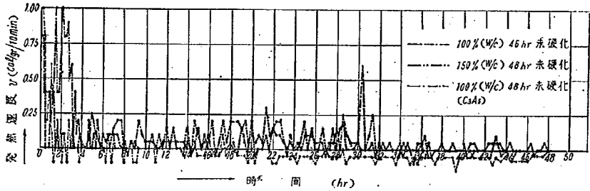
図—14 C_3A-H_2O 系: 発熱速度—時間 0^\circ C (恒温法) 48hr
