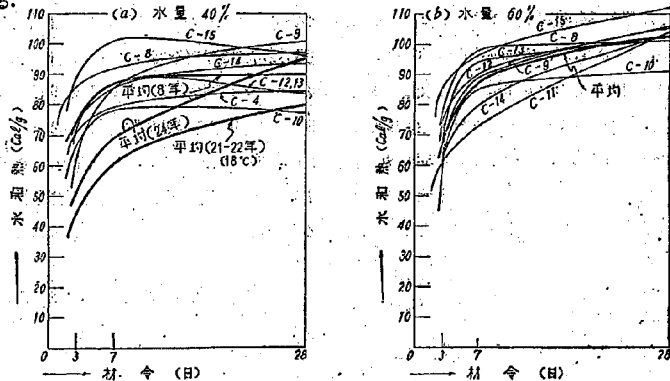
図-7 セメントの水和熱—材令 ( 38^{\circ}\text{C} )
