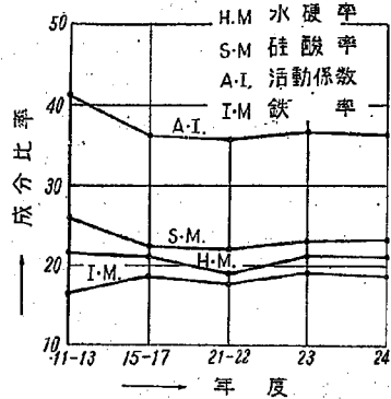
図—4 年度別セメント成分比率
