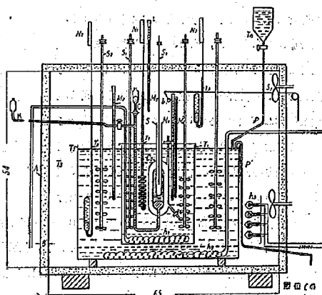
図—3 Diphenyl-ether 熱量計装置(配管図)
