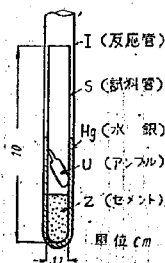
図—2 試料投入図
