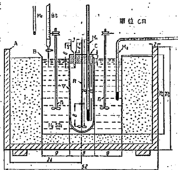
図-1 熱量計
