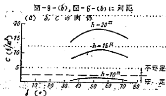
図-11 受効土圧破壊の計算結果
