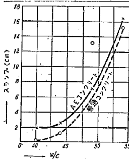
図-10 AEコンクリートと普通コンクリートのスランプ
