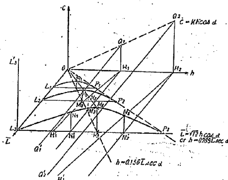
図-4 地り最大深さと地表面長さ粘着力間関係
