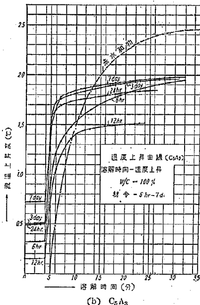
図-4 C_m A_n 溶解液温度上昇曲線
