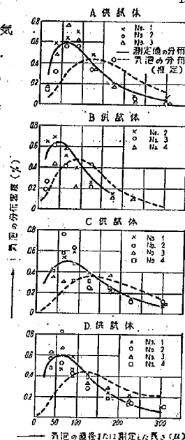
図-6 気泡の分布
