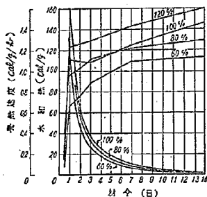
図-7 CA-H 2 O 系の水和熱及発熱速度 一時的に停滞する時期がある。
