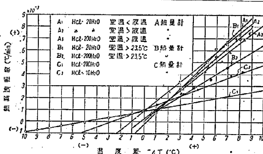
図—2 熱漏減恒数測定例
