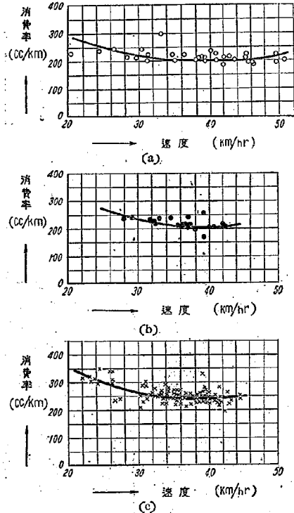
図-5 速度とガソリン消費率の関係
