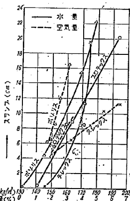
図-7 スランプと空気量又は水量との関係
