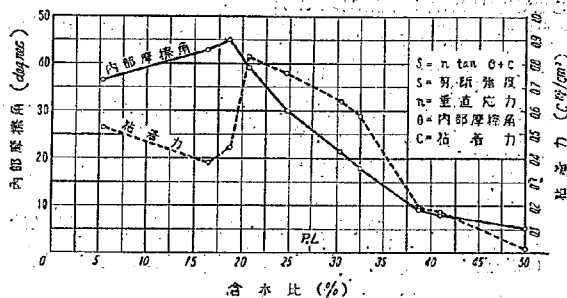
図-17 含水比と剪断強度との関係
