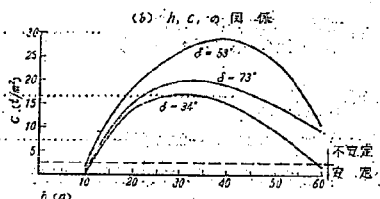
図-11 受効土圧破壊の計算結果
