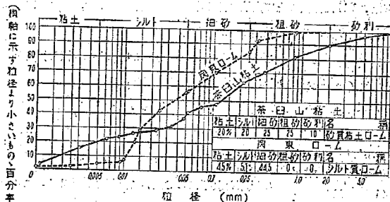
図-16 横型実験用土の粒径加積曲線
