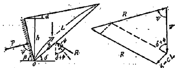
図-8 受仕土圧による破壊
