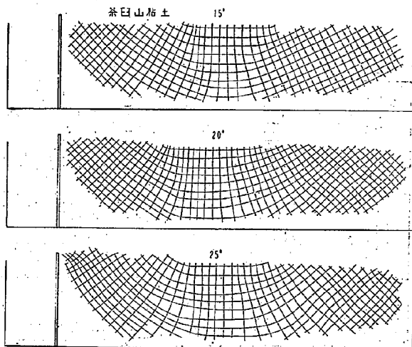
図-25 主歪方向線図
