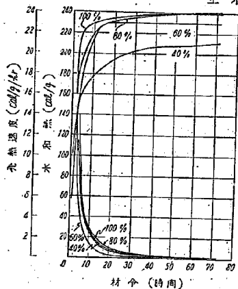
図-5 C_3A-H_2O 系の水和熱および発熱速度
