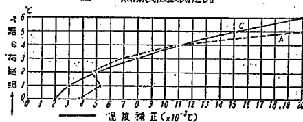
図—3 Beckmann 温度計目盛補正図
