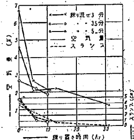
図-5 練り置き時間と空気量との関係
