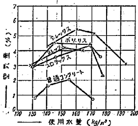
図—4 使用水量と空気量との関係
