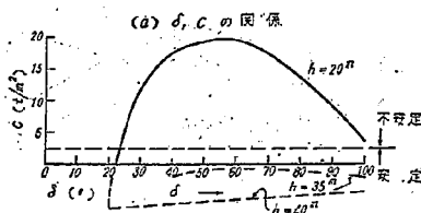
図-10 受効土圧破壊の計算結果
