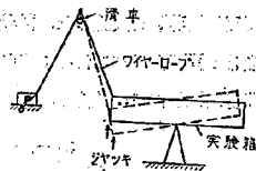
図—18 実験方法
