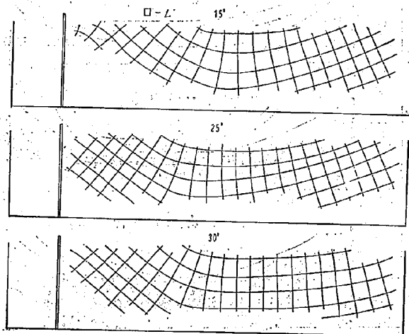
図-25 主歪方向線図
