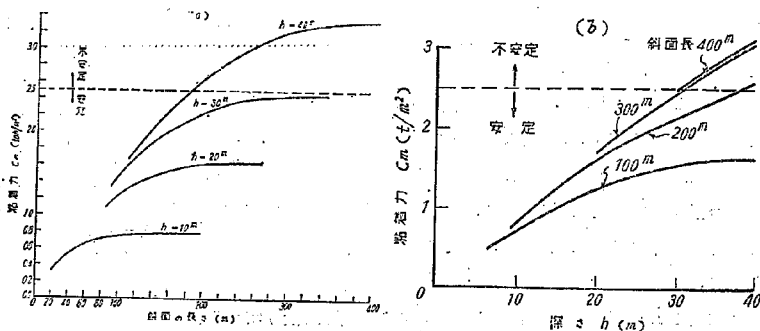
図-5 摩擦円法による斜面安定計算結果
