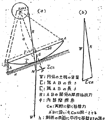
図一 円形這り面
