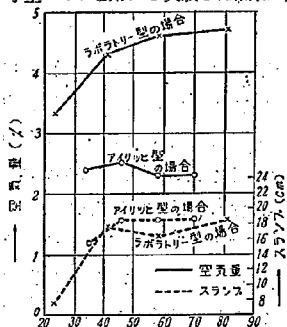
ミキサの公称容量に対するパッチの量(%) 図—3 練り混ぜ量と空気量スランプとの関係
