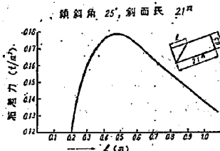
図-23 茶臼山粘土を用いた地中り面観測において受効土圧破壊を仮定して計算した結果
