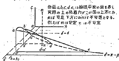
図-9 受仕土圧破壊に於ける c , \delta , h 間の関係
