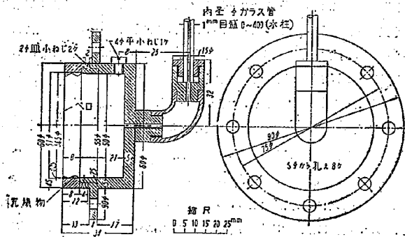
図-15 土 圧 計
