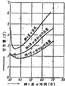
図—2 練り混ぜ時間と空気量との関係
