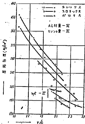
図-9 V/C と強度との関係
