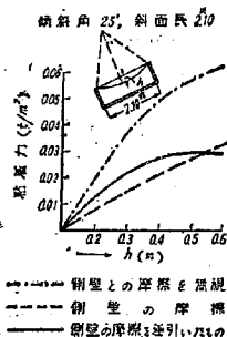
図-22 茶臼山粘土を用いた地中り面観測において円形滑り面説で計算した結果
