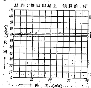
図-26 土圧計測定結果
