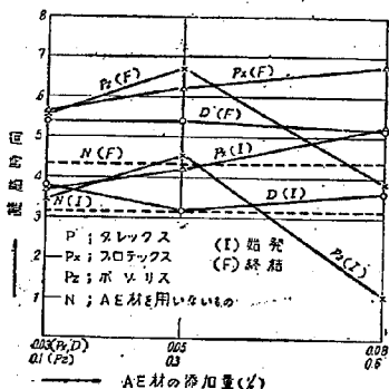
図-8 A E 材の添加が凝結に及ぼす影響
