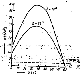
図-13 壁面と土との滑りに對する安定度 壁面の水平に對する傾角 \beta (°) と粘着力 c (kg/cm²) の関係
