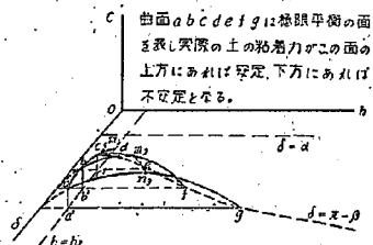
図-9 受仕土圧破壊に於ける c , \delta , h 間の関係
