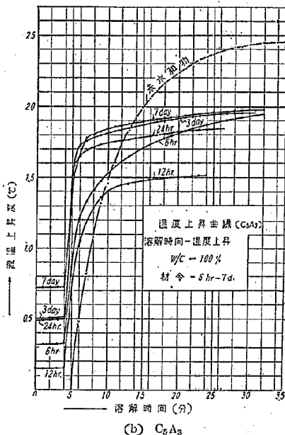
図-4 C_mA_n 溶解液温度上昇曲線
