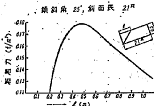
図-23 茶臼山粘土を用いた地中り面観測において受働土圧破壊を仮定して計算した結果
