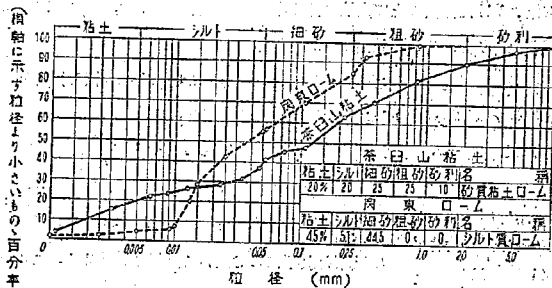
図-16 模型実験用土の粒径加積曲線
