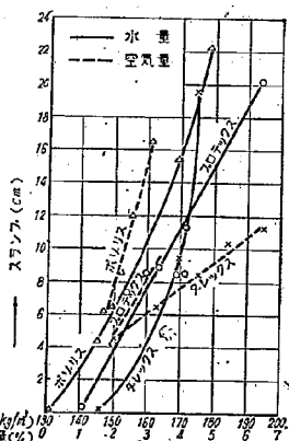
図-7 スランプと空気量又は水量との関係
