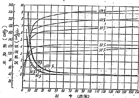
図-6 C_5A_3-H_2O 系の水和熱及発熱速度
