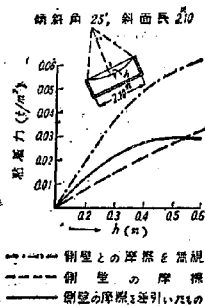
図-22 茶臼山粘土を用いた地中り面観測に於いて円形滑り面説で計算した結果
