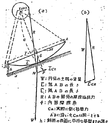
図-1 円形這り面
