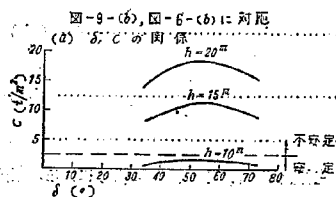
図-11 受効土圧破壊の計算結果
