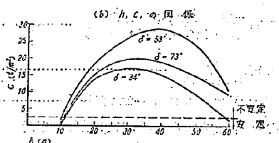
図-11 受効土圧破壊の計算結果
