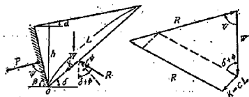
図-8 受仕土圧による破壊
