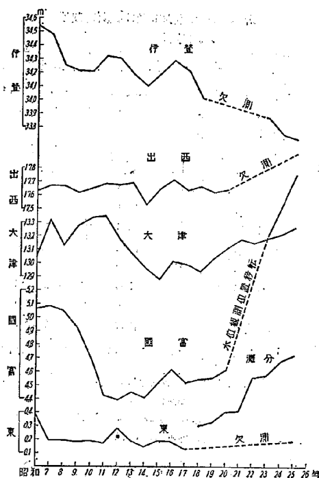
図-6 伊勢川水系量水標年平均低水位変化図
