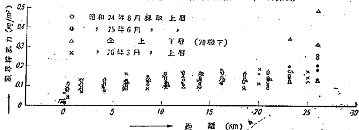
圖—14 限界掃流力変化圖
