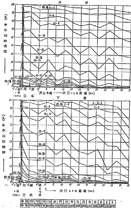
圖—13 斐伊川底質距離通過百分率圖(昭和25年6月採取)
