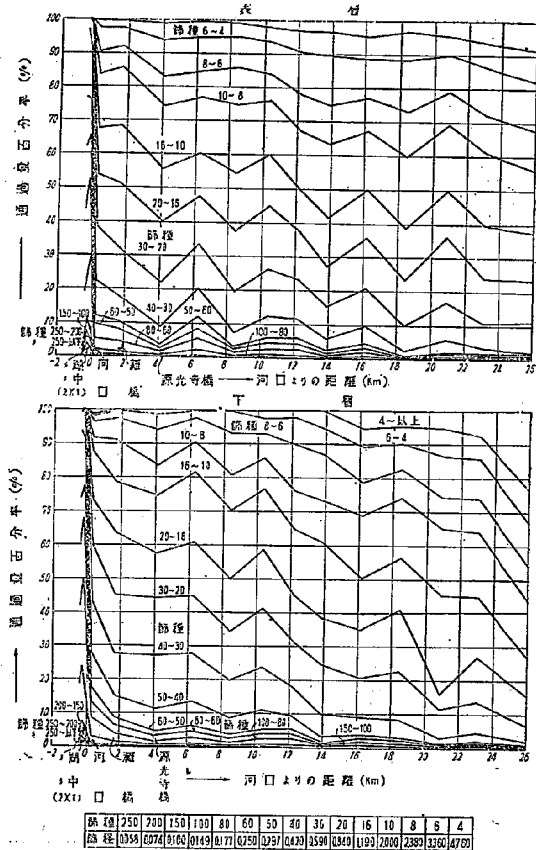
図一13 斐伊川底質距離毎通過百分率図(昭和25年6月採取)
