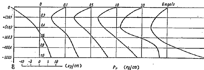
図—13 p_r (kg/cm)
