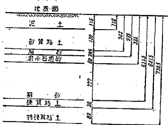
その下 5.20m 位までは貫入抵抗 0.01068~0.00117cm で 中位地層と硬質地層との混合地層なる事が推定され、その 下 5.972m までは貫入抵抗 0.00117~0.000087cm で硬質 地層の上部なる事が推定される。貫入深さ 5.972m の時上 部枕と下部枕との継手ボルトが下側に於て全部切断し、継 手面コンクリートが圧挫して、これ以上枕を打込む事が出 来なくなつたので、打込試験を中止し、この試験枕より約 2.5m 離れた位置にてボーリングを行つて地盤の現実調査 を行つた。
