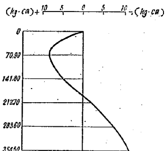
図—19 p_r(\text{kg/cm})
