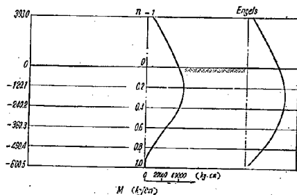
図-15 M (kg/cm)
