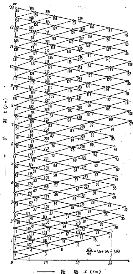
図-2 特性曲線群
