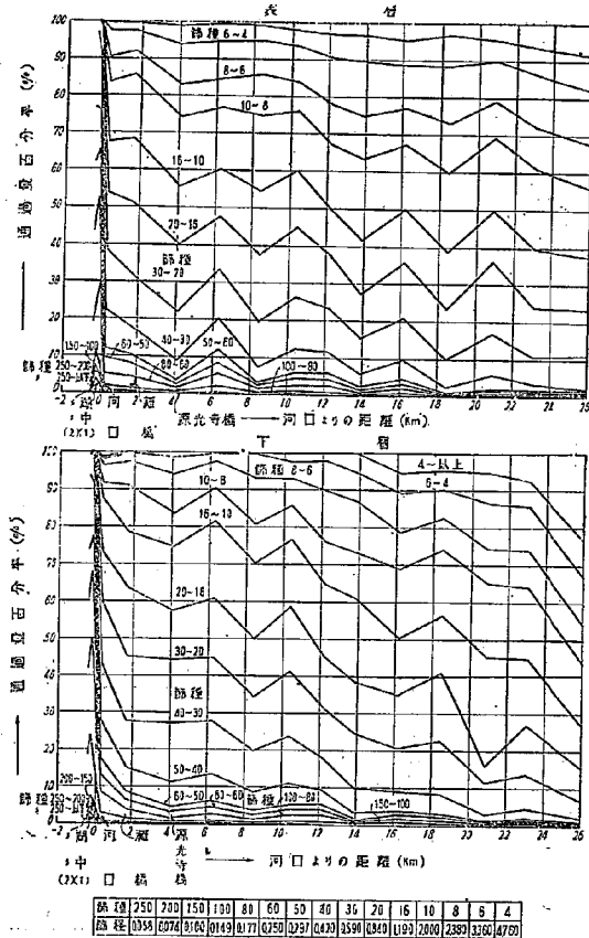
図—13 斐伊川底質距離毎通過百分率図(昭和25年6月採取)
