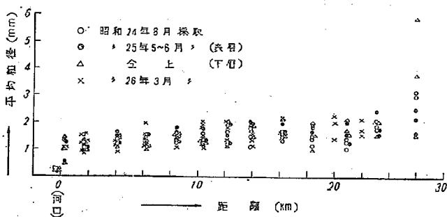
図-12 河床材料平均粒径変化図
