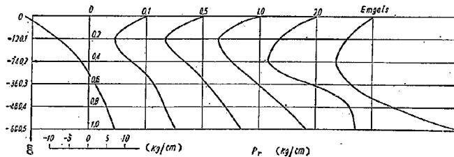
図—13 p_r (kg/cm)
