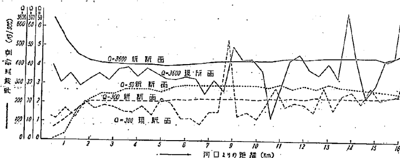
図-15 浮游流砂量距離的变化図
