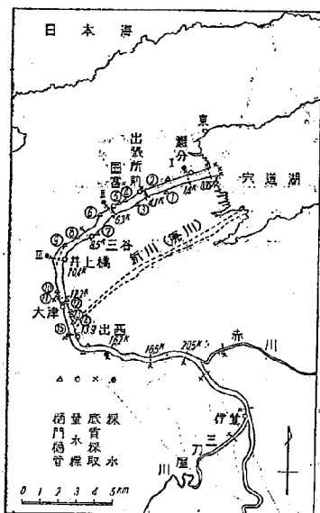
図-5. 灌溉一般図
