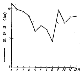
図-11 月別浮游流砂量(澁分～国富)
