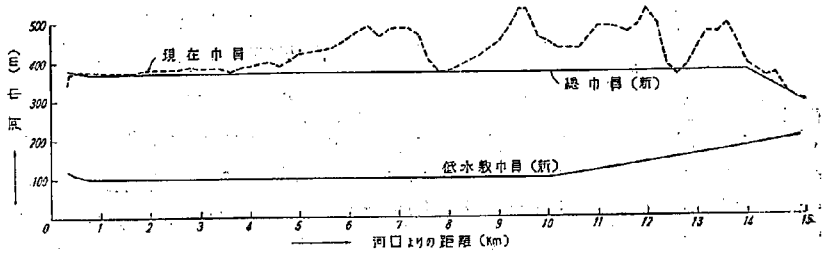
図-16 幅員変化図
